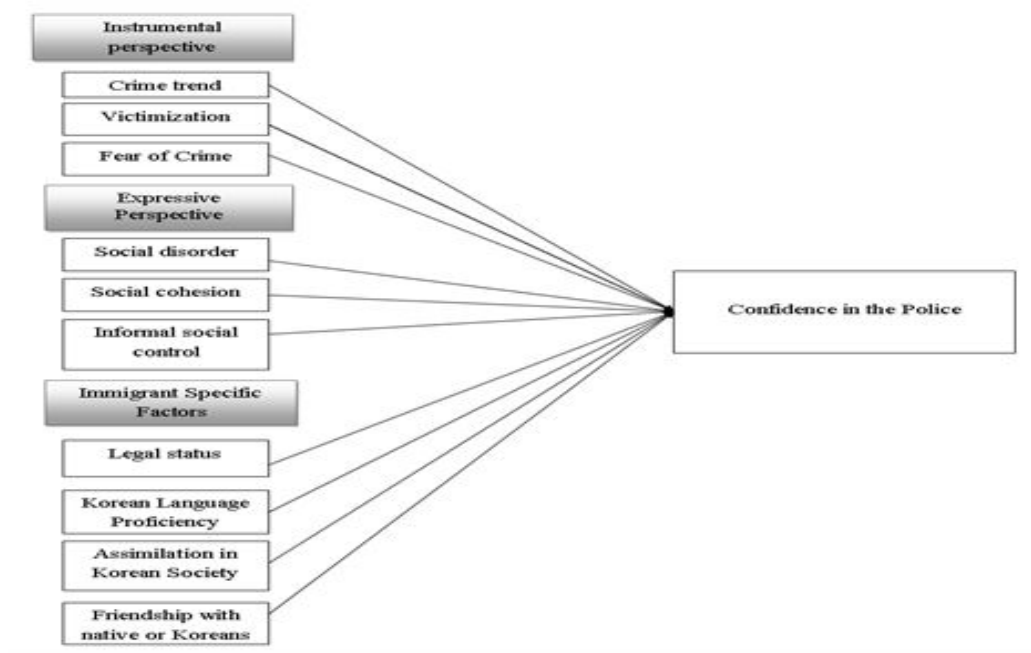
Загвар-1. Монголчуудын цагдаад итгэх хандлагыг шалгах загвар
