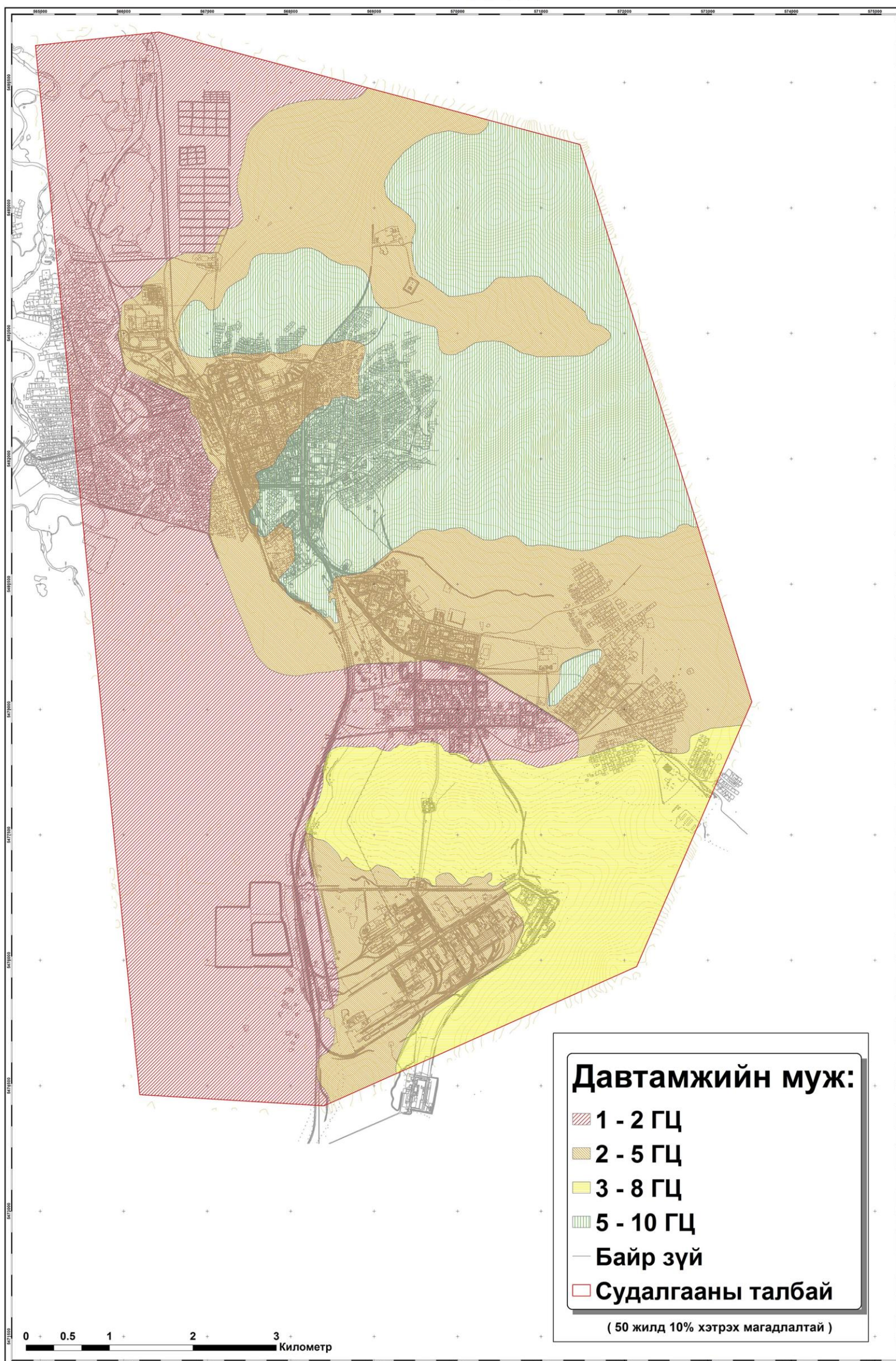
Зураг 45 Дархан- Уул аймгийн төв Дархан сумын хөрсний зонхилох давтамжийн мужлал
