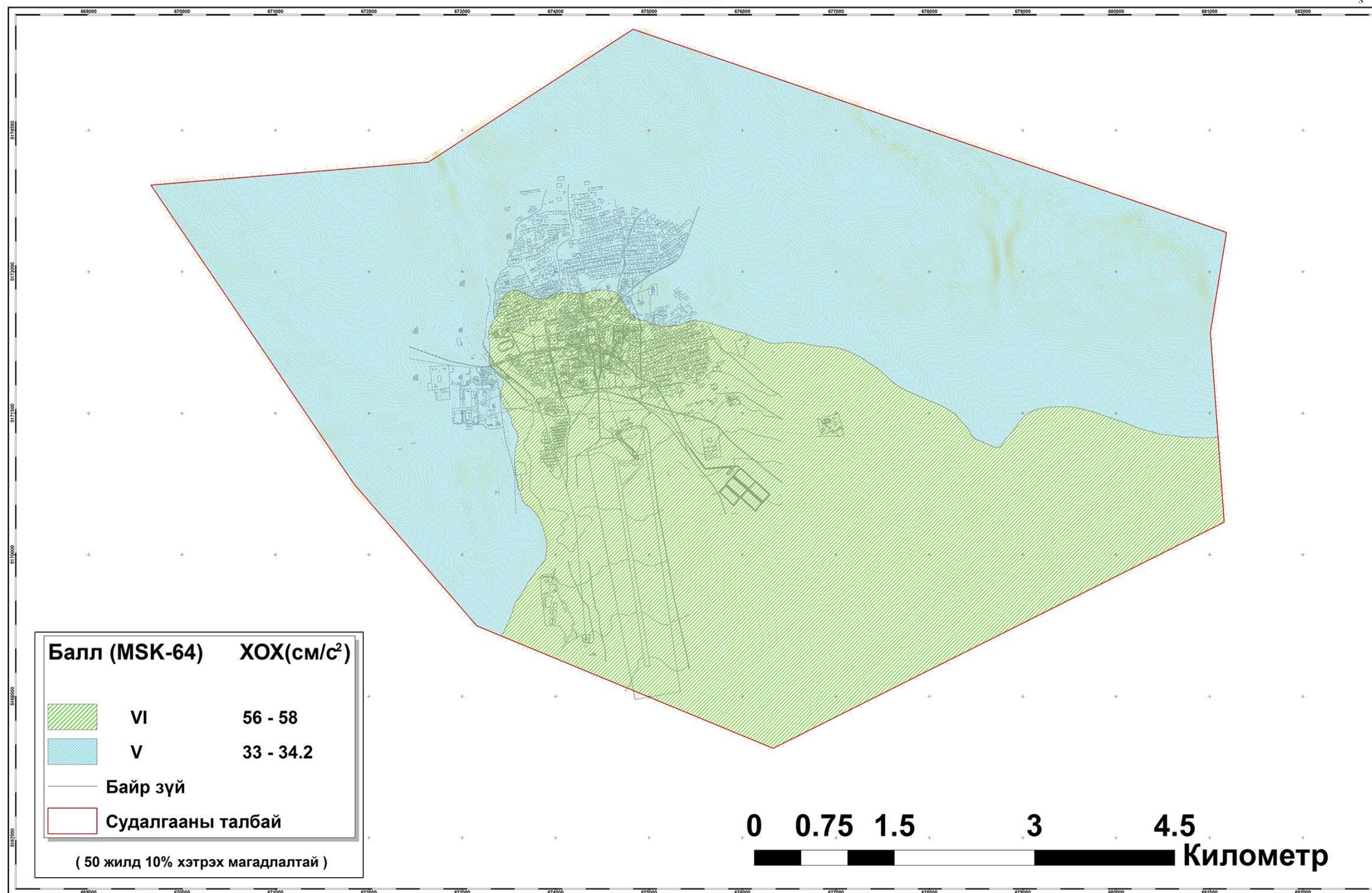
Зураг 112 Сүхбаатар аймгийн төв Баруун- урт сумын газар хөдлөлийн бичил мужлалын зураг (500 - жил )
