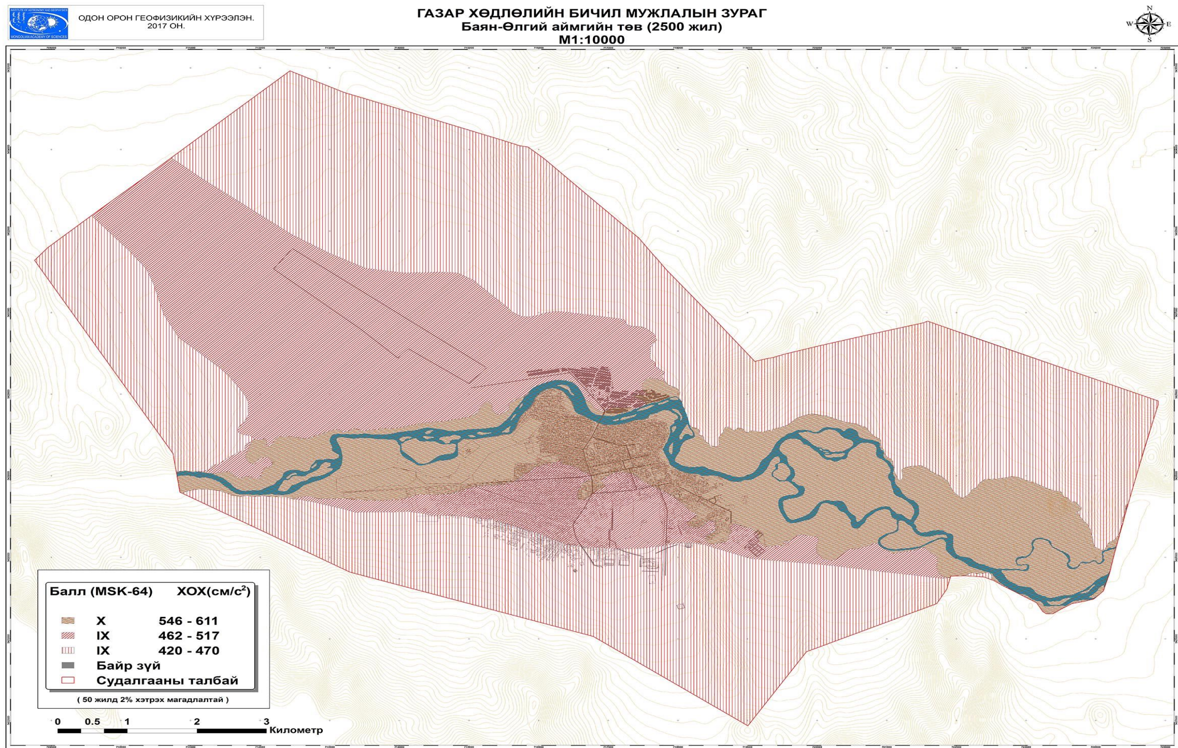
Зураг 36 Баян- өлгий аймгийн төв Өлгий сумын газар хөдлөлийн бичил мужлал (2500- жил )
