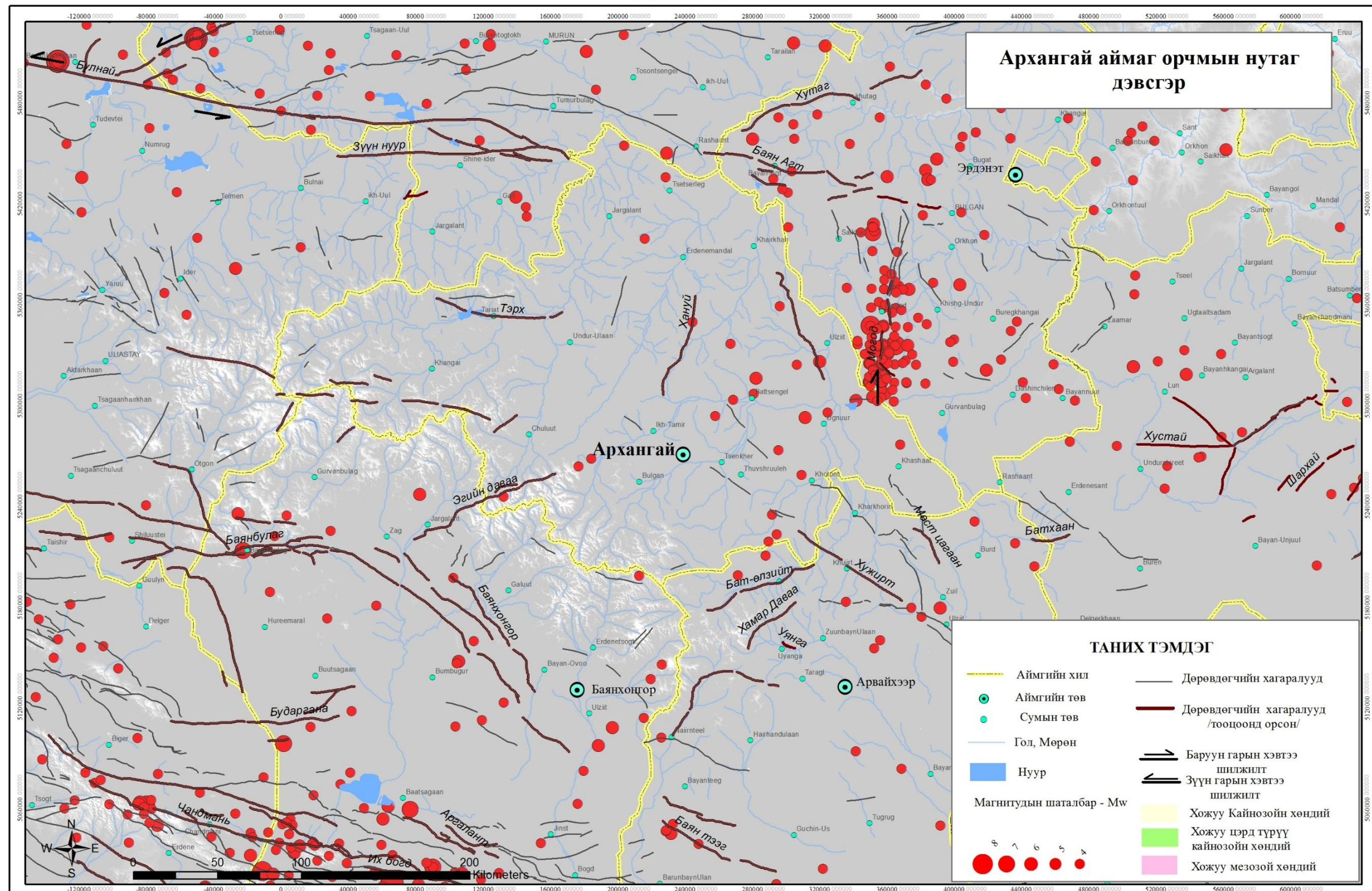
Зураг 7 Архангай аймаг орчмын сейсмотектоникийн тойм зураг
