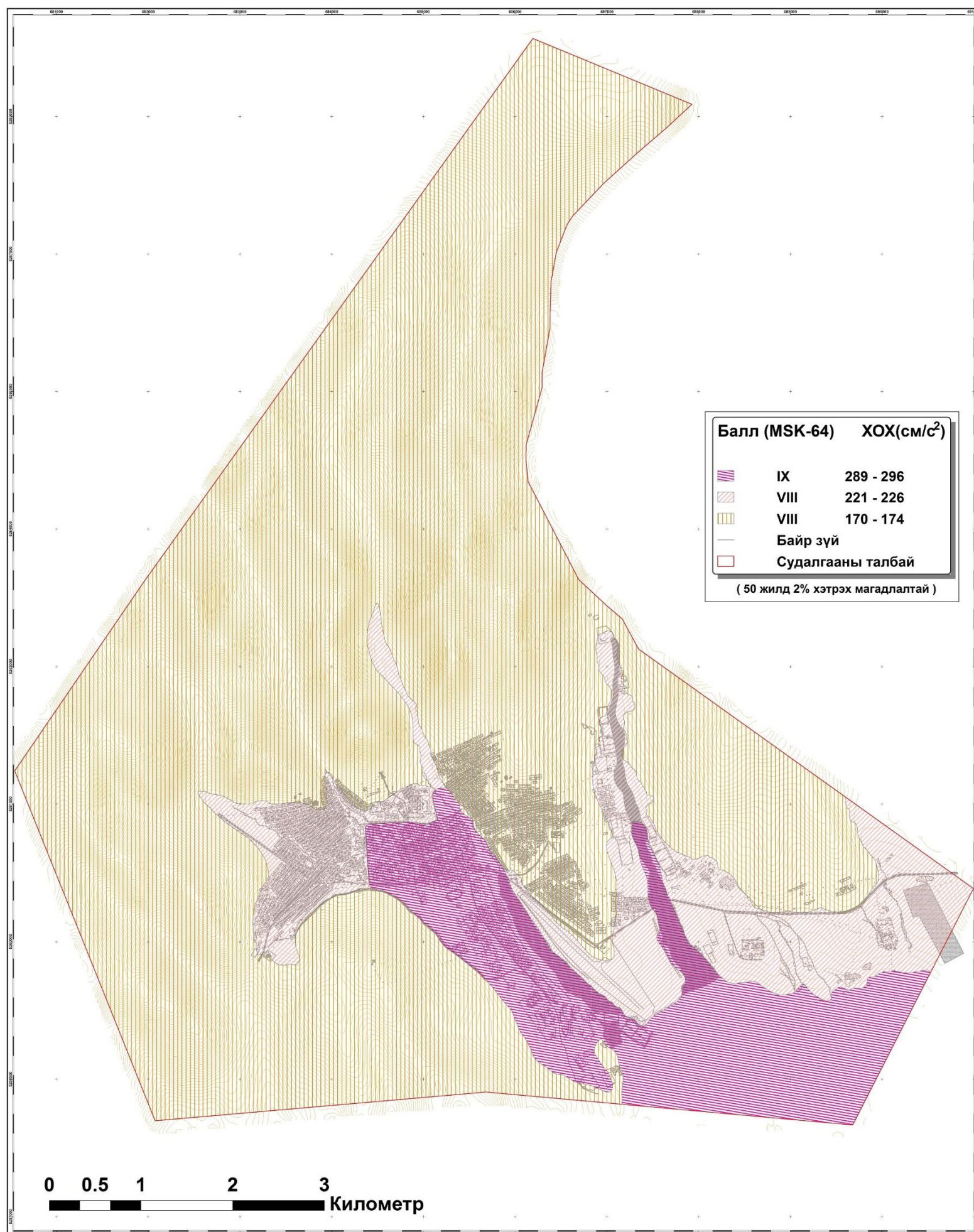
Зураг 14 Архангай аймгийн төв Эрдэнэбулган сумын газар хөдлөлийн мужлал. (2500 жил)
