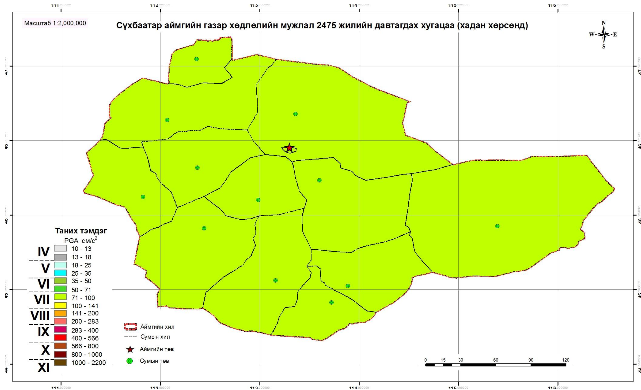
Зураг 109 Сүхбаатар аймгийн төв Баруун- урт сумын газар хөдлөлийн мужлал (2475 жилийн давтагдах хугацаа- хадан хөрсөнд)
