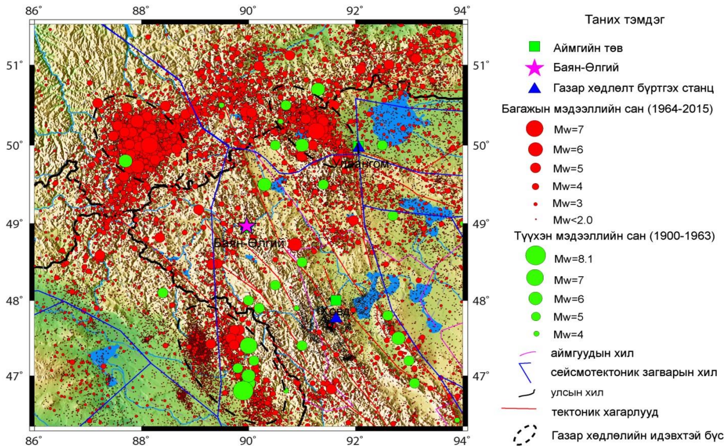
Зураг 30 Баян- өлгий аймаг орчмын сейсмоструктурн тойм зураг
