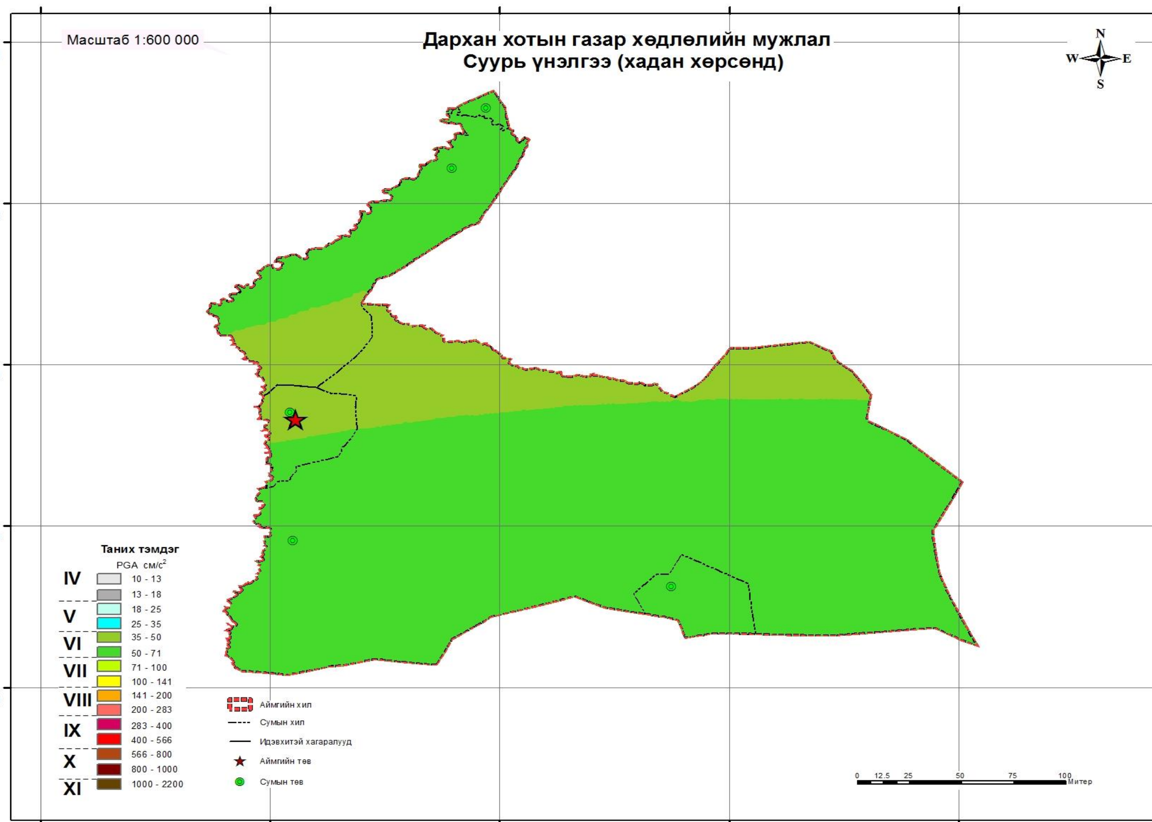
Зураг 44 Дархан- Уул аймгийн төв Дархан сумын газар хөдлөлийн мужлал –Суурь үнэлгээ ( хадан хөрсөнд)
