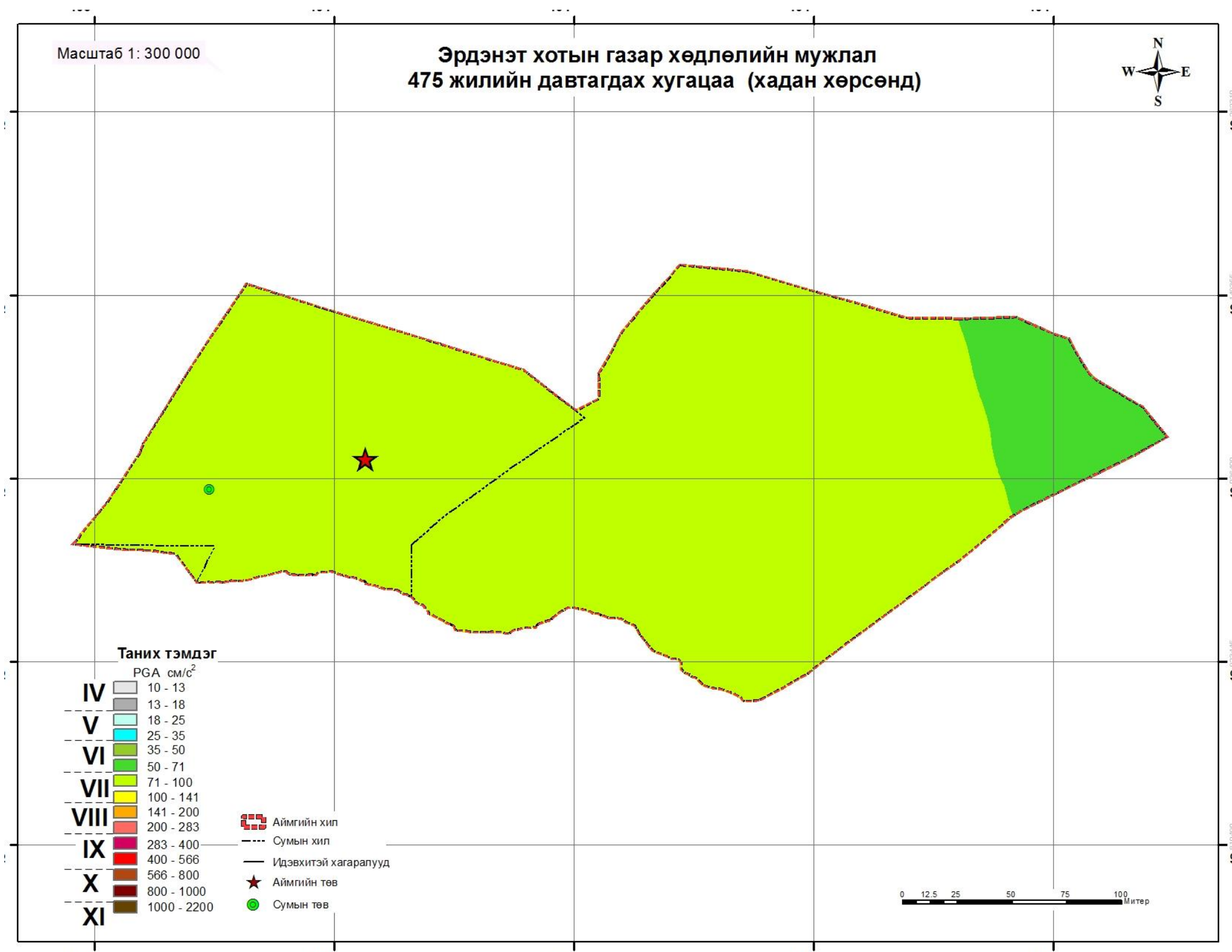
Зураг 86 Орхон аймгийн төв Баян- Өндөр сумын газар хөдлөлийн мужлал (475 жилийн давтагдах хугацаа- хадан хөрсөнд)
