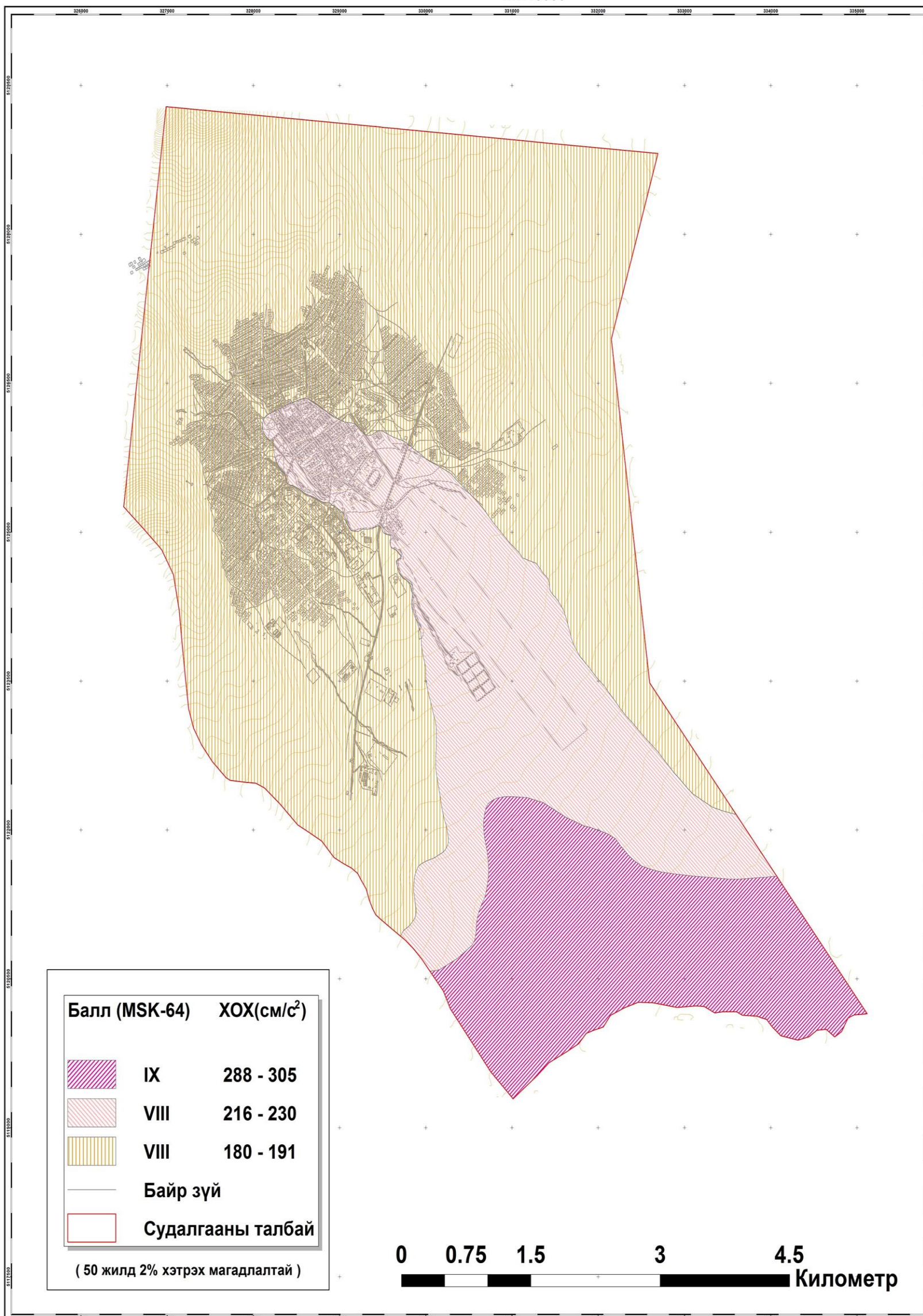
Зураг 124 Өвөрхангай аймгийн төв Арвайхээр сумын газар хөдлөлийн бичил мужлалын зураг (2500 жил )
