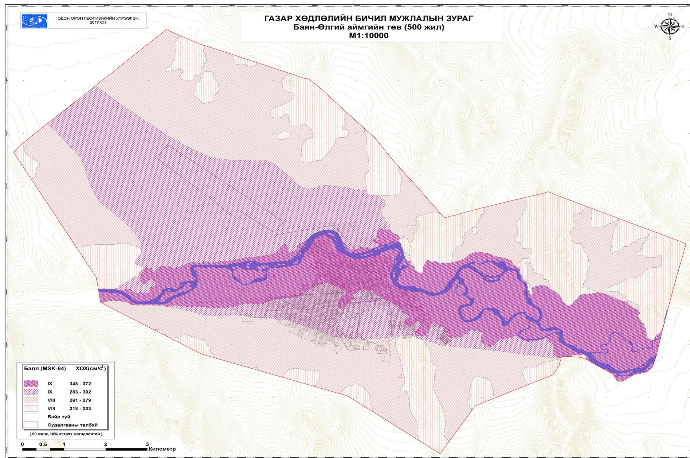
Зураг 35 Баян- өлгий аймгийн төв Өлгий сумын газар хөдлөлийн бичил мужлал (500- жил )
