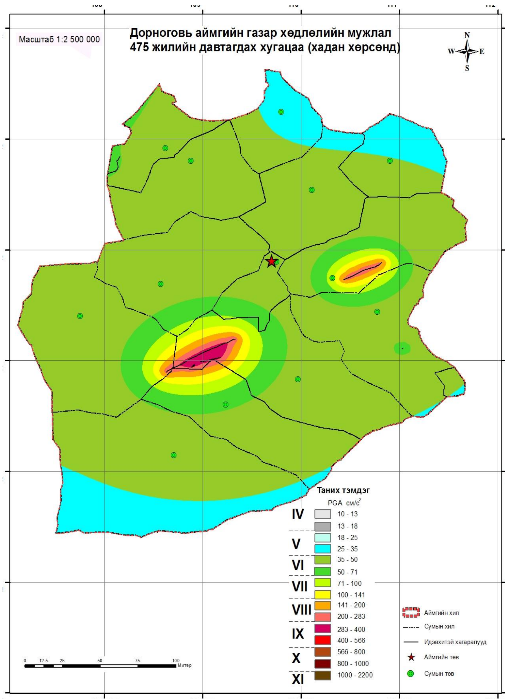
Зураг 53 Дорноговь аймгийн төв Сайншанд сумын газар хөдлөлийн мужлал (475 жилийн давтагдах хугацаа- хадан хөрсөнд)
