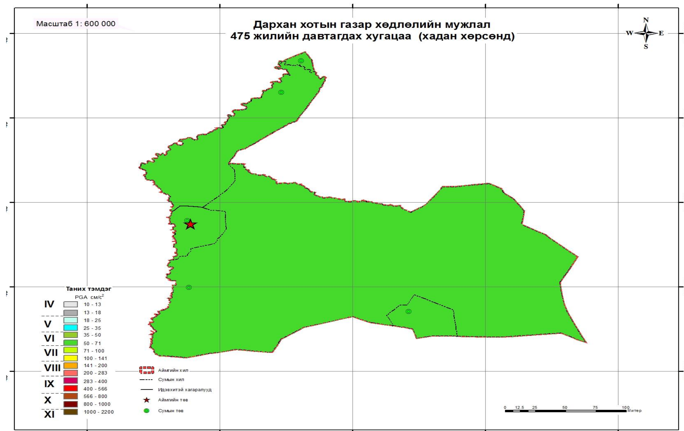
Зураг 42 Дархан- Уул аймгийн төв Дархан сумын газар хөдлөлийн мужлал (475 жилийн давтагдах хугацаа- хадан хөрсөнд)
