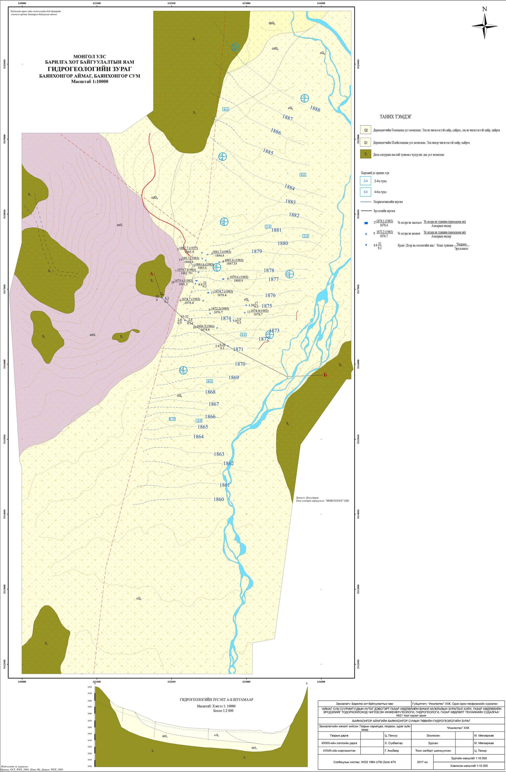
Зураг 17 Баянхонгор аймгийн Баянхонгор сумын гидро геологийн нөхцөлийн зураг.
