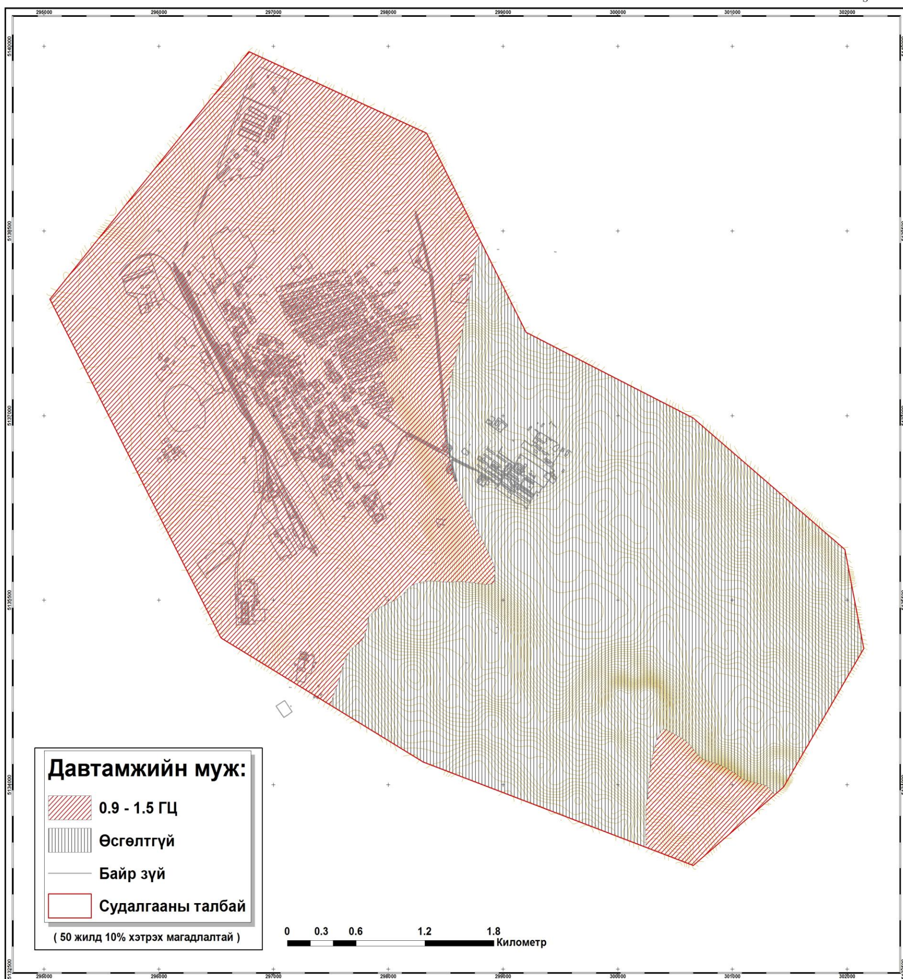
Зураг 78 Говьсүмбэр аймгийн төв Сүмбэр сумын хөрсний зонхилох давтамжийн мужлал.
