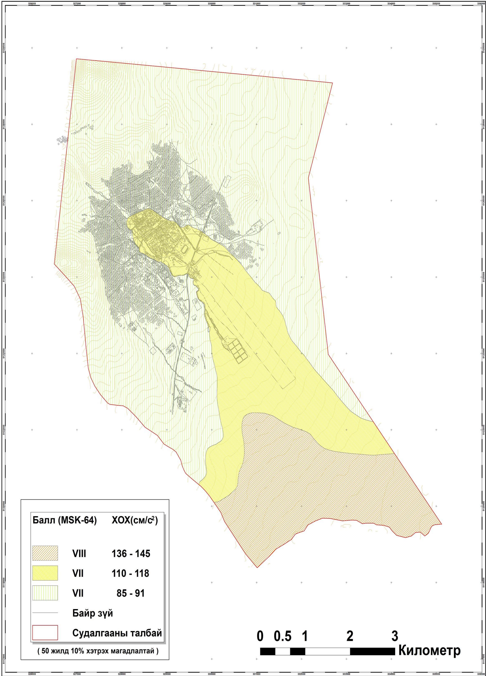
Зураг 123 Өвөрхангай аймгийн төв Арвайхээр сумын газар хөдлөлийн бичил мужлалын зураг (500 жил )
