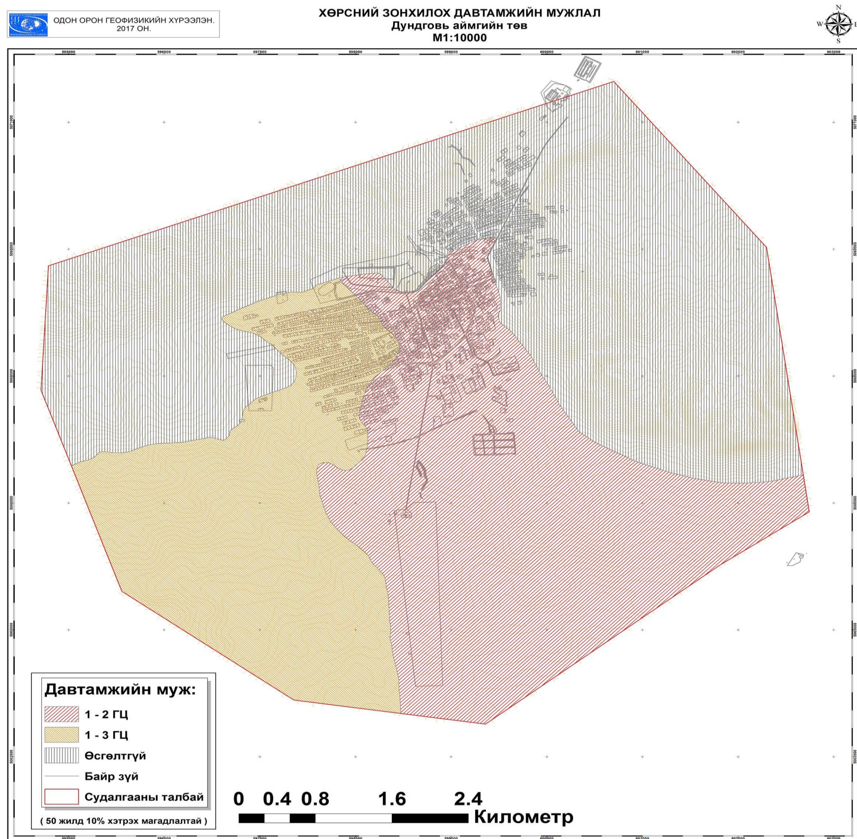
Зураг 67 Дундговь аймгийн төв Сайнцагаан сумын хөрсний зонхилох давтамжийн мужлал
