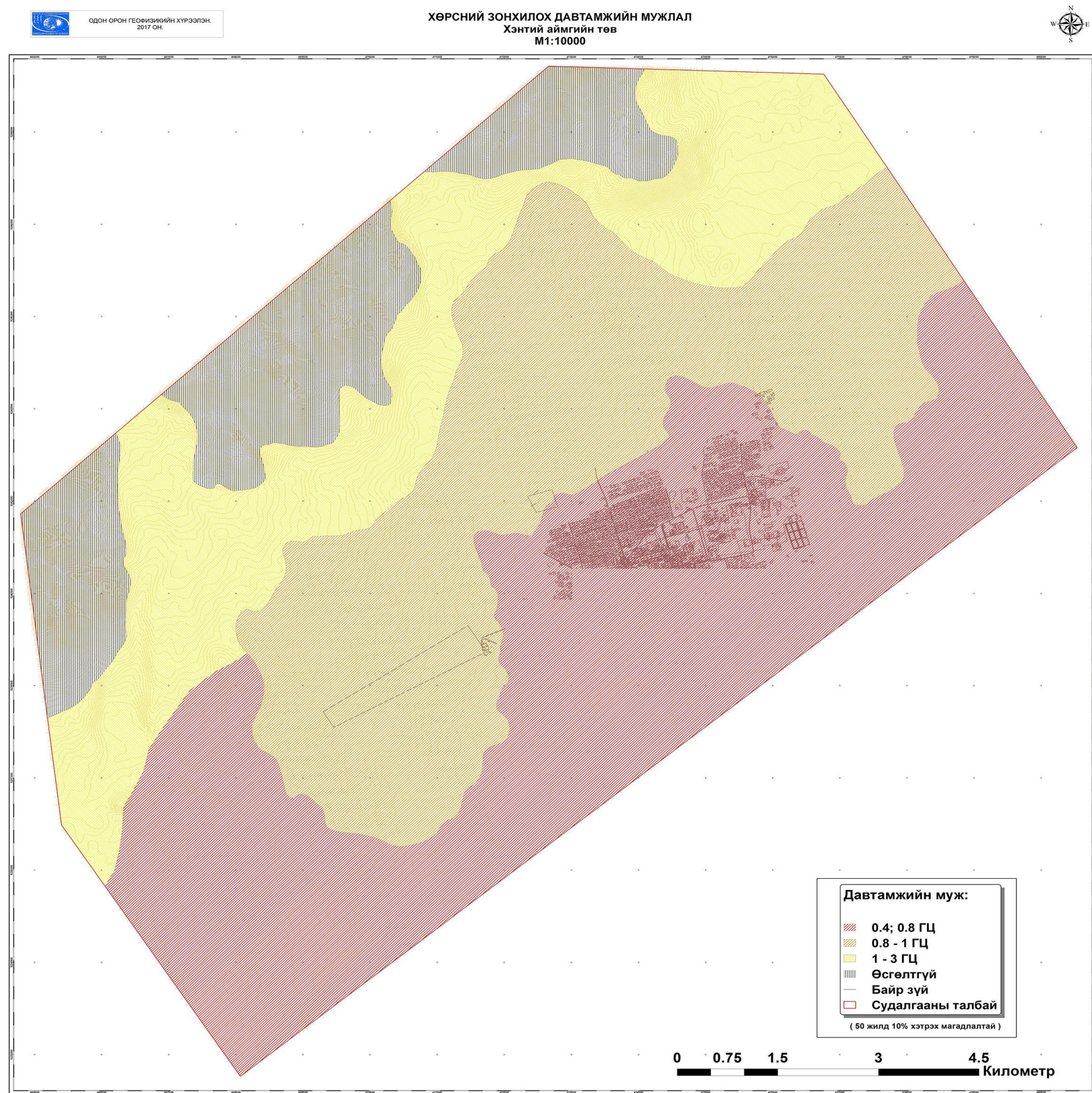
Зураг 100 Хэнтий аймгийн төв Хэрлэн сумын хөрсний зонхилох давтамжийн мужлал.
