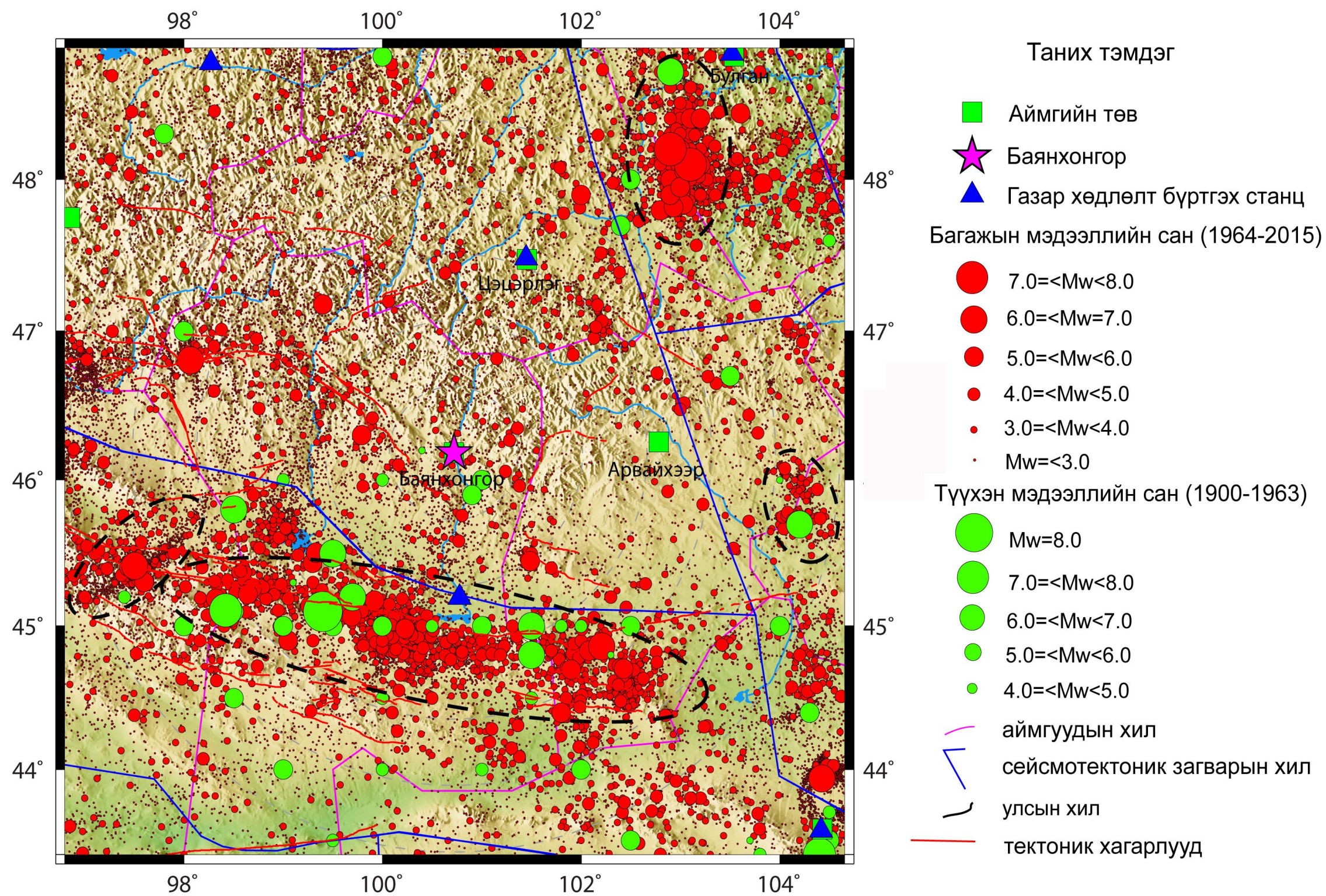
Зураг 19 Баянхонгор аймгийн Баянхонгор сумын газар хөдлөлийн идэвхжилт.
