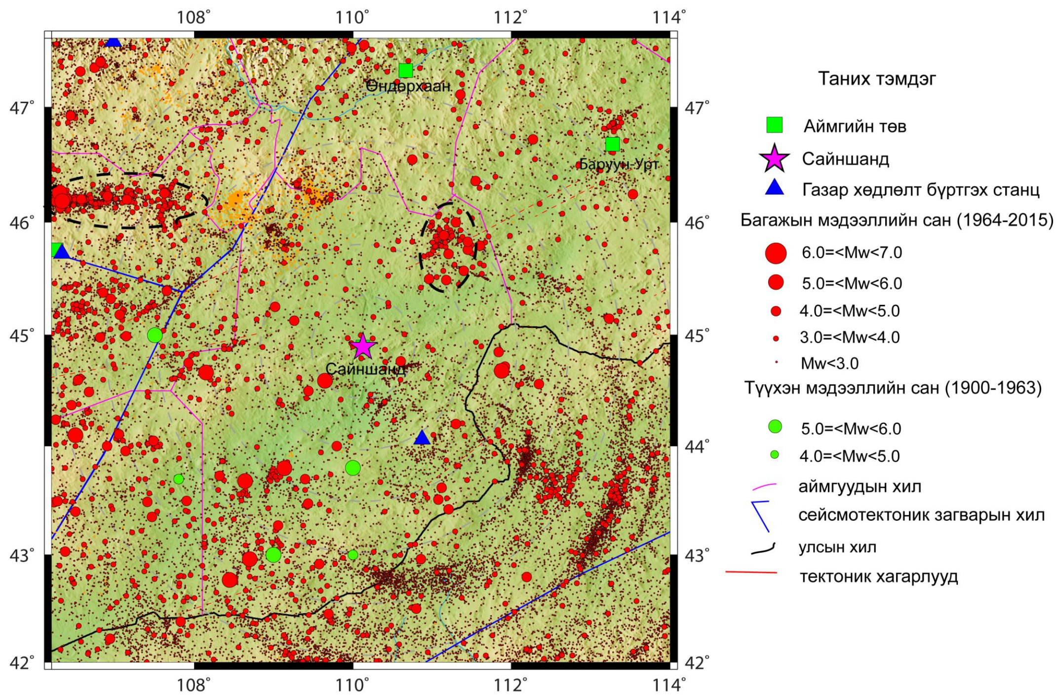
Зураг 52 Дорноговь аймгийн төв Сайншанд сумын газар хөдлөлийн идэвхжилт.
