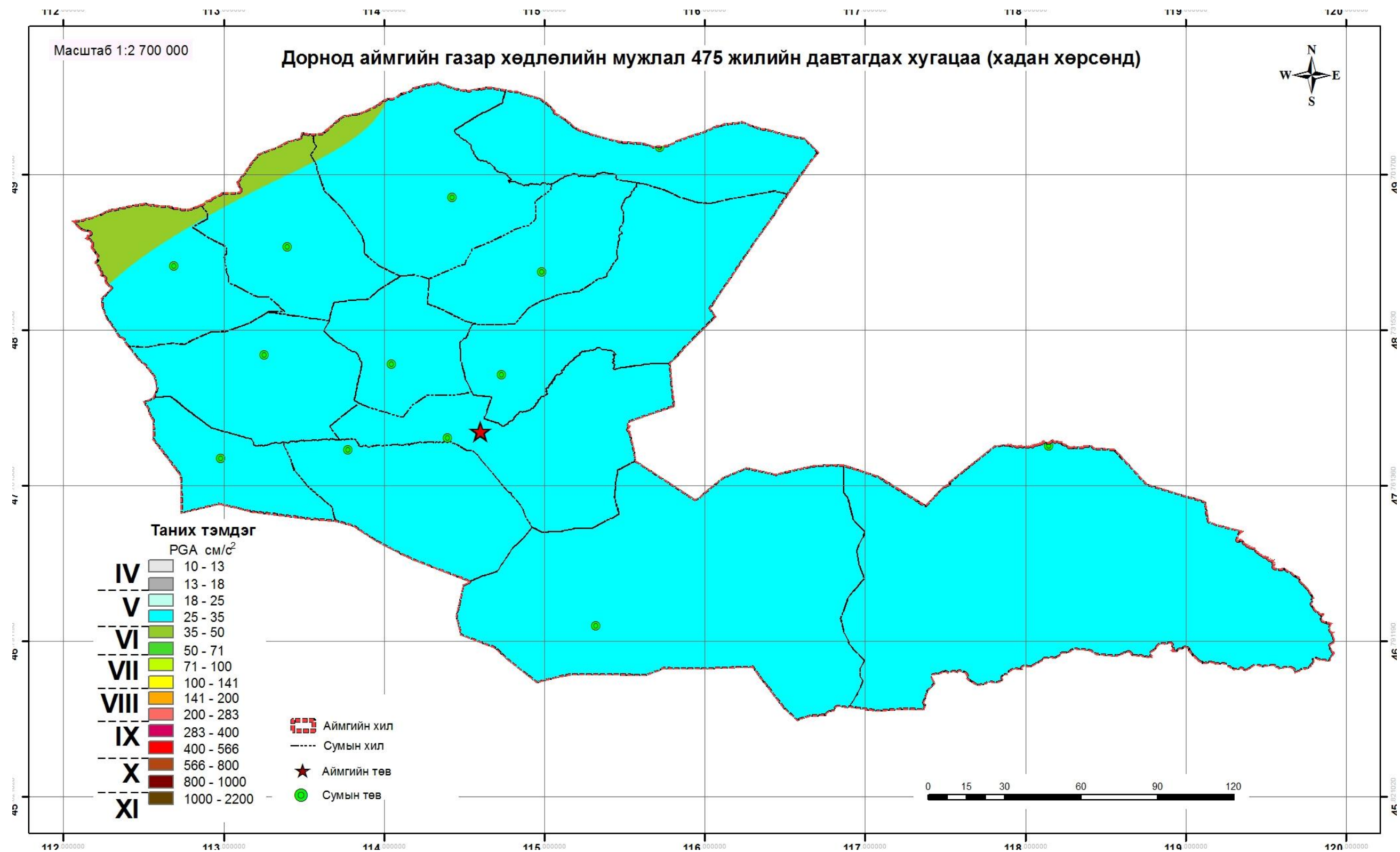
Зураг 130 Дорнод аймгийн төв Хэрлэн сумын газар хөдлөлийн мужлал (475 жилийн давтагдах хугацаа-хадан хөрсөнд)
