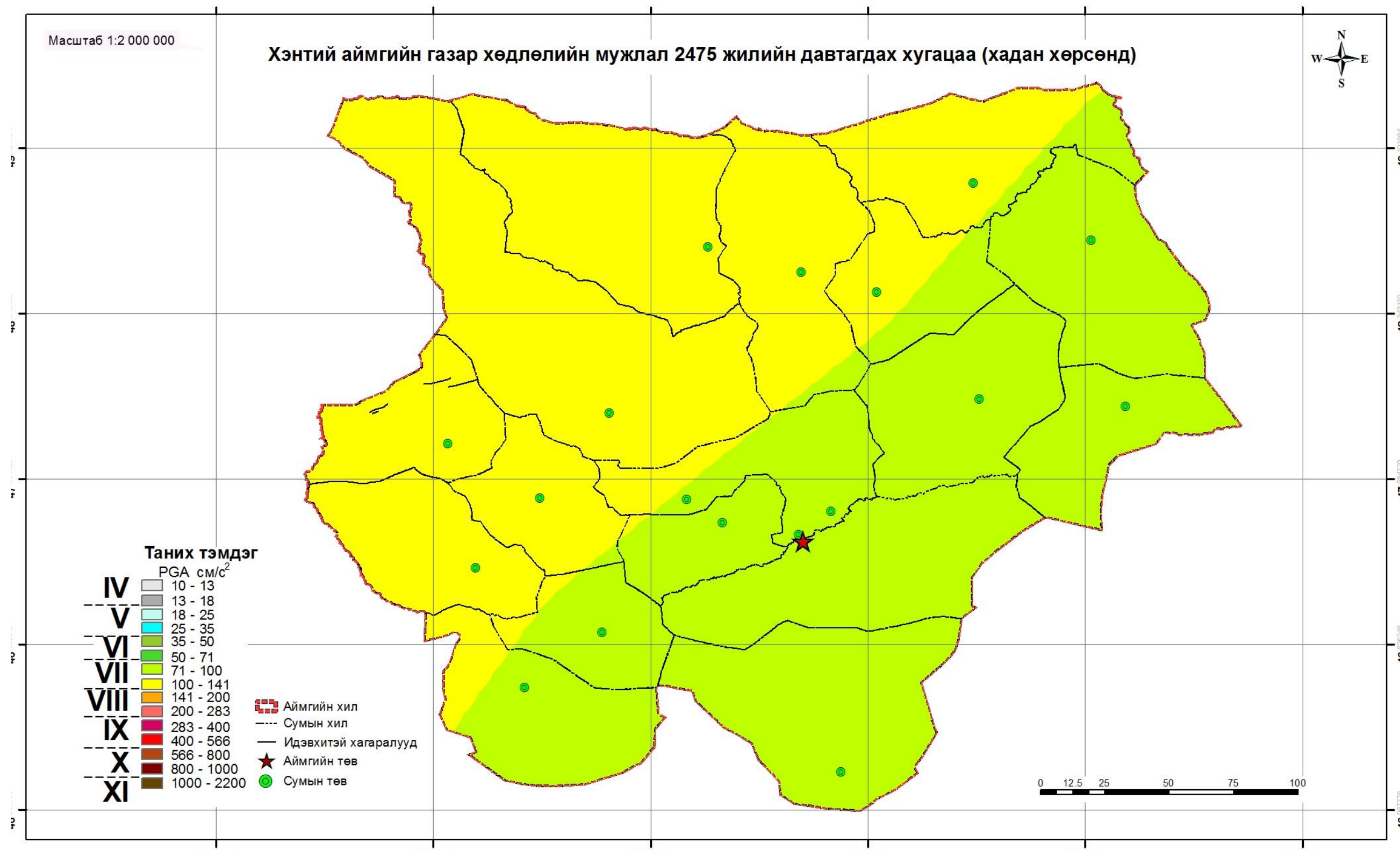
Зураг 98 Хэнтий аймгийн төв Хэрлэн сумын газар хөдлөлийн мужлал (2475 жилийн давтагдах хугацаа- хадан хөрсөнд)
