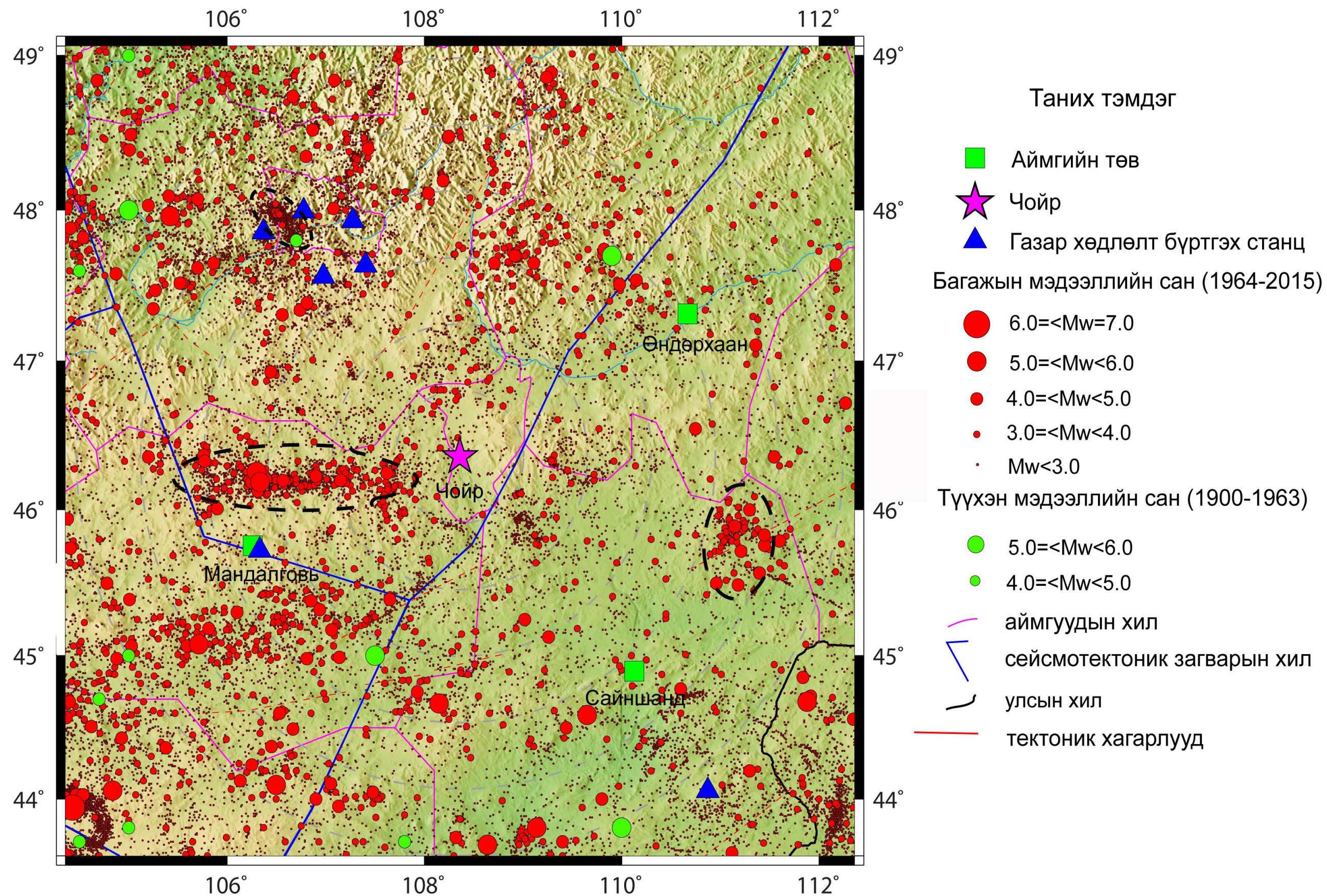
Зураг 74 Говьсүмбэр аймгийн төв Сүмбэр сумын газар хөдлөлийн идэвхжилт.
