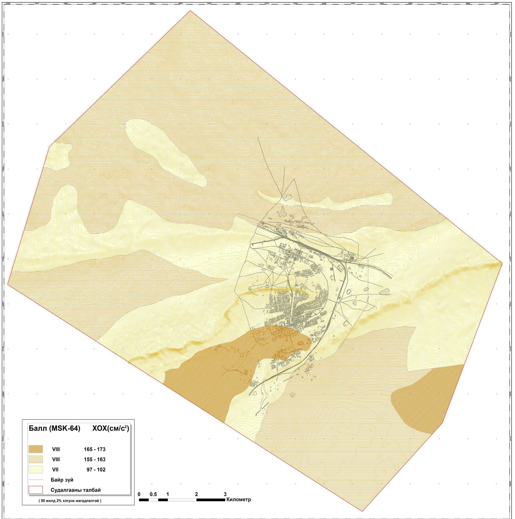
Зураг 58 Дорноговь аймгийн төв Сайншанд сумын газар хөдлөлийн бичил мужлалын зураг (2500 жил )
