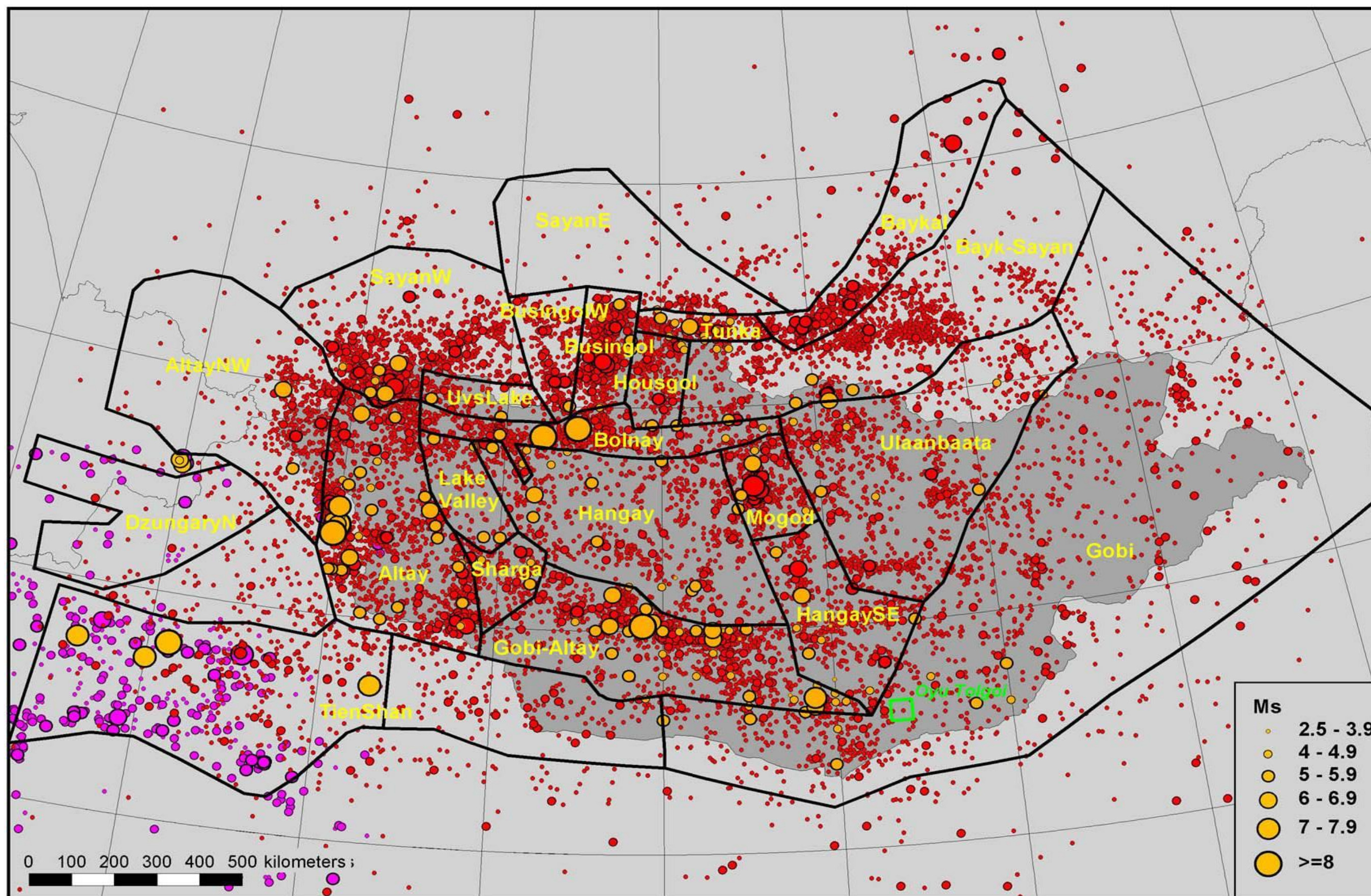
Зураг 3 ГХАУ- ний судалгаанд хэрэглэсэн Монголын сейсмотектоник загвар
