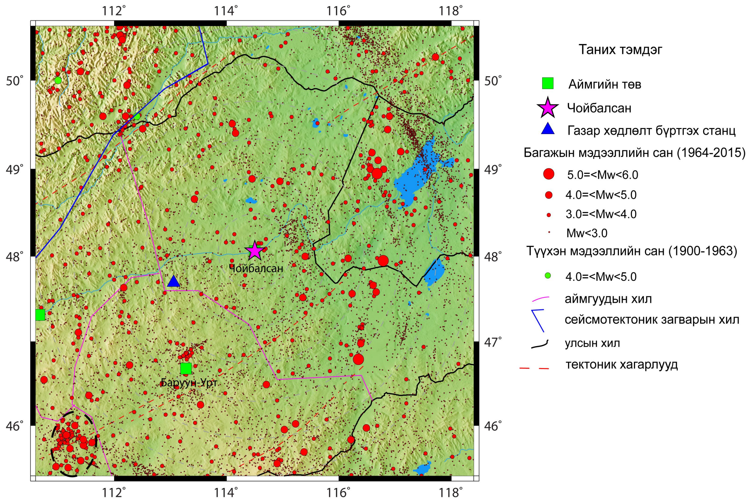
Зураг 129 Дорнод аймаг орчмын газар хөдлөлийн идэвхжилт.
