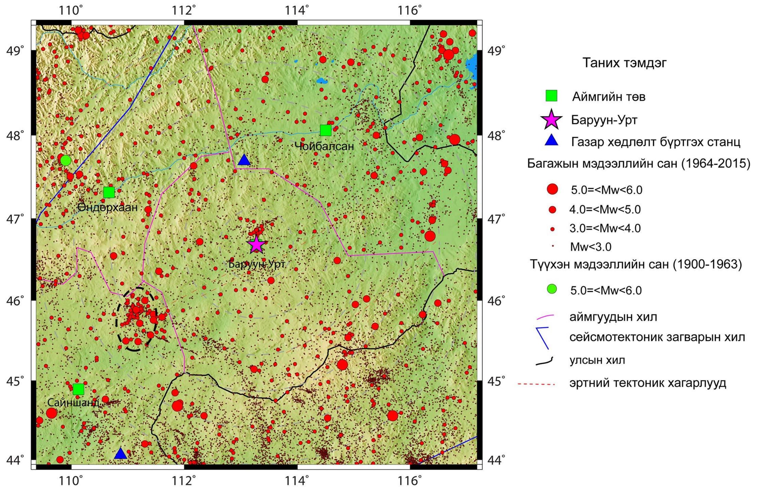
Зураг 107 Сүхбаатар аймгийн төв Баруун- урт сумын газар хөдлөлийн идэвхжилт.
