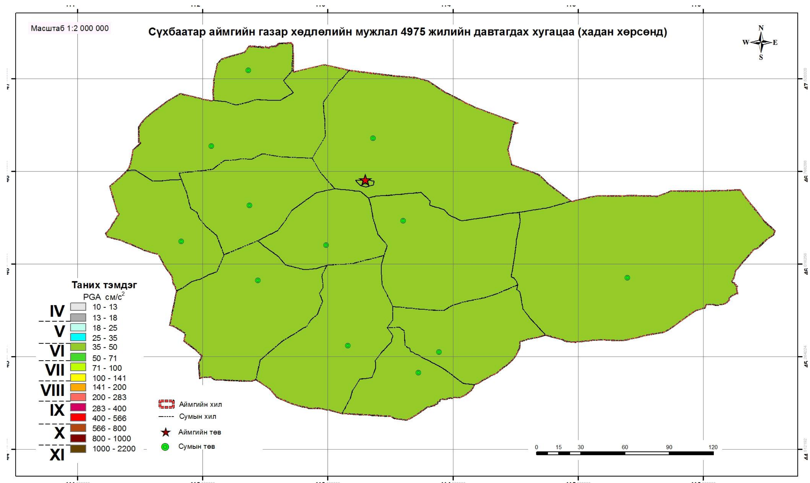
Зураг 110 Сүхбаатар аймгийн төв Баруун- урт сумын газар хөдлөлийн мужлал Суурь үнэлгээ (хадан хөрсөнд)
