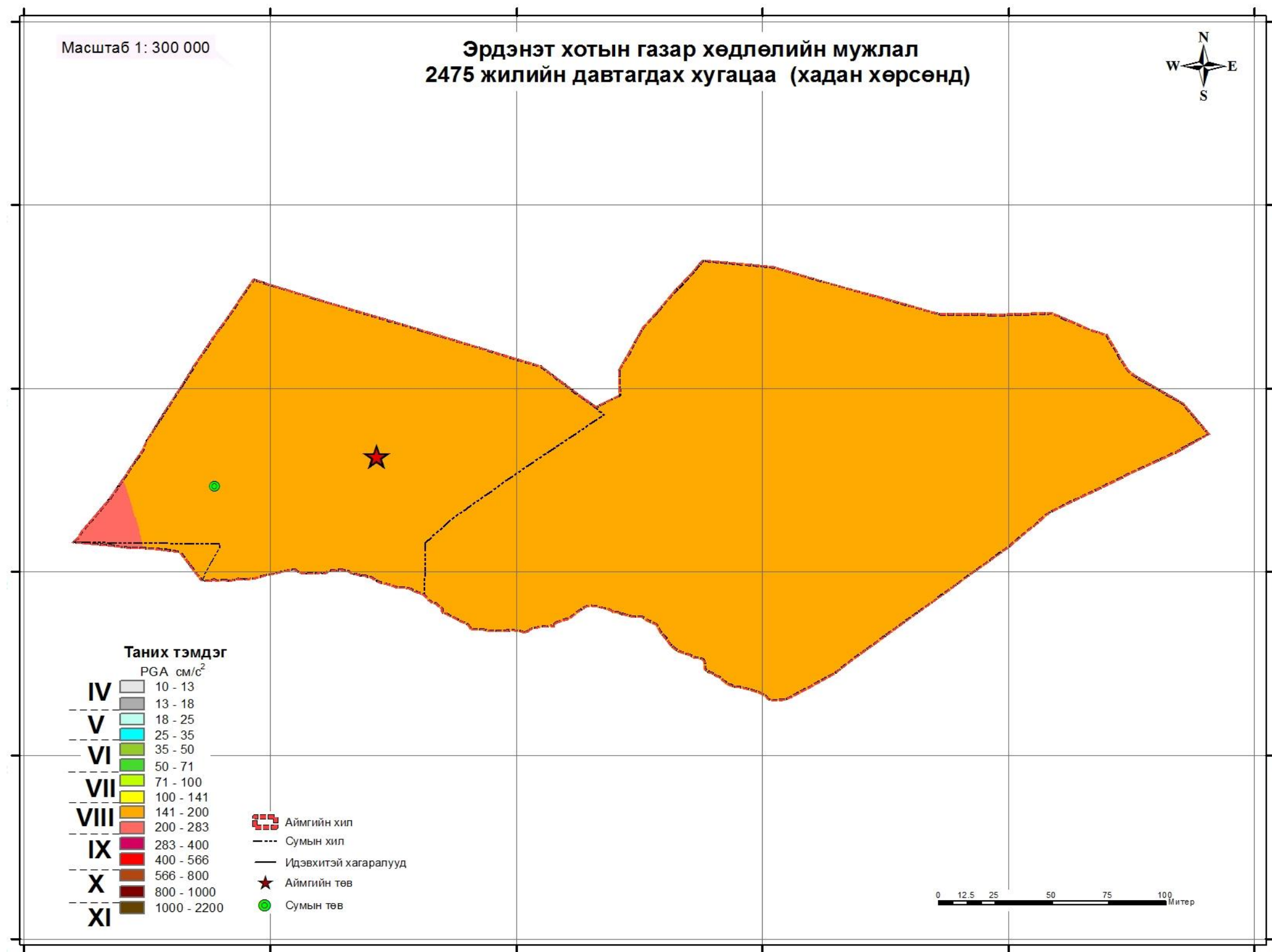
Зураг 87 Орхон аймгийн төв Баян- Өндөр сумын газар хөдлөлийн мужлал (2475 жилийн давтагдах хугацаа-хадан хөрсөнд)
