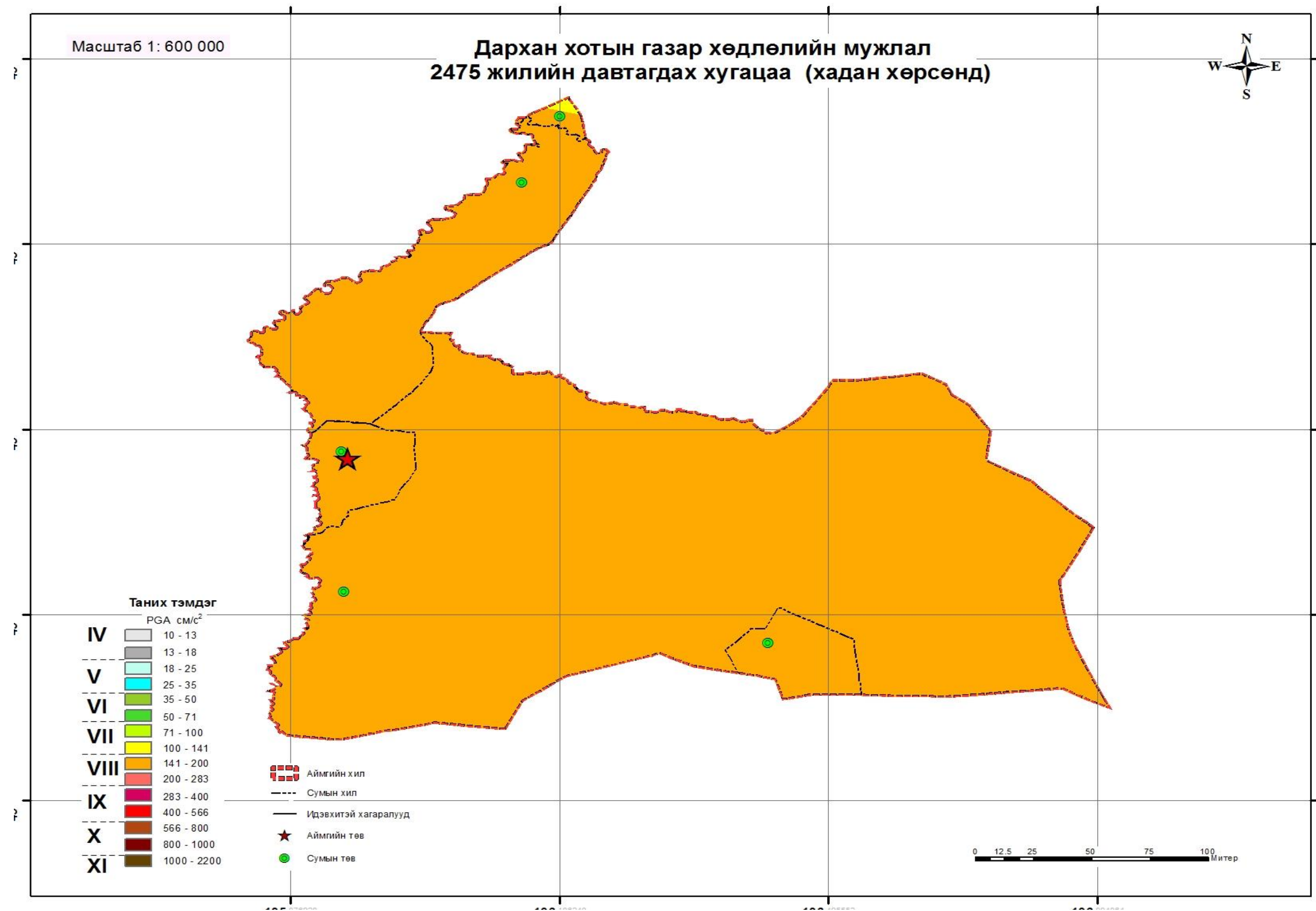
Зураг 43 Дархан- Уул аймгийн төв Дархан сумын газар хөдлөлийн мужлал (2475 жилийн давтагдах хугацаа- хадан хөрсөнд)
