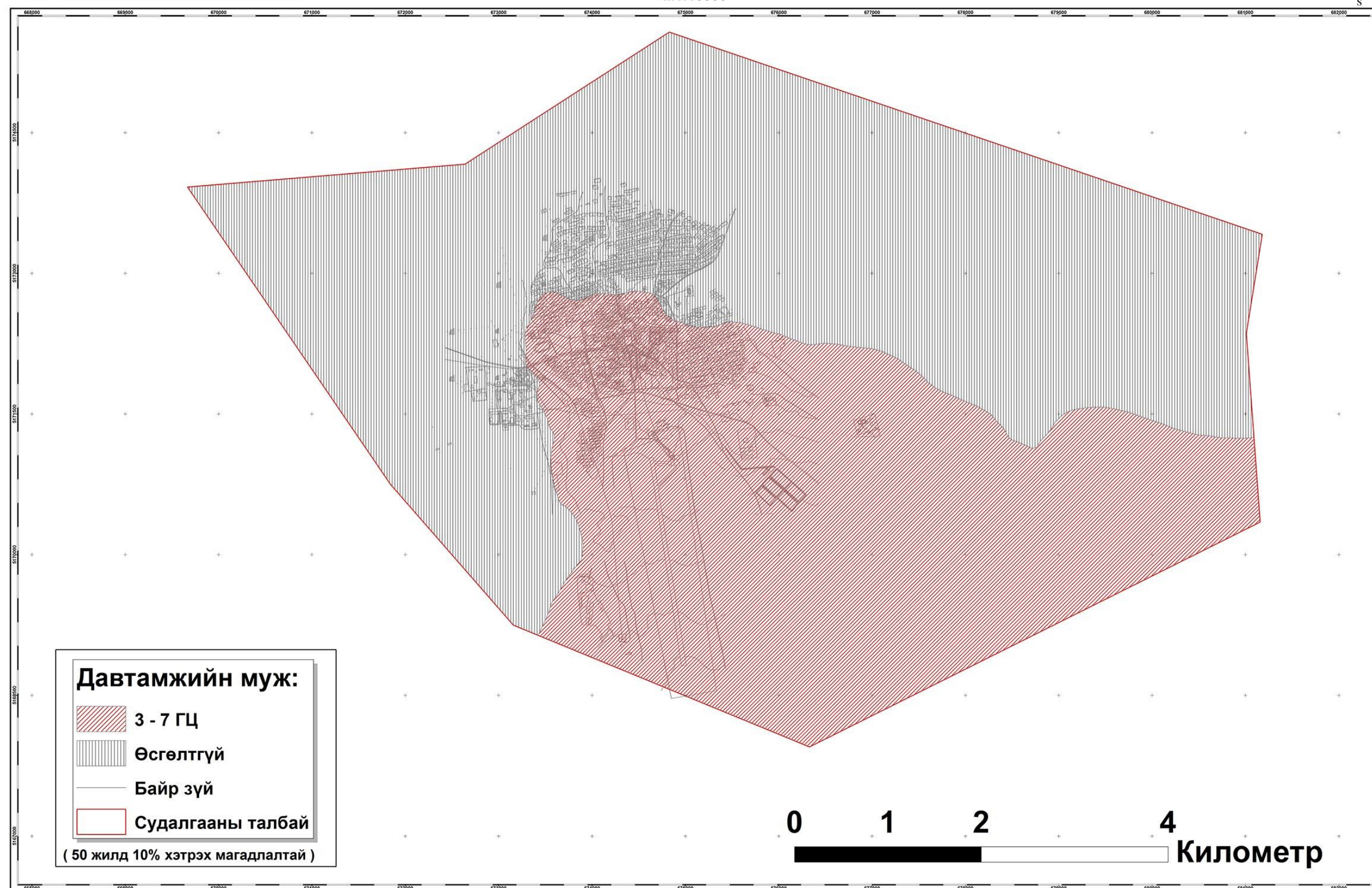
Зураг 111 Сүхбаатар аймгийн төв Баруун- урт сумын хөрсний зонхилох давтамжийн мужлал.
