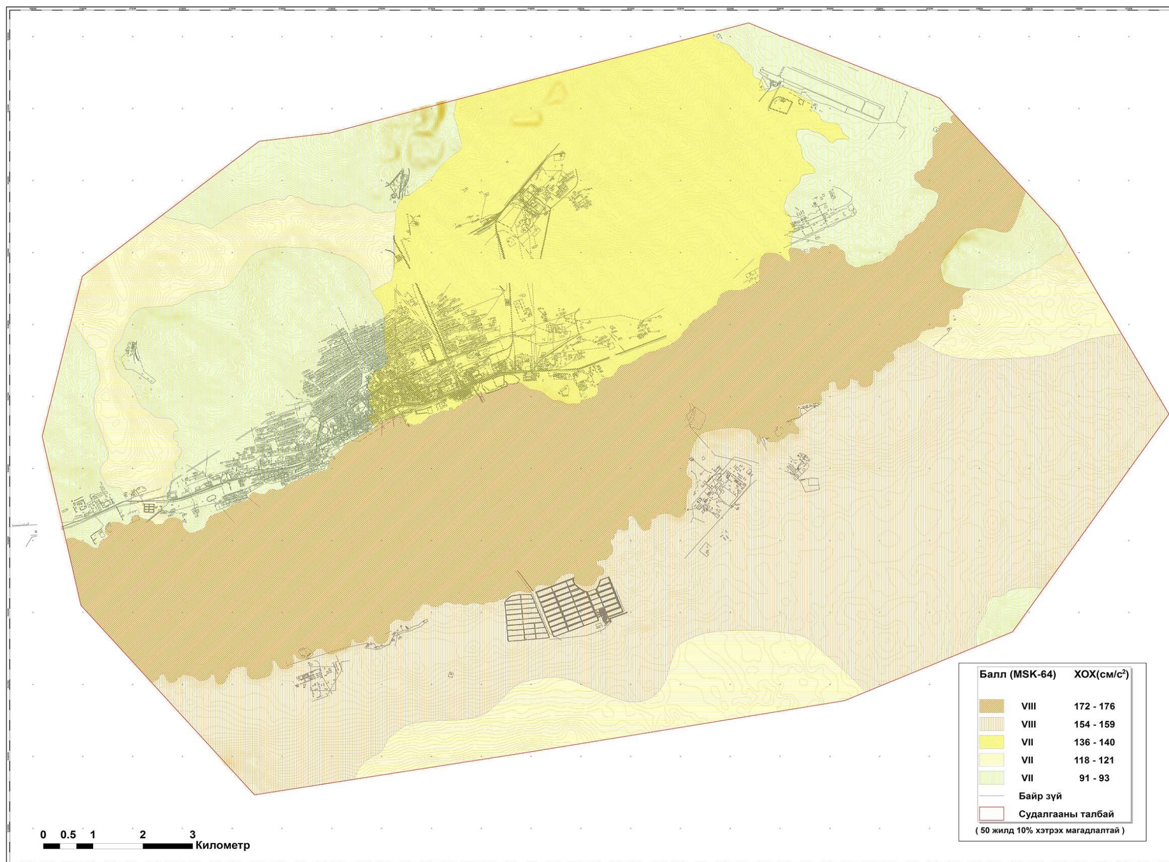
Зураг 135 Дорнод аймгийн төв Хэрлэн сумын газар хөдлөлийн бичил мужлалын зураг (2500 жил)
