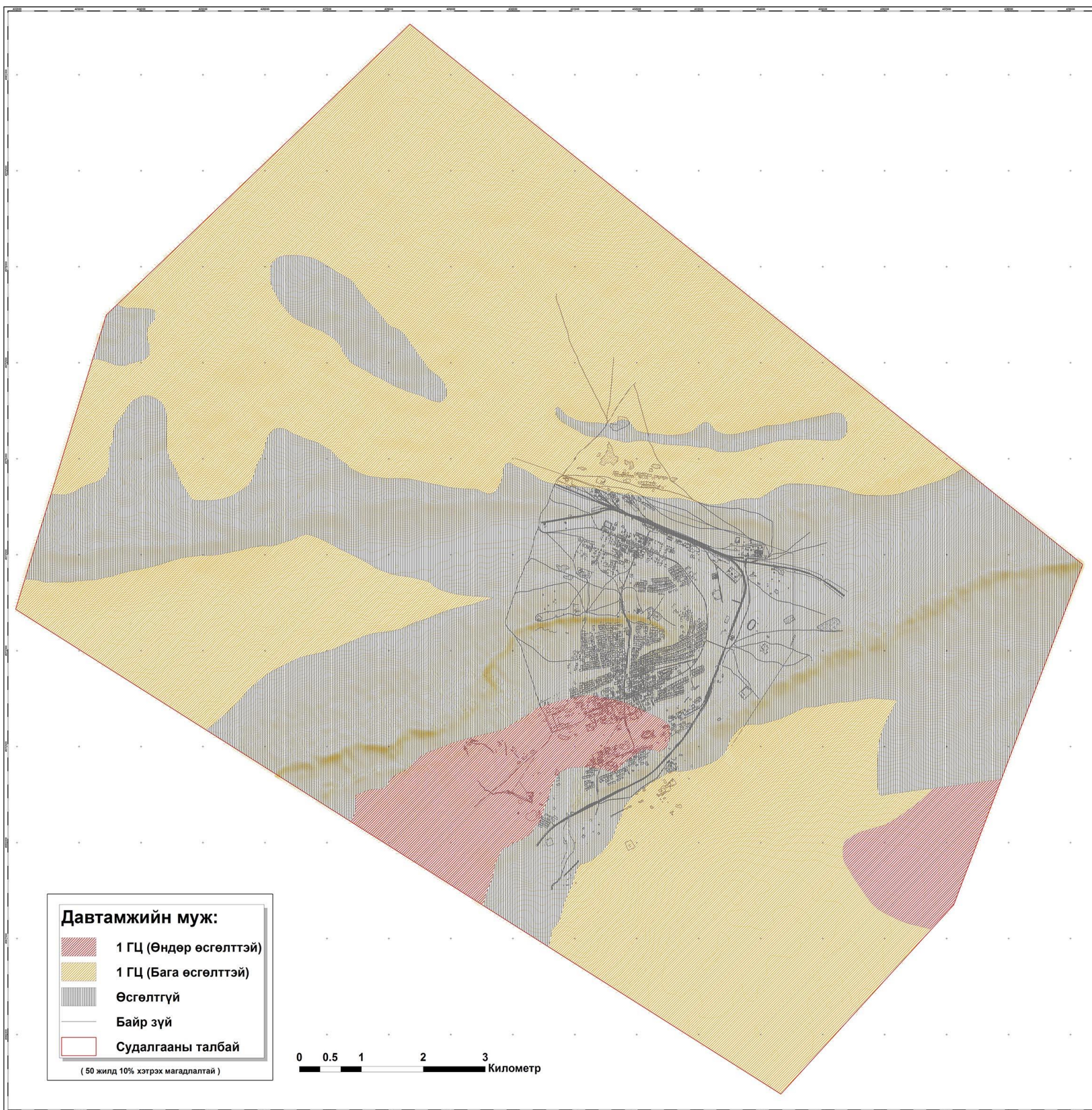
Зураг 56 Дорноговь аймгийн төв Сайншанд сумын хөрсний зонхилох давтамжийн мужлал.
