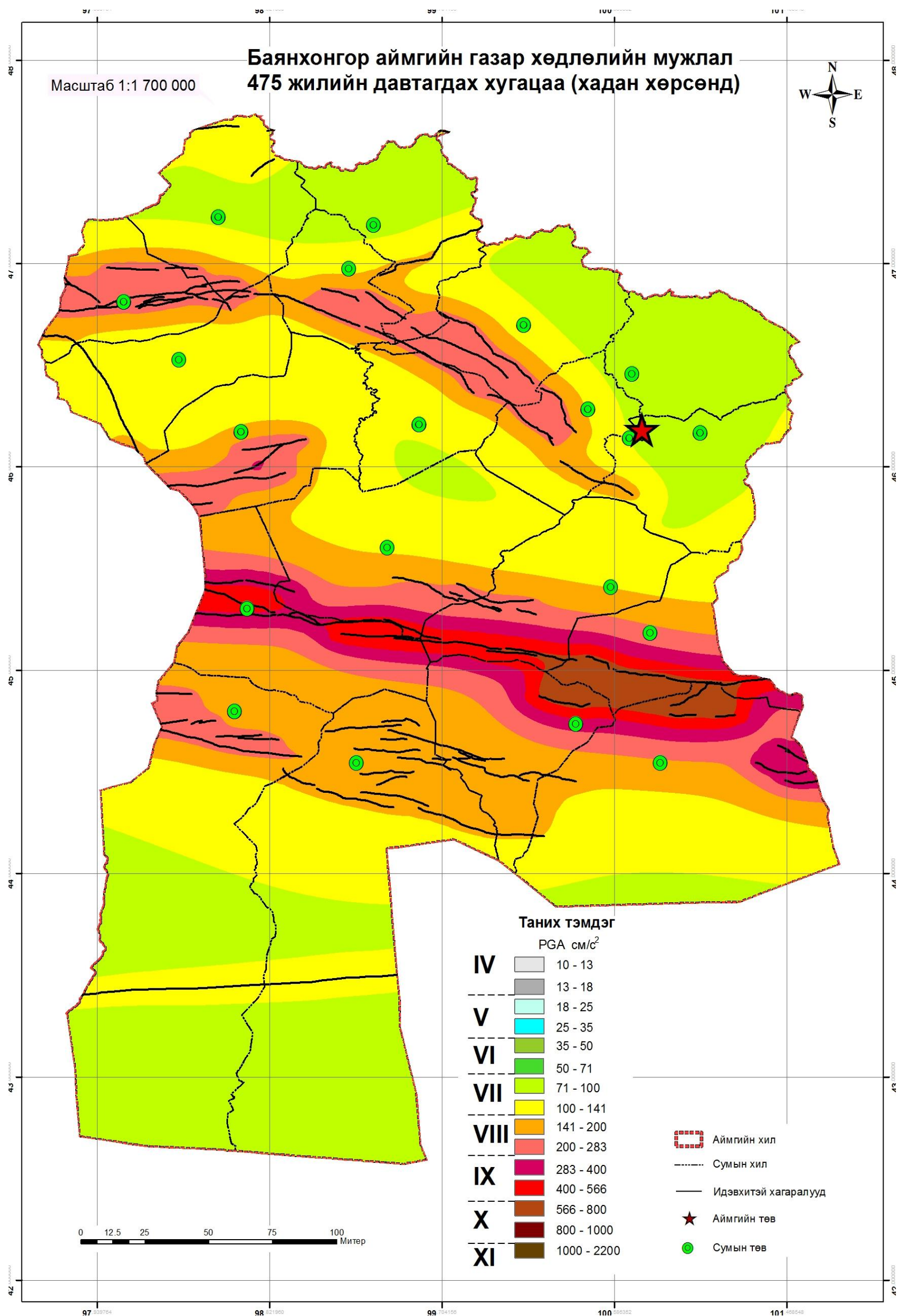
Зураг 20 Баянхонгор аймгийн Баянхонгор сумын газар хөдлөлийн мужлал ( 475 жилийн давтагдах хугацаа хадан хөрсөнд)
