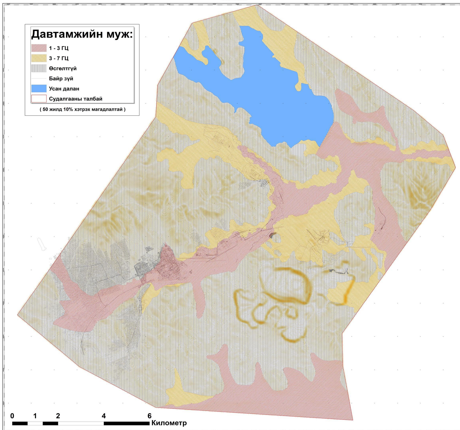
Зураг 89 Орхон аймгийн төв Баян- Өндөр сумын хөрсний зонхилох давтамжийн мужлал.
