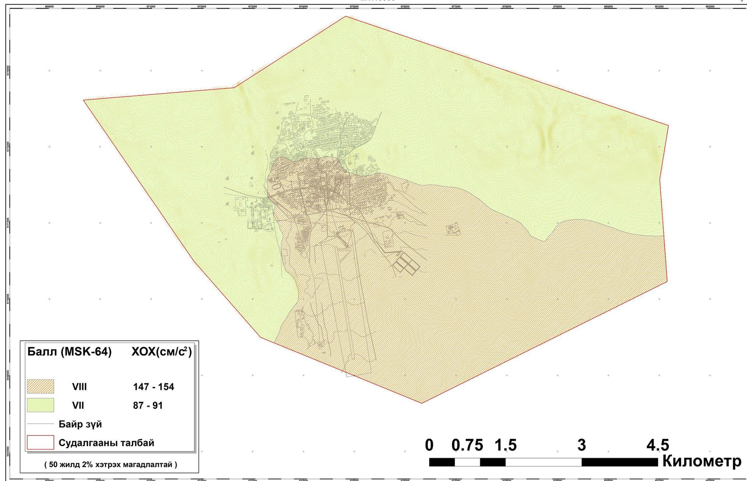
Зураг 113 Сүхбаатар аймгийн төв Баруун- урт сумын газар хөдлөлийн бичил мужлалын зураг (2500 жил )
