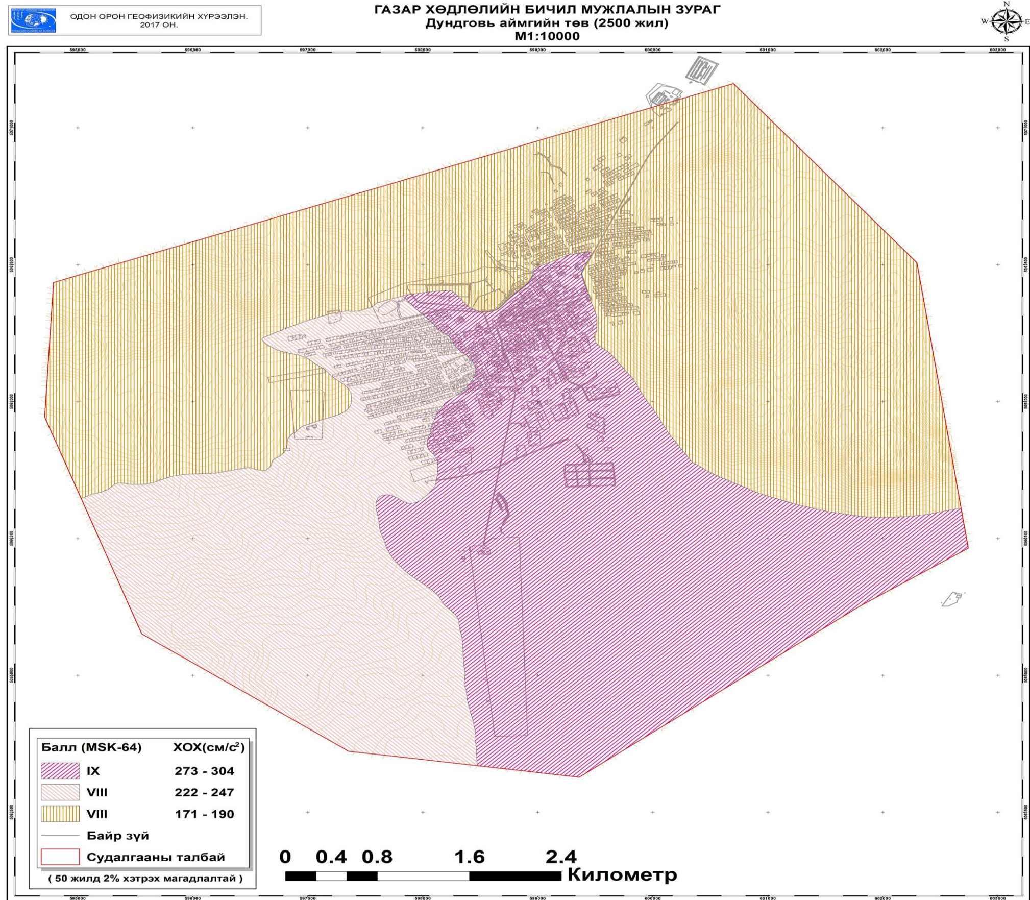
Зураг 69 Дундговь аймгийн төв Сайнцагаан сумын газар хөдлөлийн бичил мужлал (2500 - жил )
