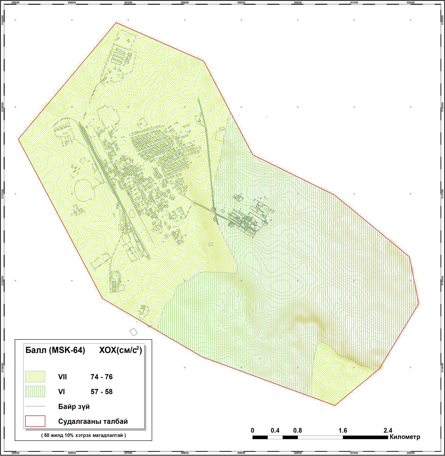
Зураг 79 Говьсүмбэр аймгийн төв Сүмбэр сумын газар хөдлөлийн бичил мужлалын зураг (500 жил )
