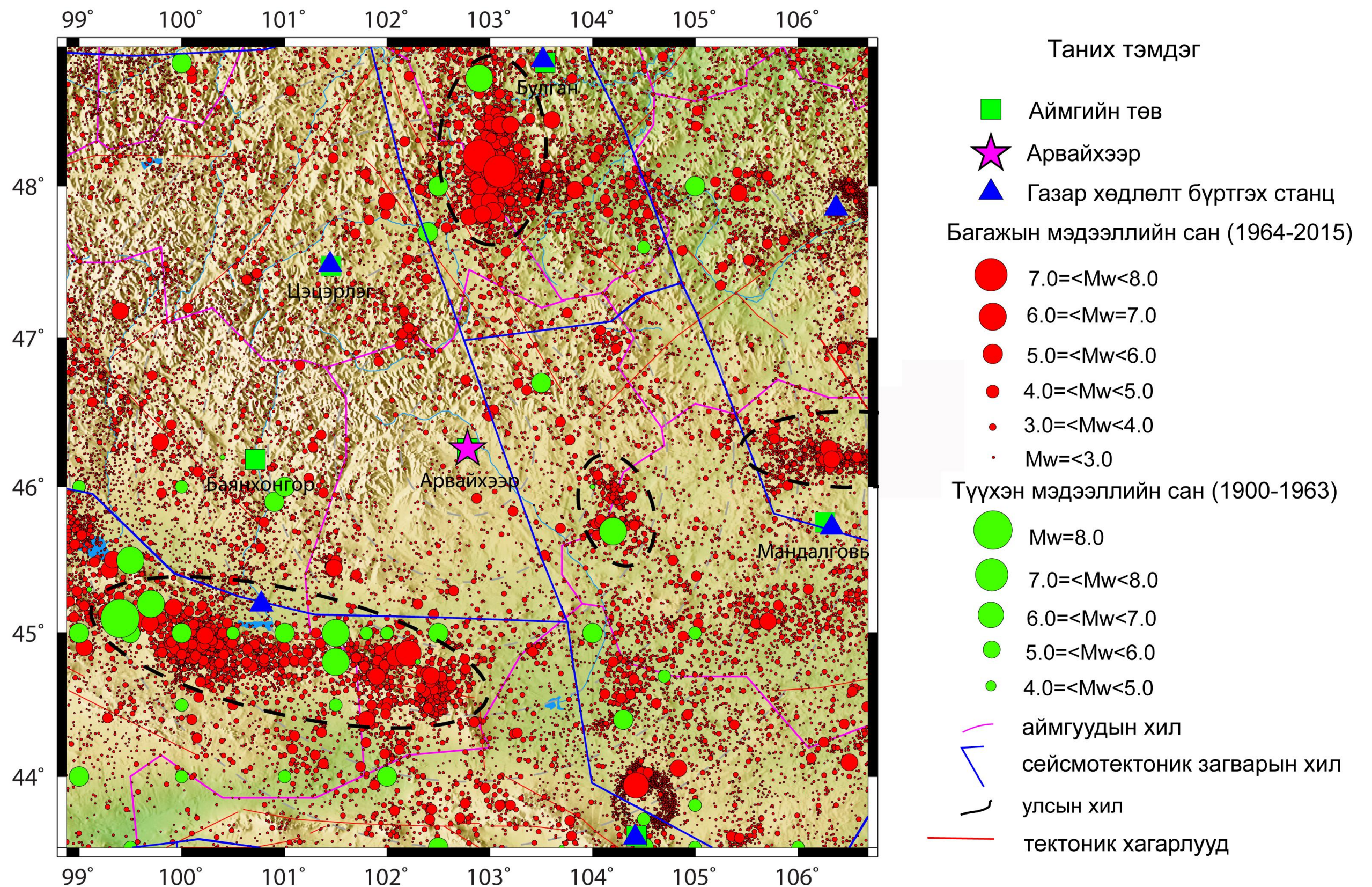
Зураг 118 Өвөрхангай аймаг орчмын газар хөдлөлийн идэвхжилт.
