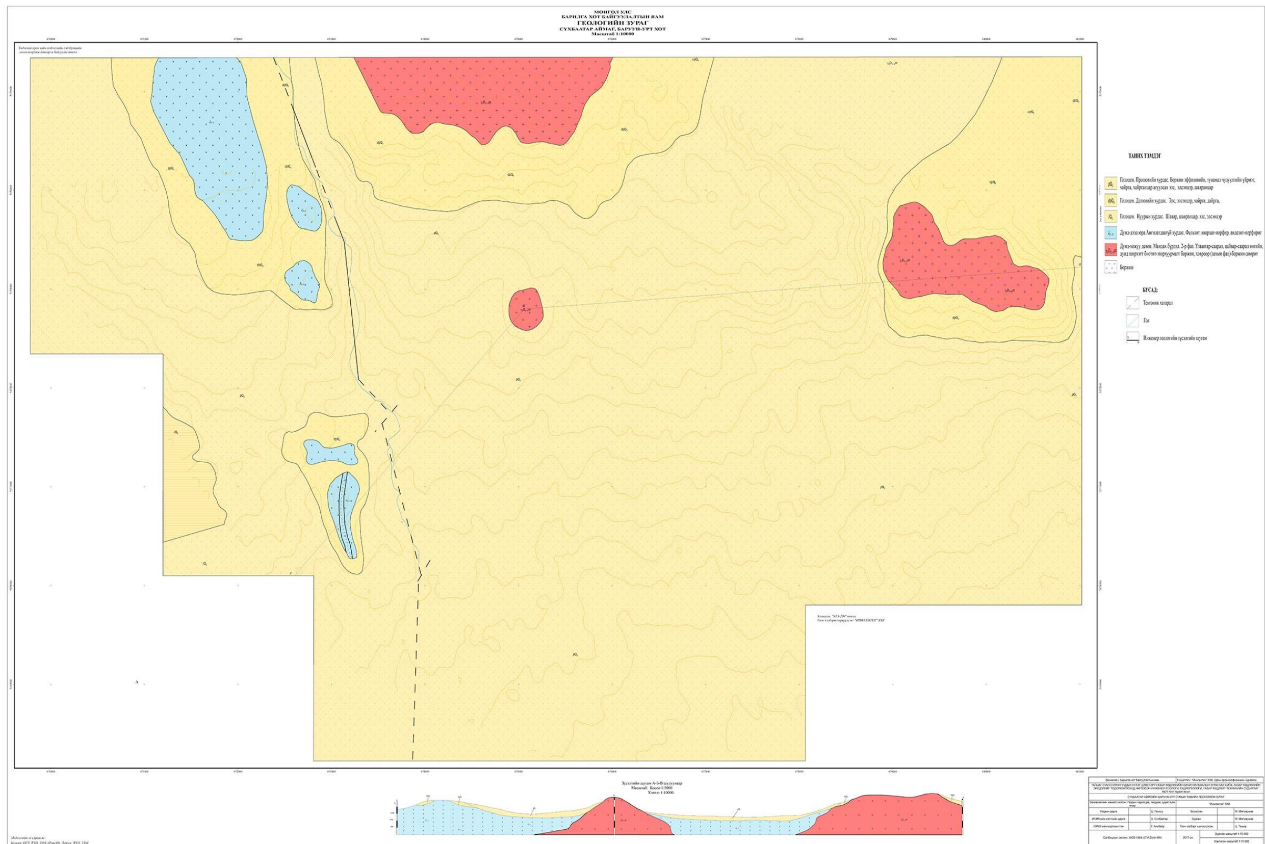
Зураг 103 Сүхбаатар аймгийн төв Баруун- урт сумын геологийн зураг.
