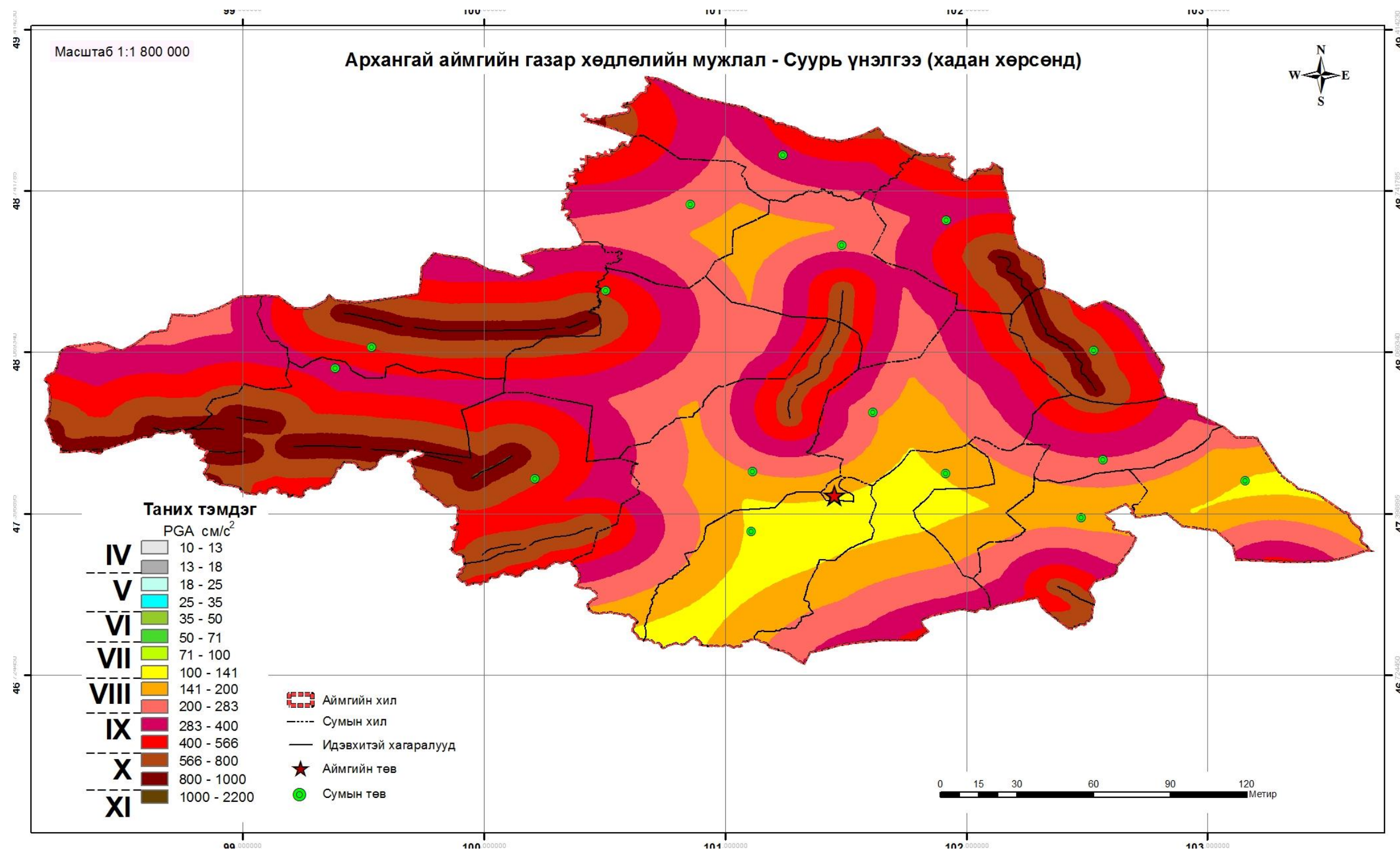
Зураг 11 Архангай аймгийн төв Эрдэнэбулган сумын газар хөдлөлийн мужлал Суурь үнэлгээ хадан хөрсөнд)
