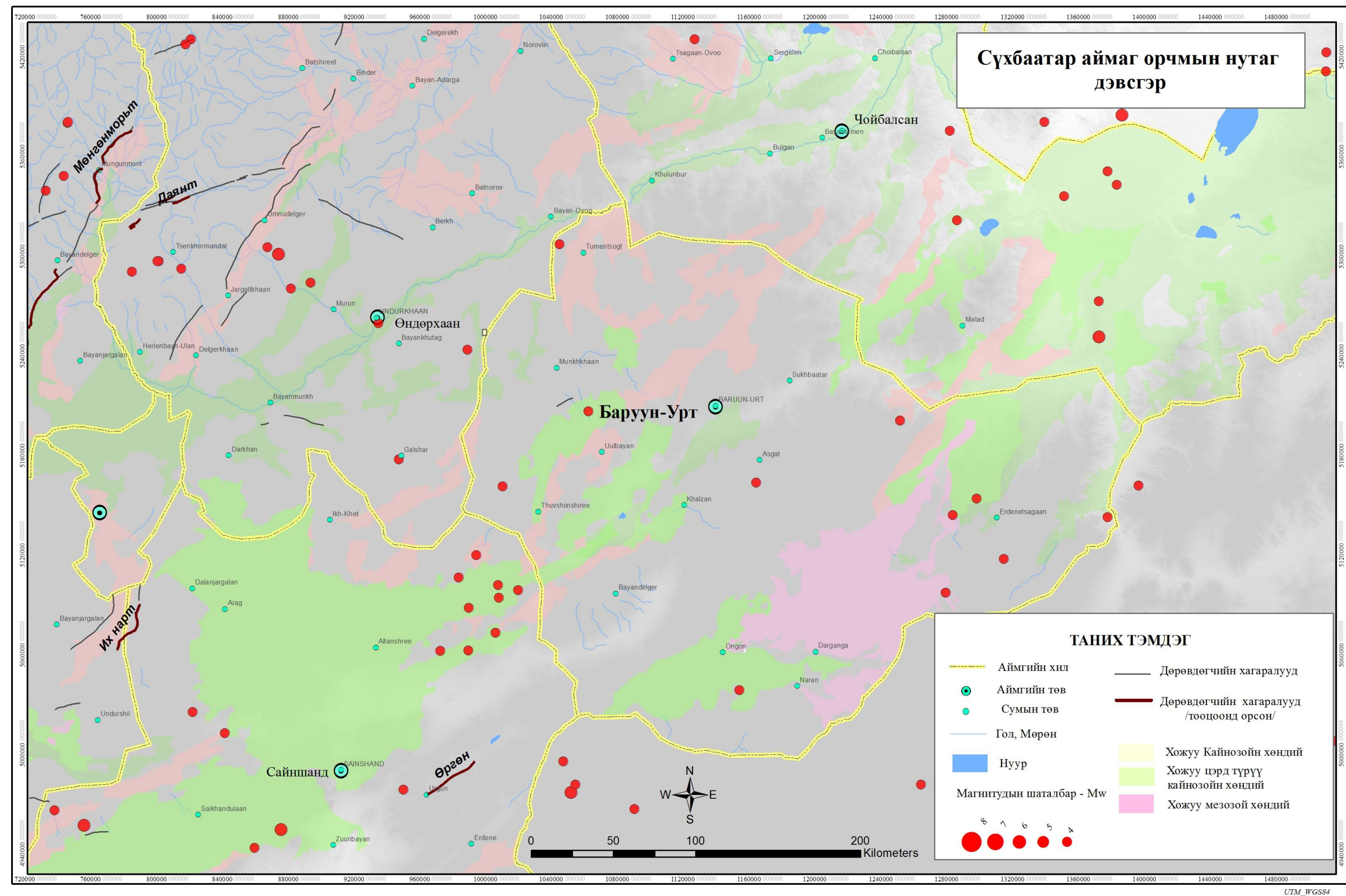
Зураг 106 Сүхбаатар аймгийн төв Баруун- урт сумын сейсмотектоникийн тойм зураг
