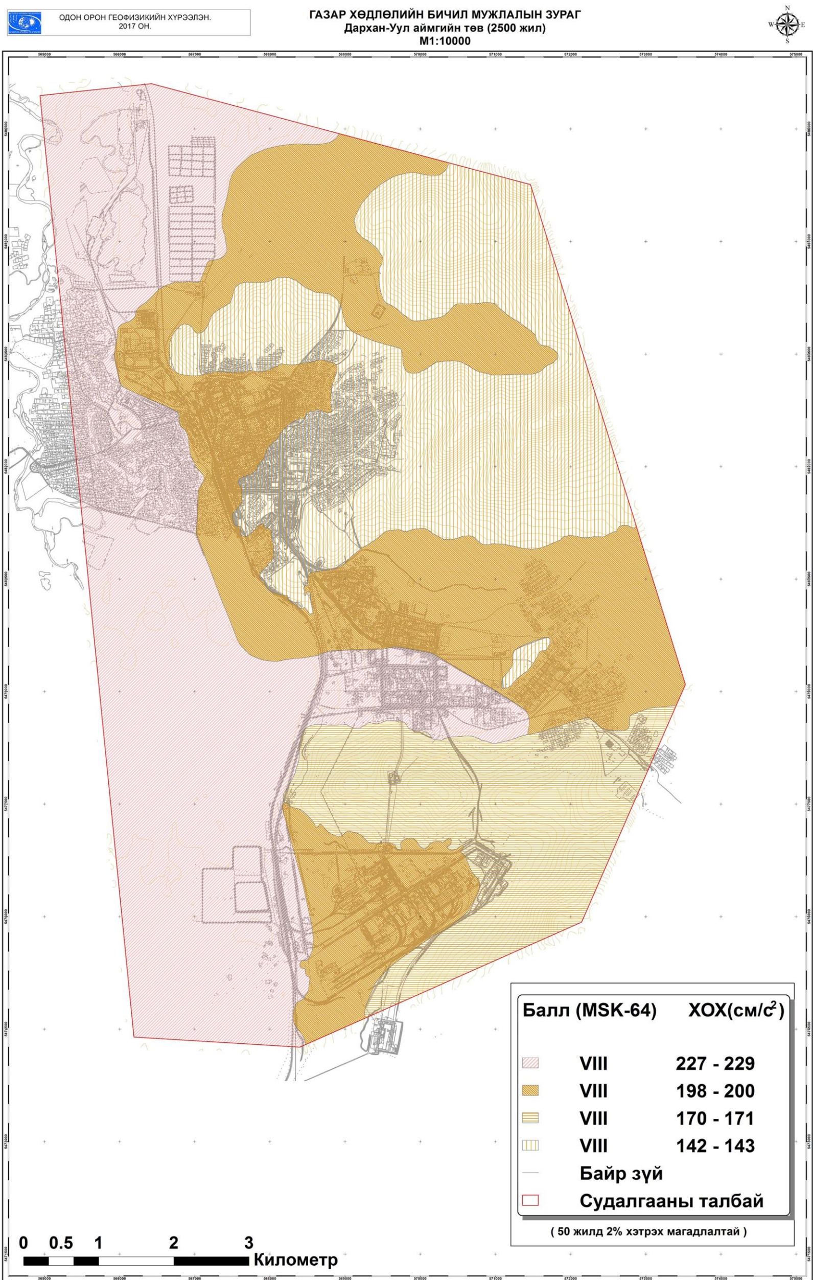
Зураг 47 Дархан- Уул аймгийн төв Дархан сумын газар хөдлөлийн бичил мужлал (2500 жил )
