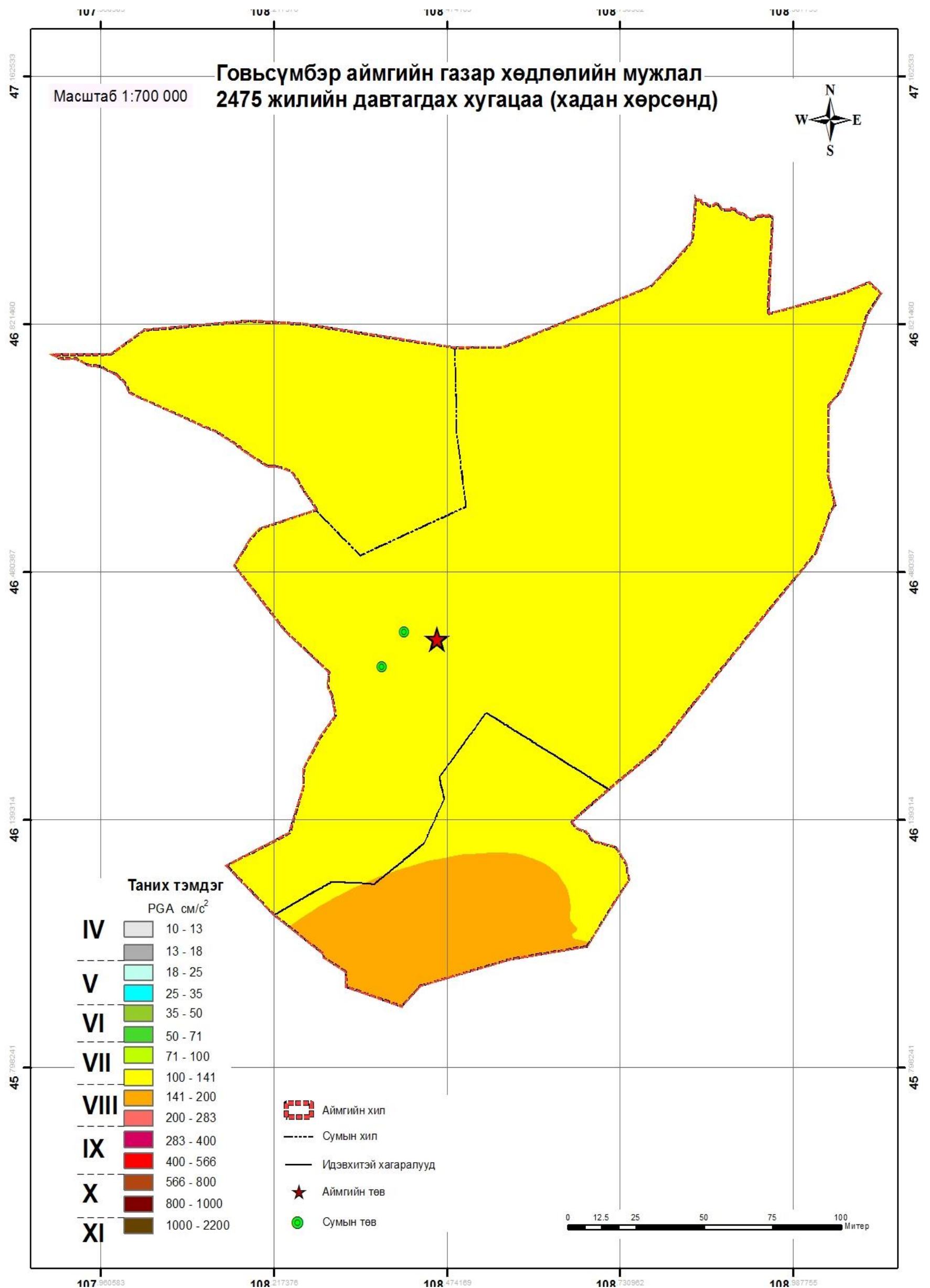
Зураг 76 Говьсүмбэр аймгийн төв Сүмбэр сумын газар хөдлөлийн мужлал (2475 жилийн давтагдах хугацаа- хадан хөрсөнд)
