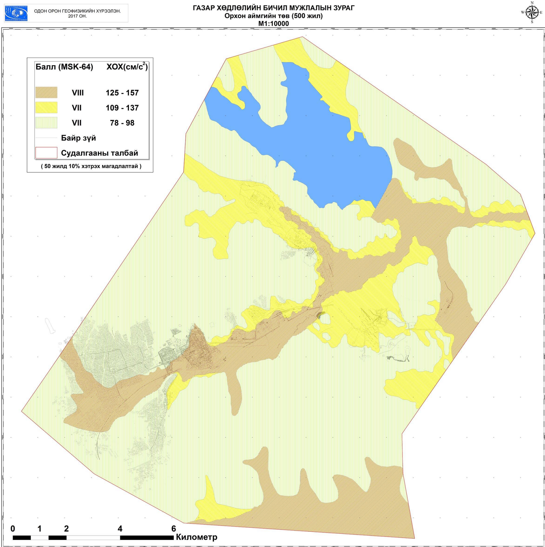
Зураг 90 Орхон аймгийн төв Баян- Өндөр сумын газар хөдлөлийн бичил мужлалын зураг (500- жил )
