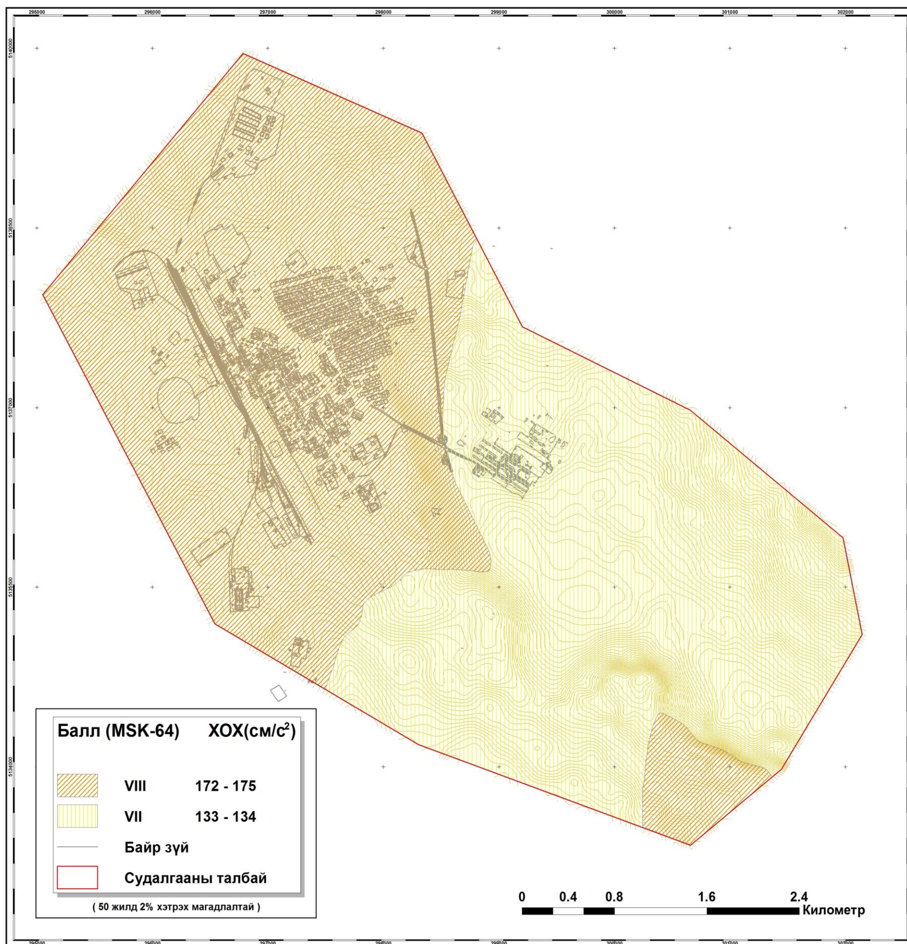
Зураг 80 Говьсүмбэр аймгийн төв Сүмбэр сумын газар хөдлөлийн бичил мужлалын зураг (2500 жил )
