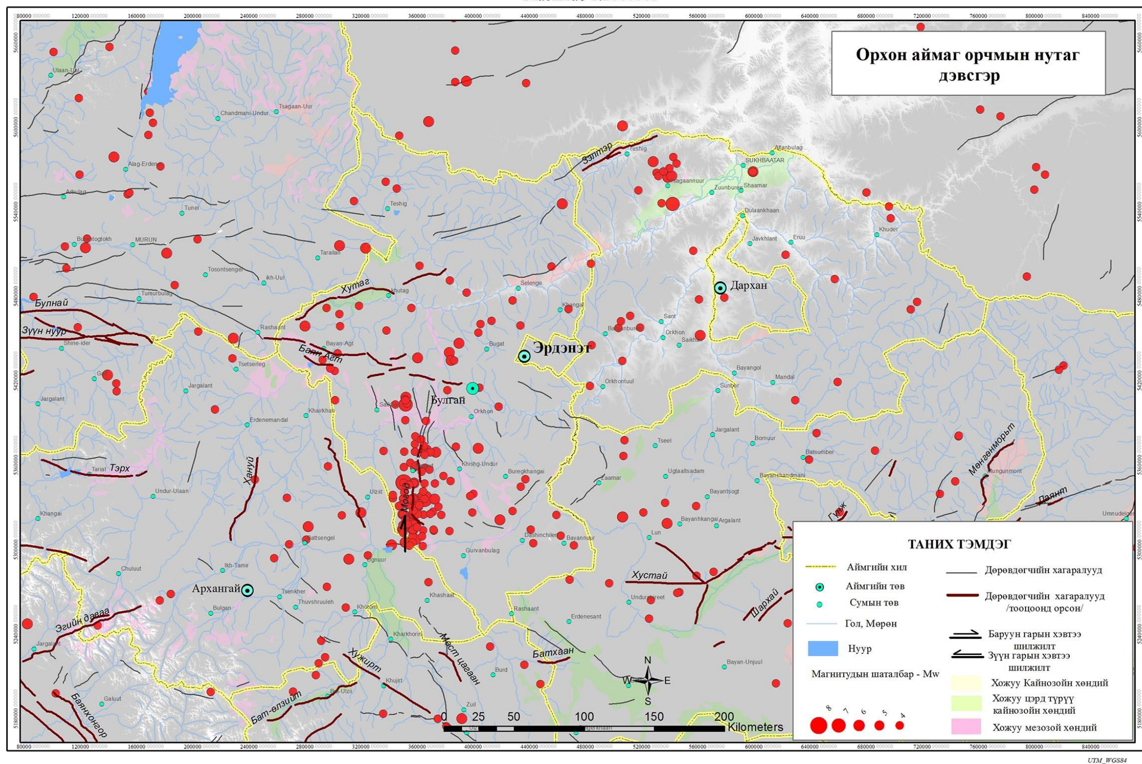
Зураг 84 Орхон аймгийн төв Баян- Өндөр сумын сейсмотектоникийн тойм зураг
