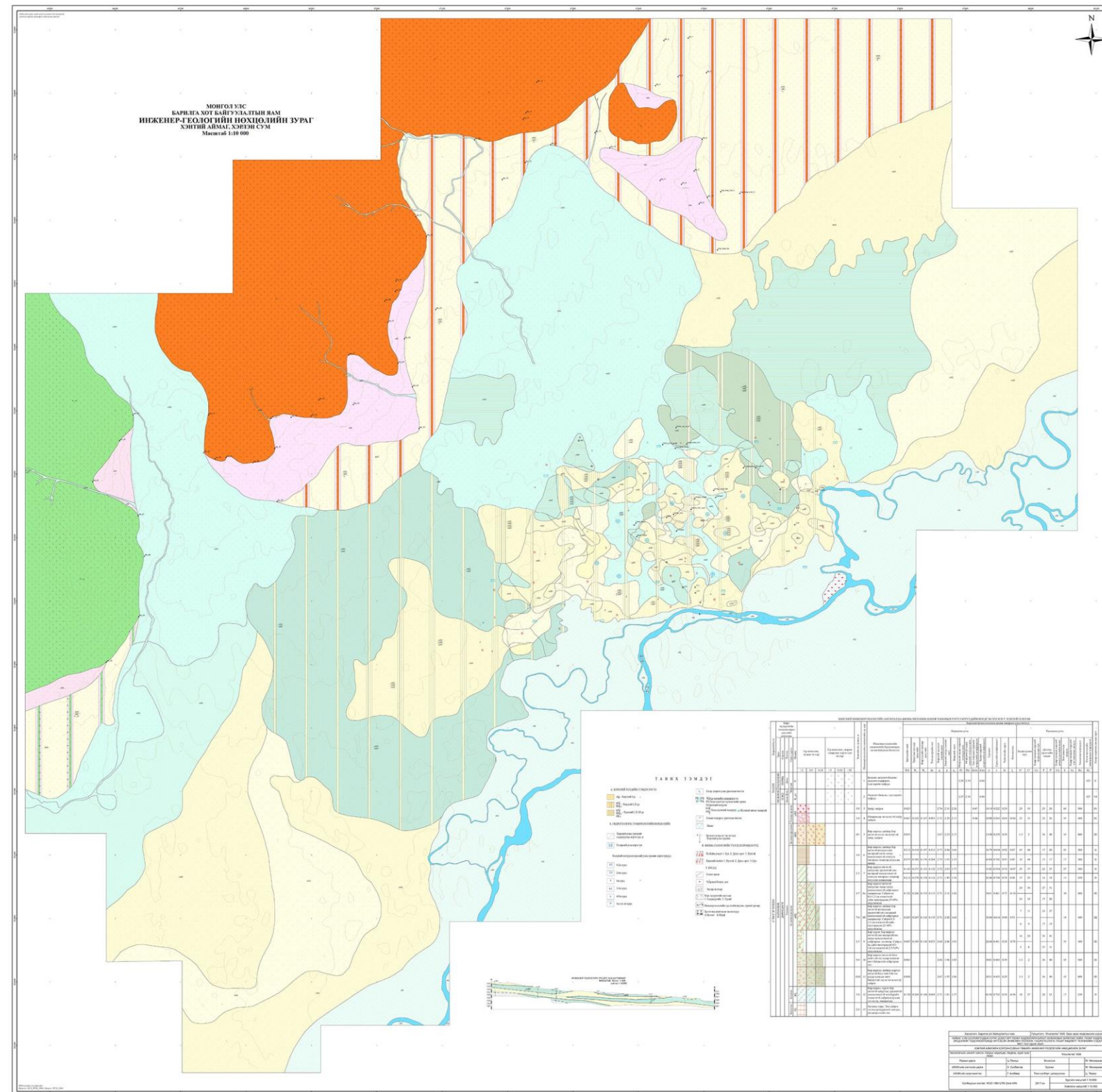
Зураг 93 Хэнтий аймгийн төв Хэрлэн сумын инженер геологийн нөхцөлийн зураг
