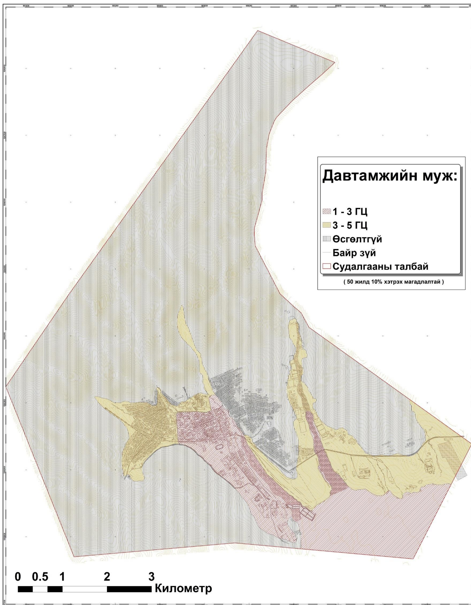
Зураг 12 Архангай аймгийн төв Эрдэнэбулган сумын хөрсний зонхилох давтамжийн мужлал
