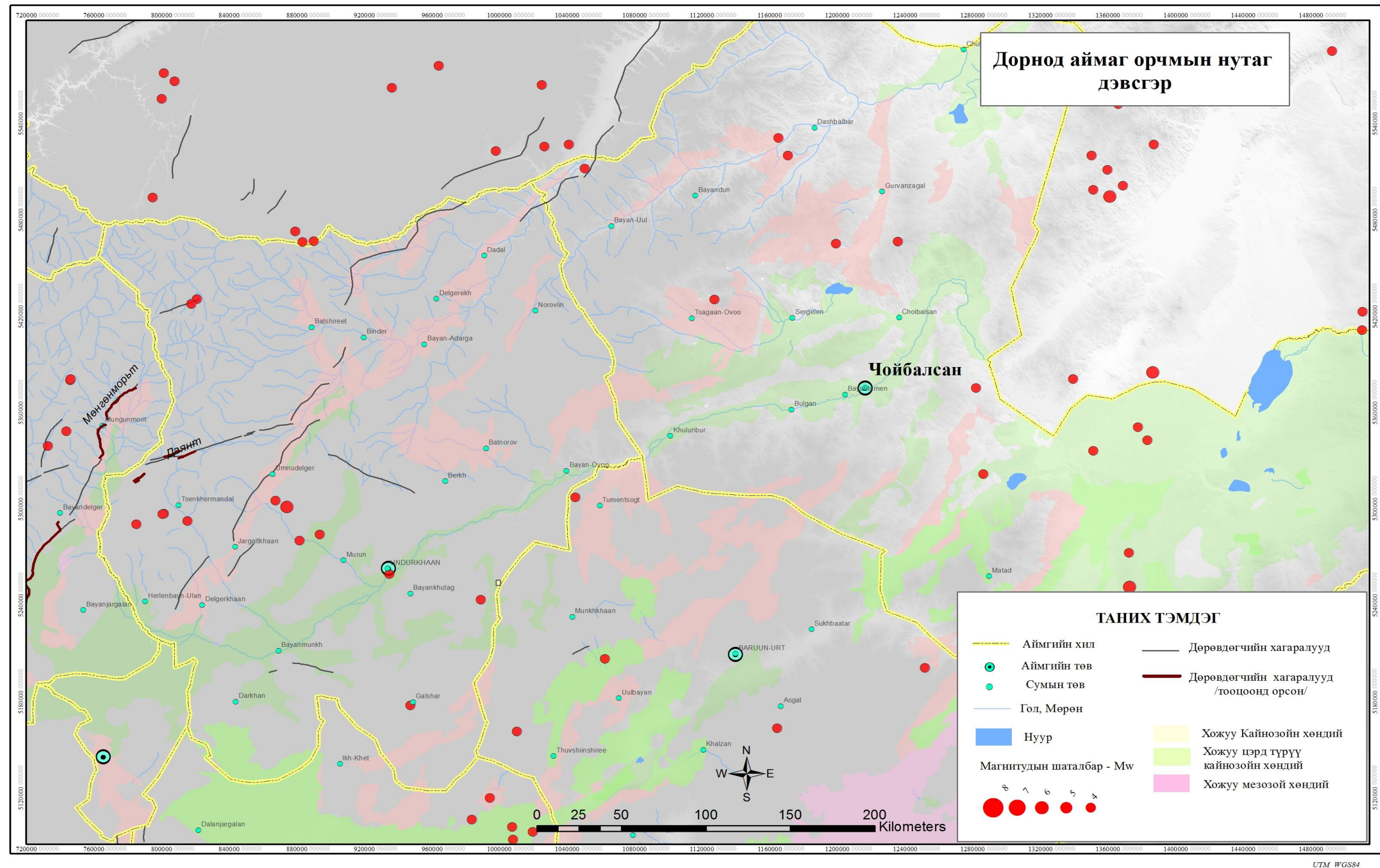
Зураг 128 Дорнод аймгийн төв Хэрлэн сумын сейсмостектоникийн тойм зураг
