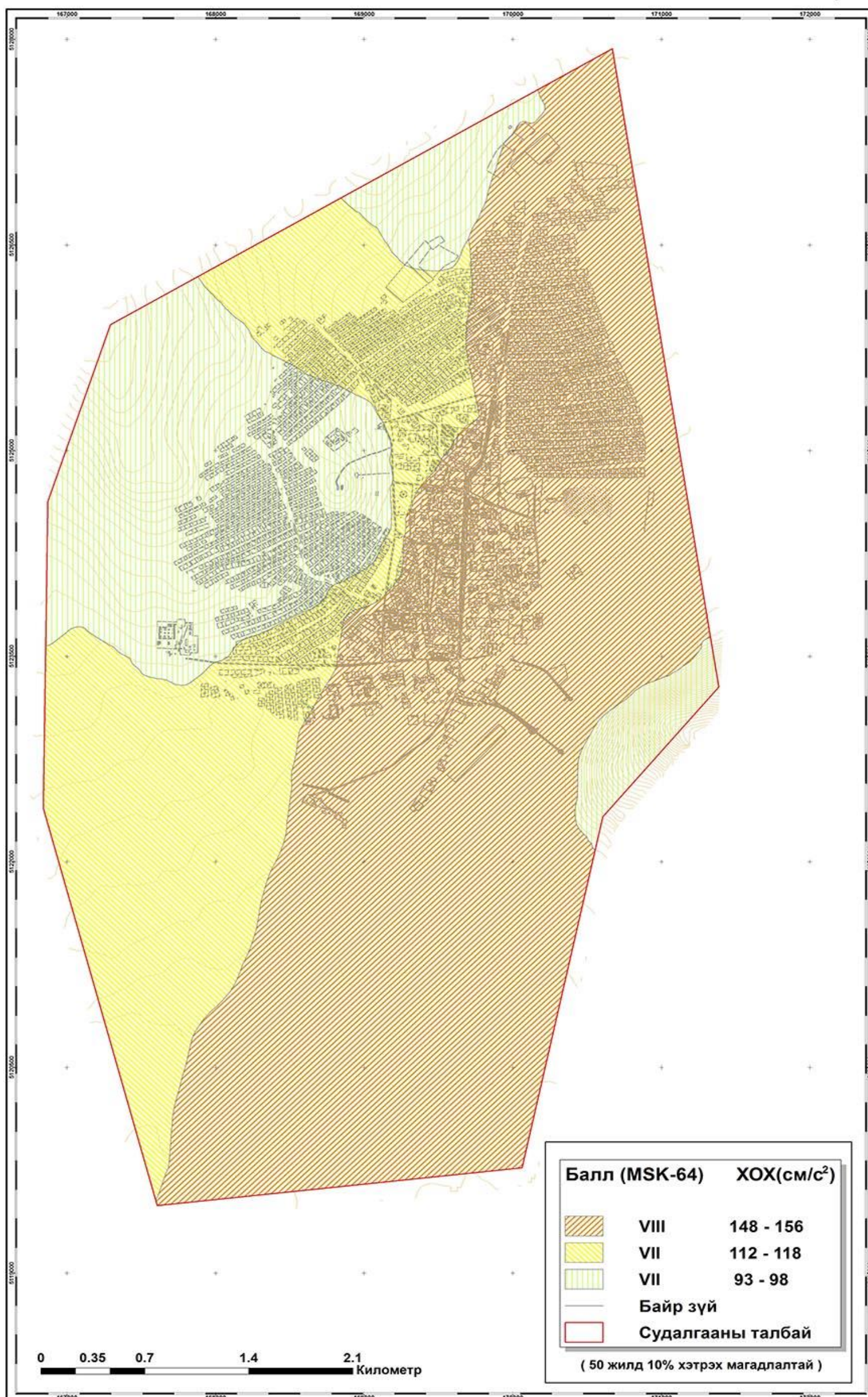
Зураг 24 Баянхонгор аймгийн Баянхонгор сумын газар хөдлөлийн бичил мужлал (500- жил )
