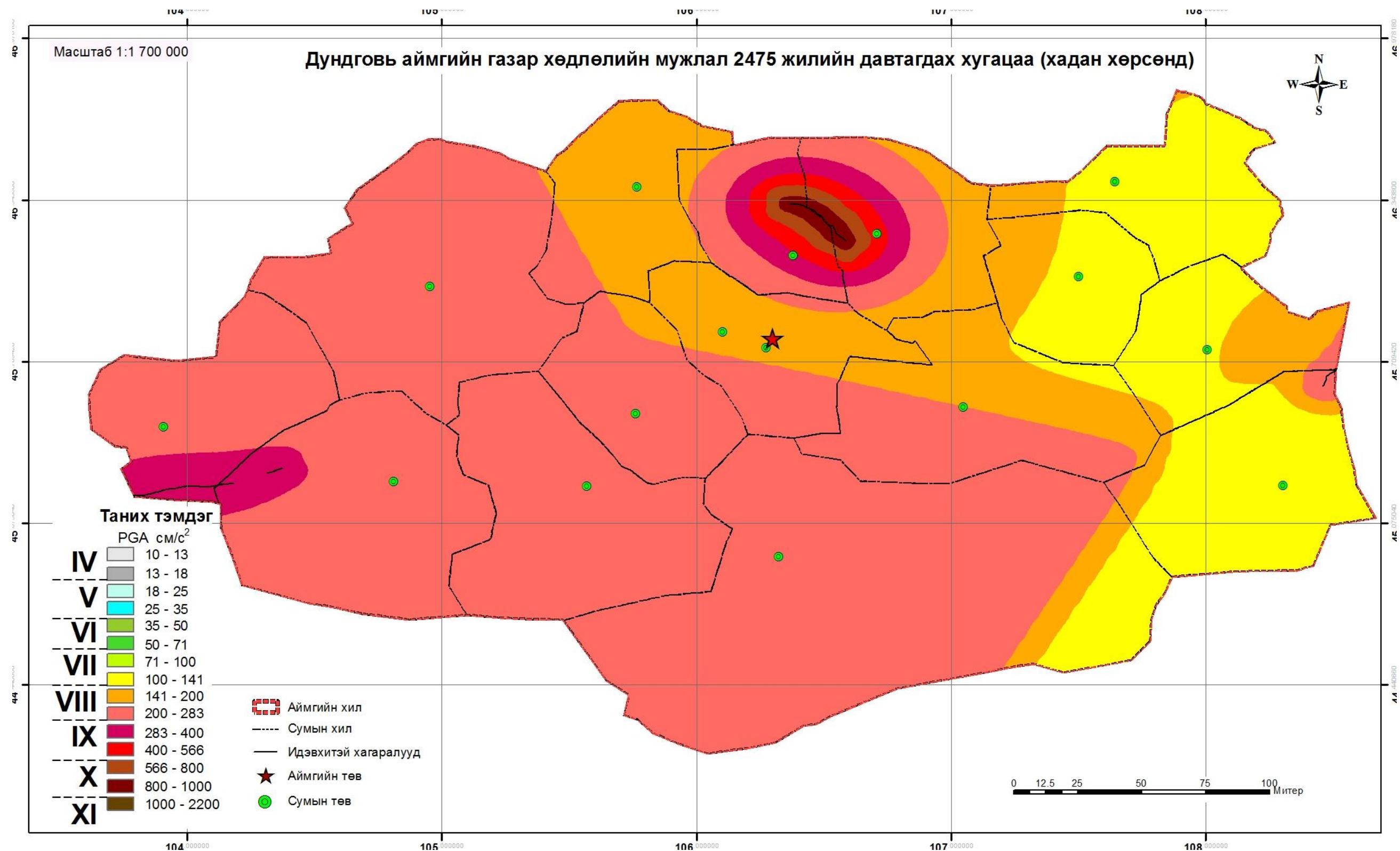
Зураг 65 Дундговь аймгийн төв Сайнцагаан сумын газар хөдлөлийн мужлал (2475 жилийн давтагдах хугацаа- хадан хөрсөнд)
