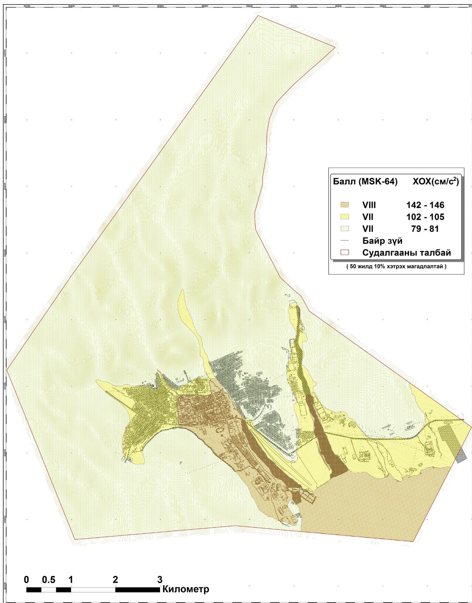
Зураг 13 Архангай аймгийн төв Эрдэнэбулган сумын газар хөдлөлийн мужлал. (500 жил)
