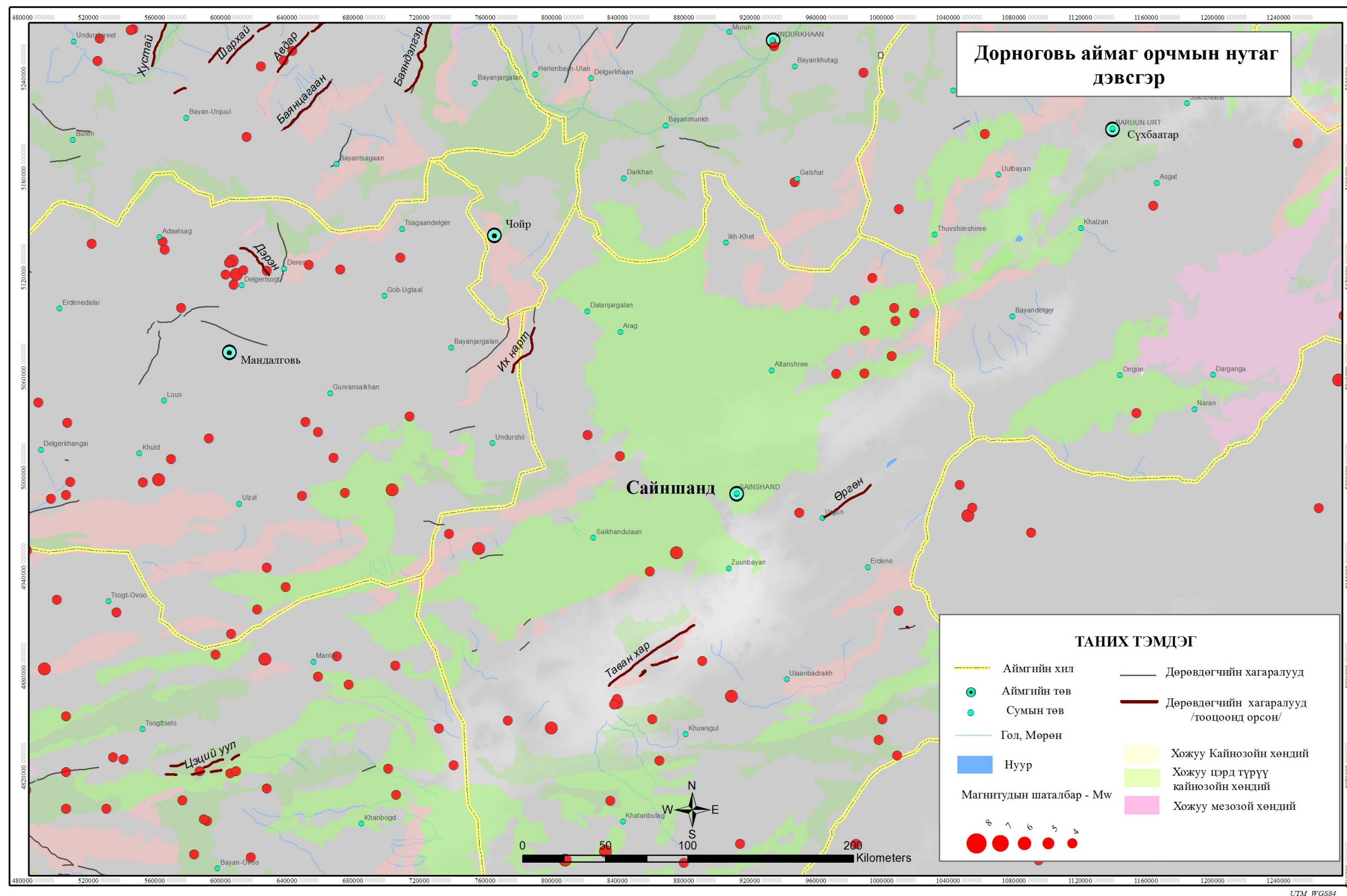
Зураг 51 Дорноговь аймгийн төв Сайншанд сумын сейсмотектоникийн тойм зураг
