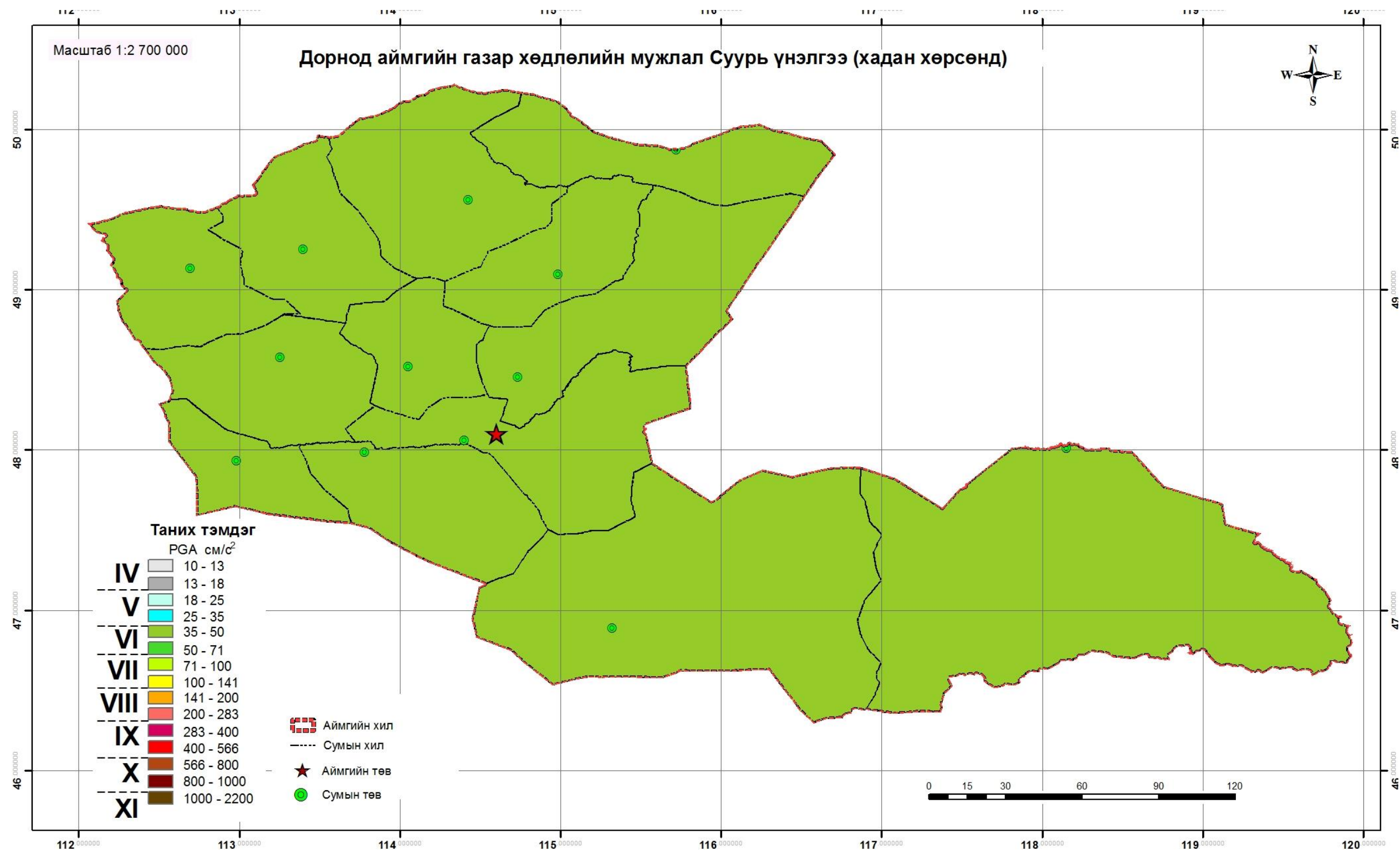
Зураг 132 Дорнод аймгийн төв Хэрлэн сумын газар хөдлөлийн мужлал – Суурь үнэлгээ (хадан хөрсөнд)
