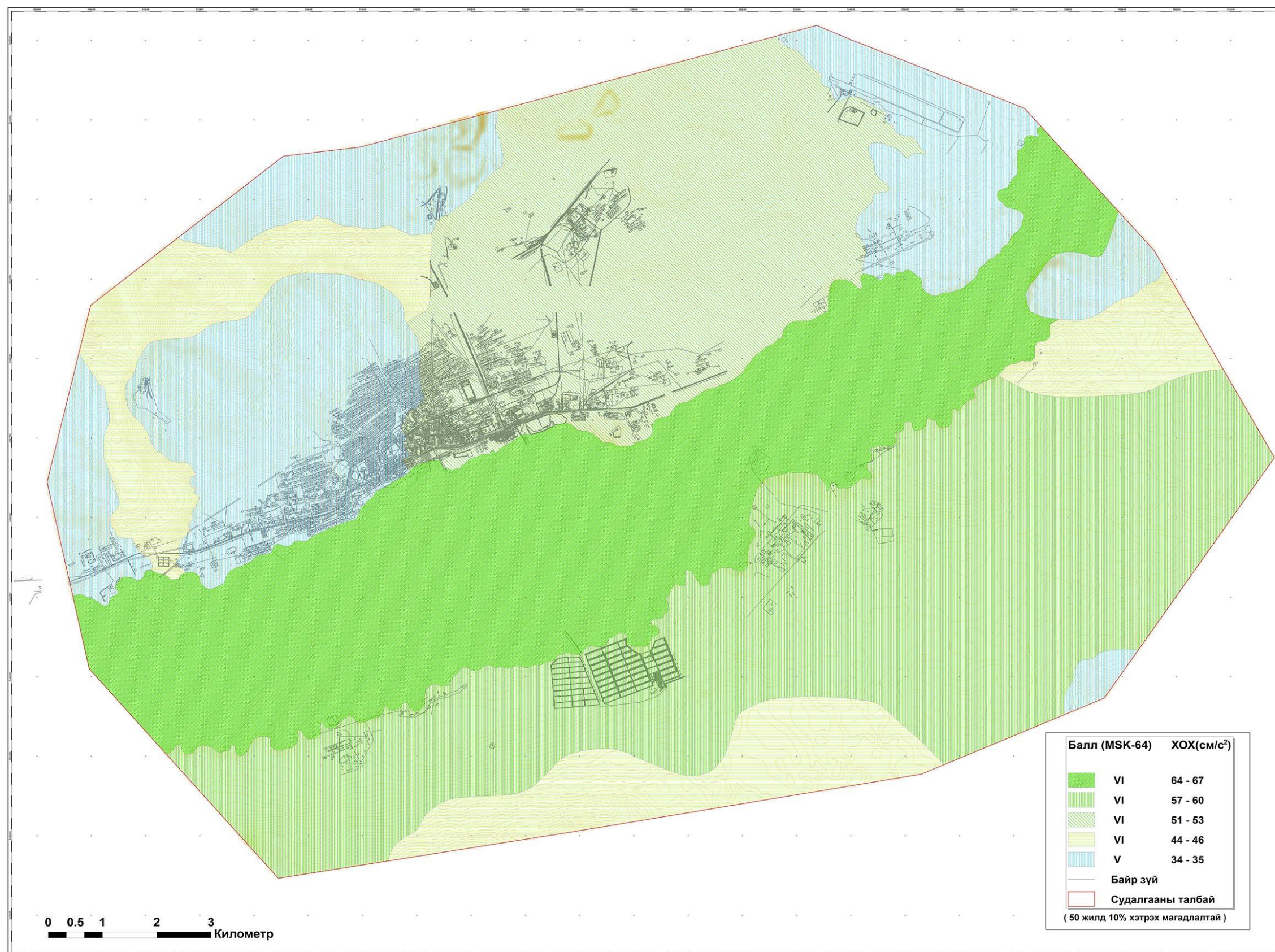
Зураг 134 Дорнод аймгийн төв Хэрлэн сумын газар хөдлөлийн бичил мужлалын зураг (500 жил )
