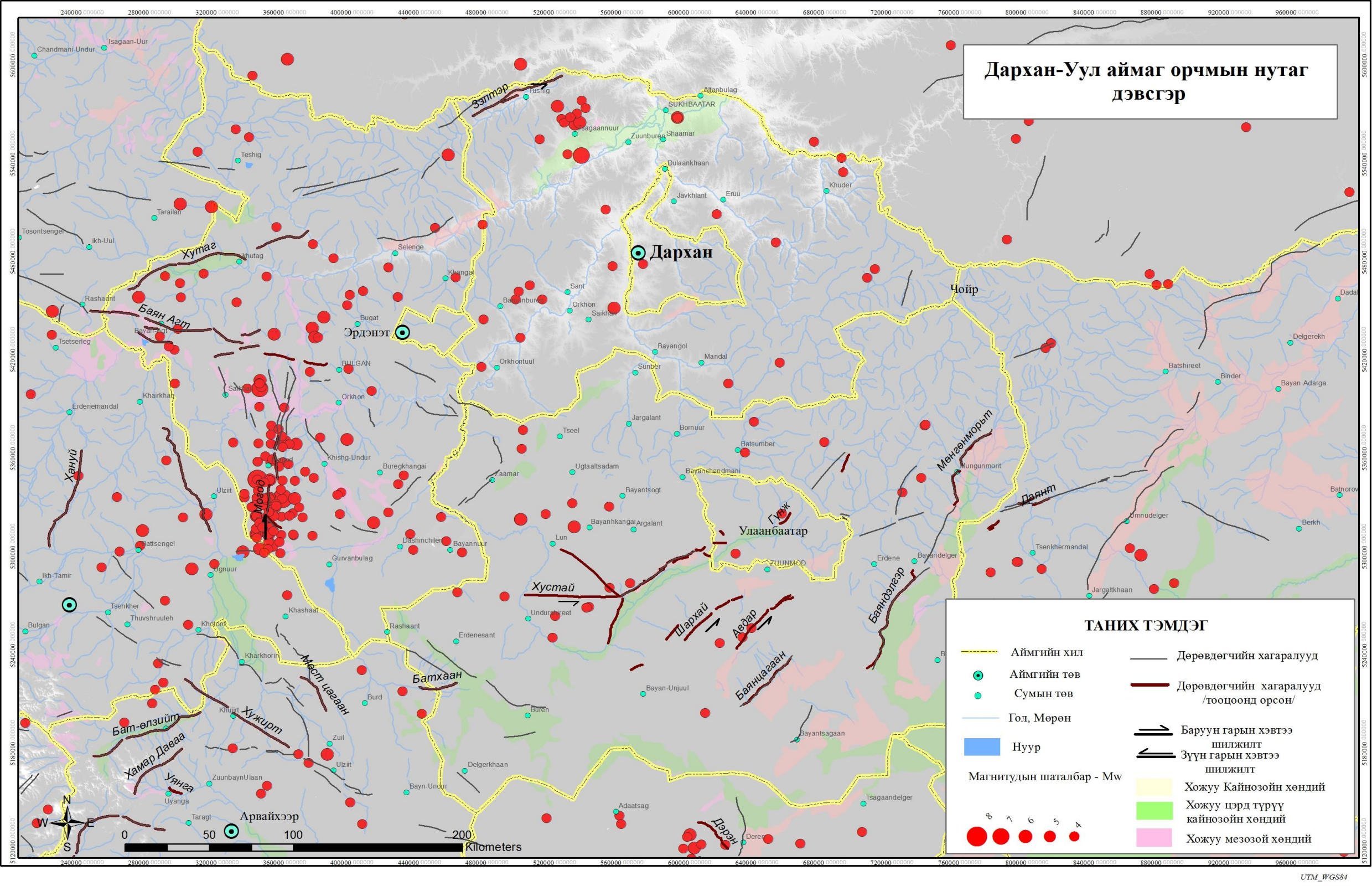
Зураг 40 Дархан- Уул аймаг орчмын Дархан сумын сейсмотектоникийн тойм зураг
