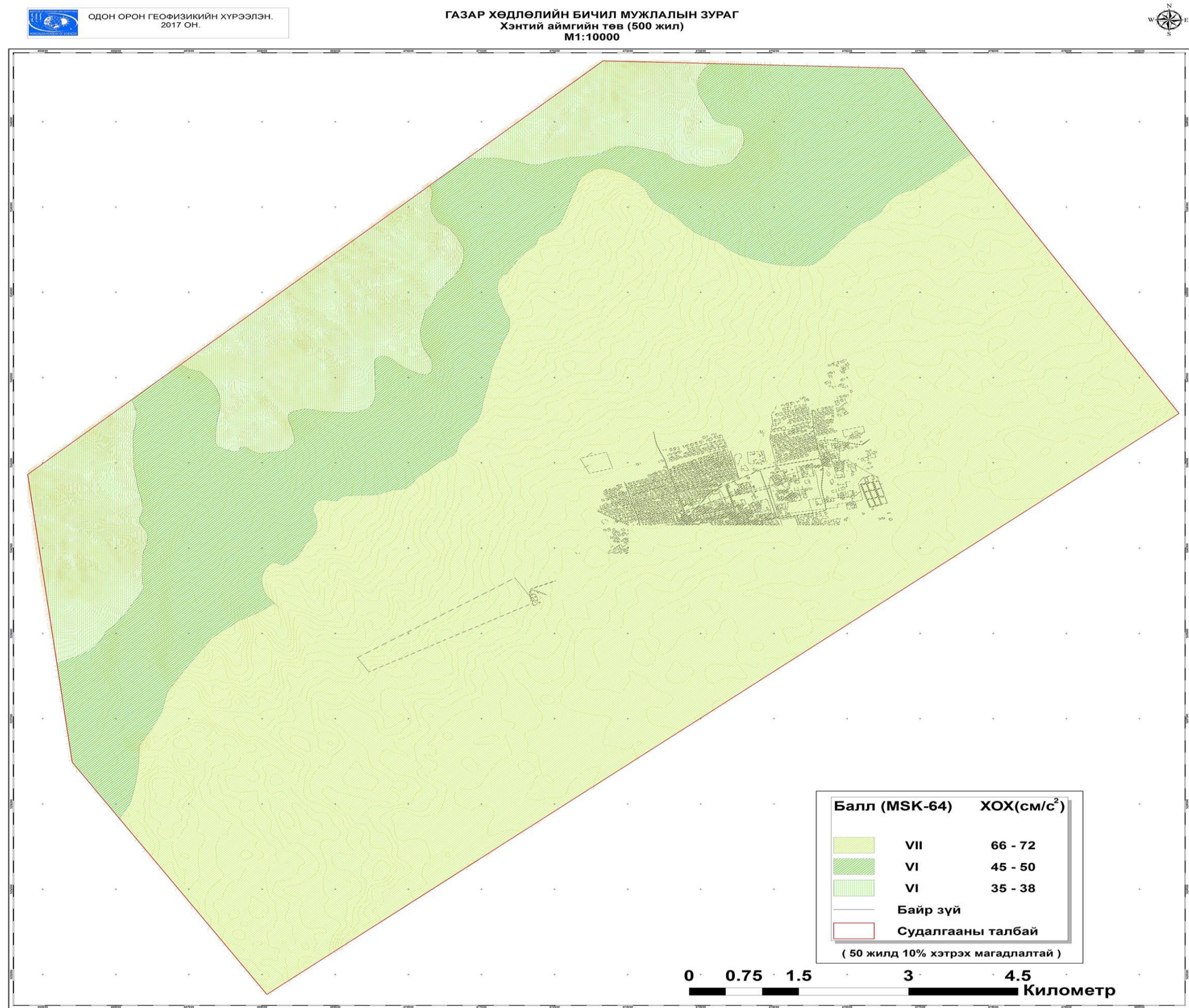
Зураг 101 Хэнтий аймгийн төв Хэрлэн сумын газар хөдлөлийн бичил мужлалын зураг (500 жил )
