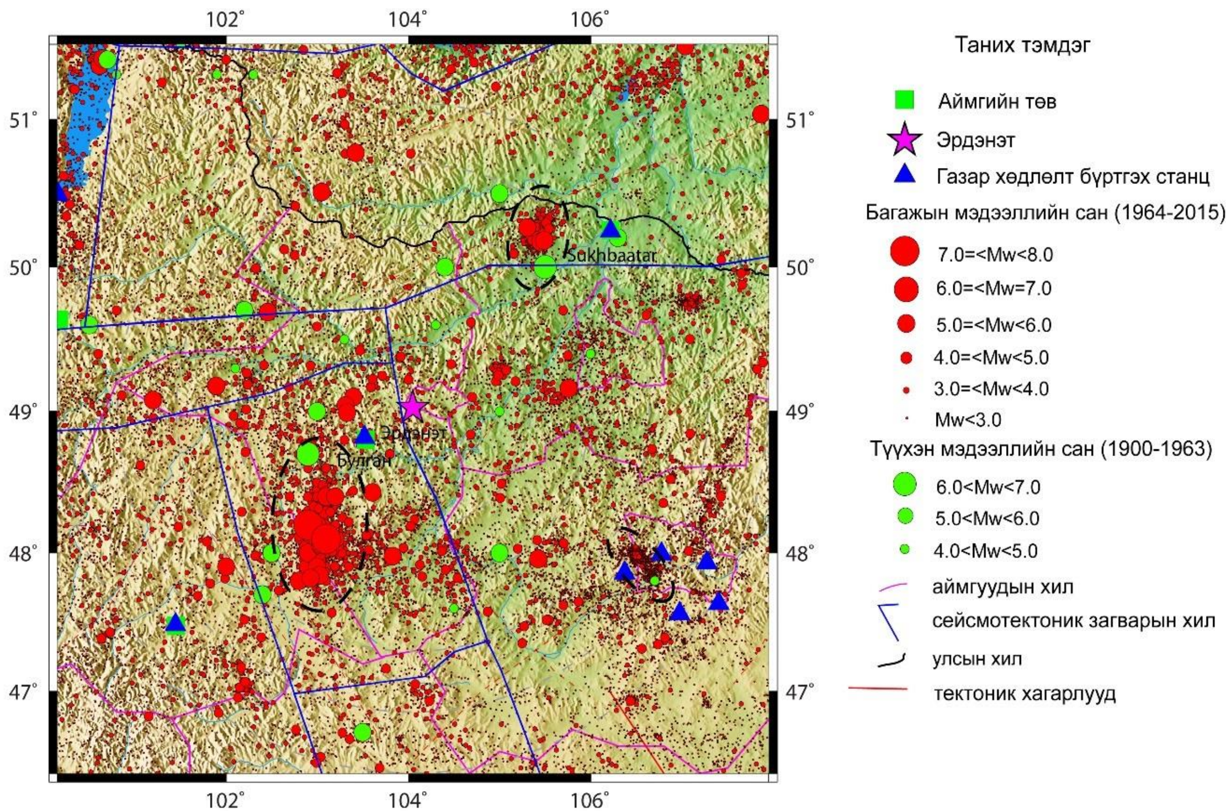
Зураг 85 Орхон аймаг орчмын газар хөдлөлтийн идэвхжилт
