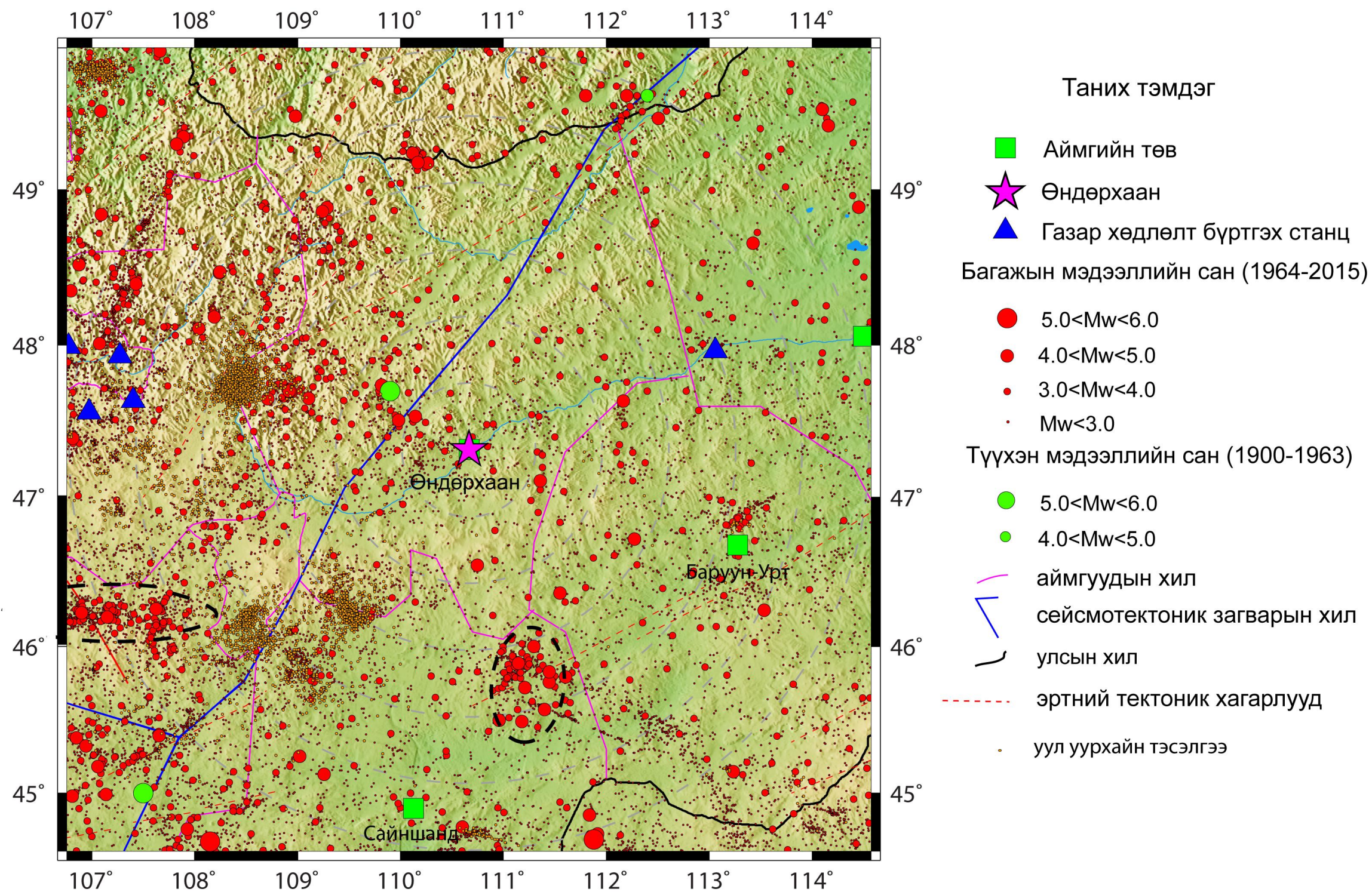
Зураг 96 Хэнтий аймаг орчмын газар хөдлөлийн идэвхжилт.
