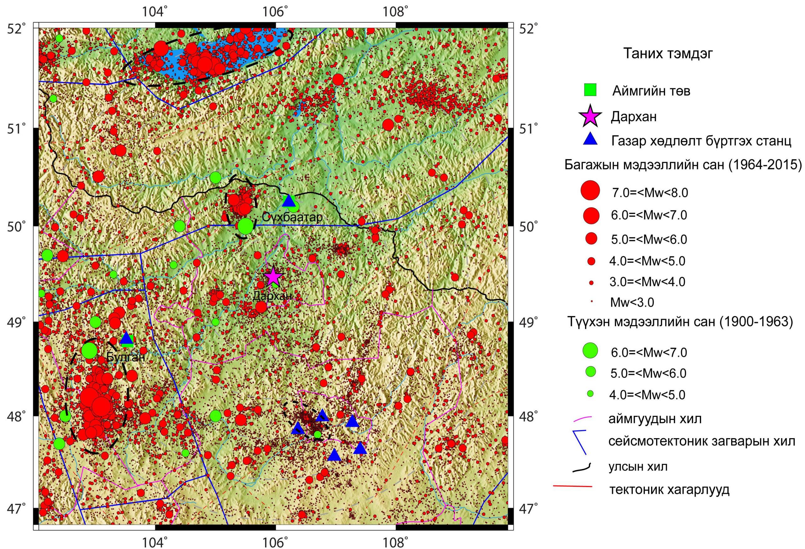
Зураг 41 Дархан- Уул аймгийн төв Дархан сумын газар хөдлөлийн идэвхжилт.
