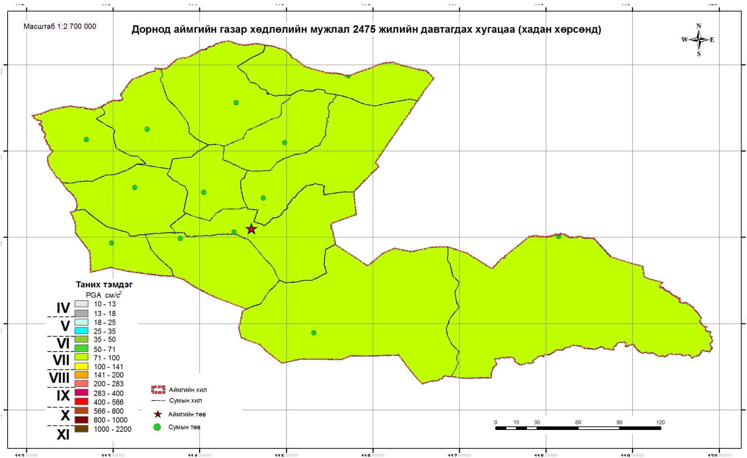
Зураг 131 Дорнод аймгийн төв Хэрлэн сумын газар хөдлөлийн мужлал (2475 жилийн давтагдах хугацаа- хадан хөрсөнд)
