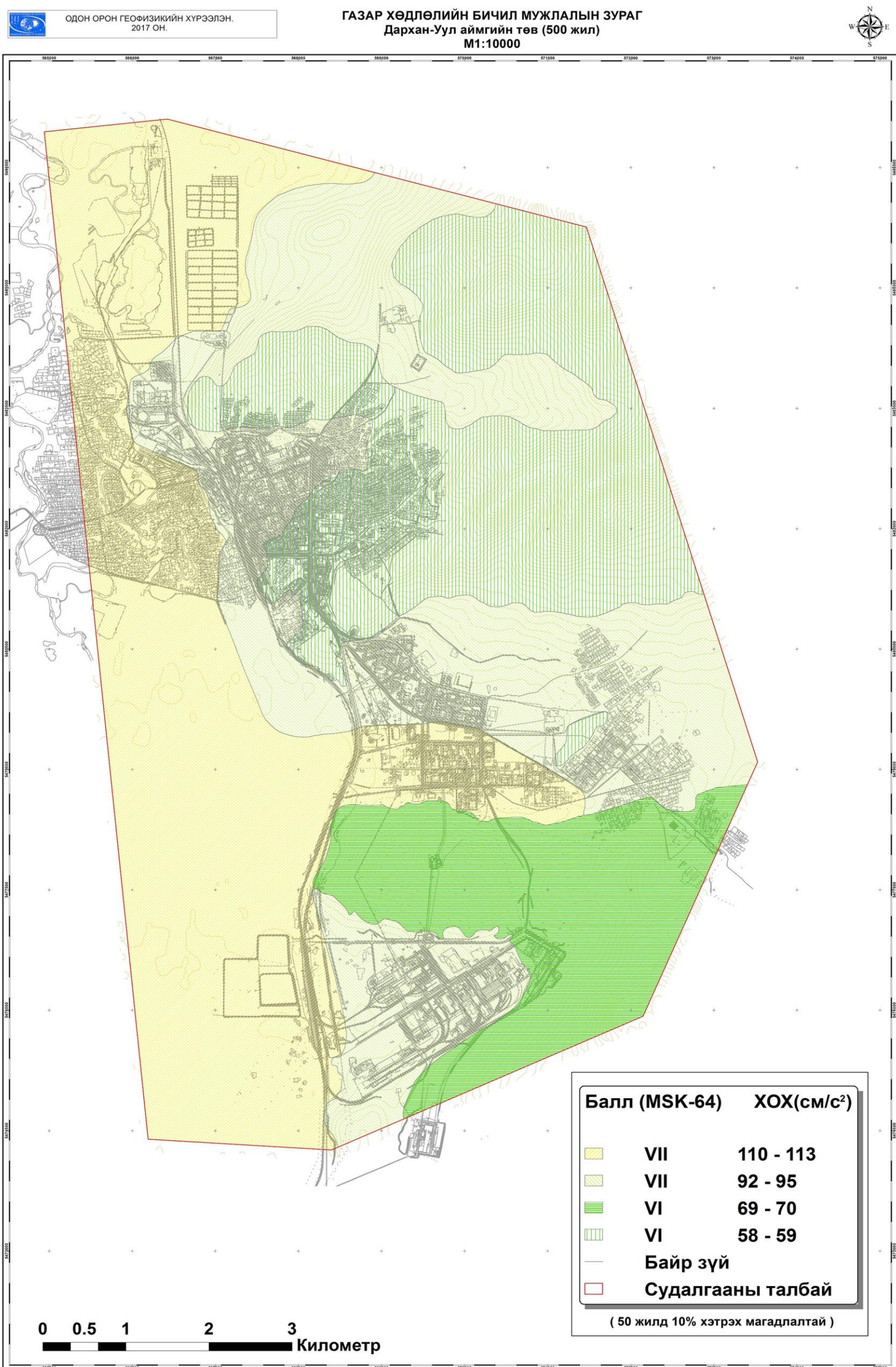
Зураг 46 Дархан- Уул аймгийн төв Дархан сумын газар хөдлөлийн бичил мужлал (500 жил )
