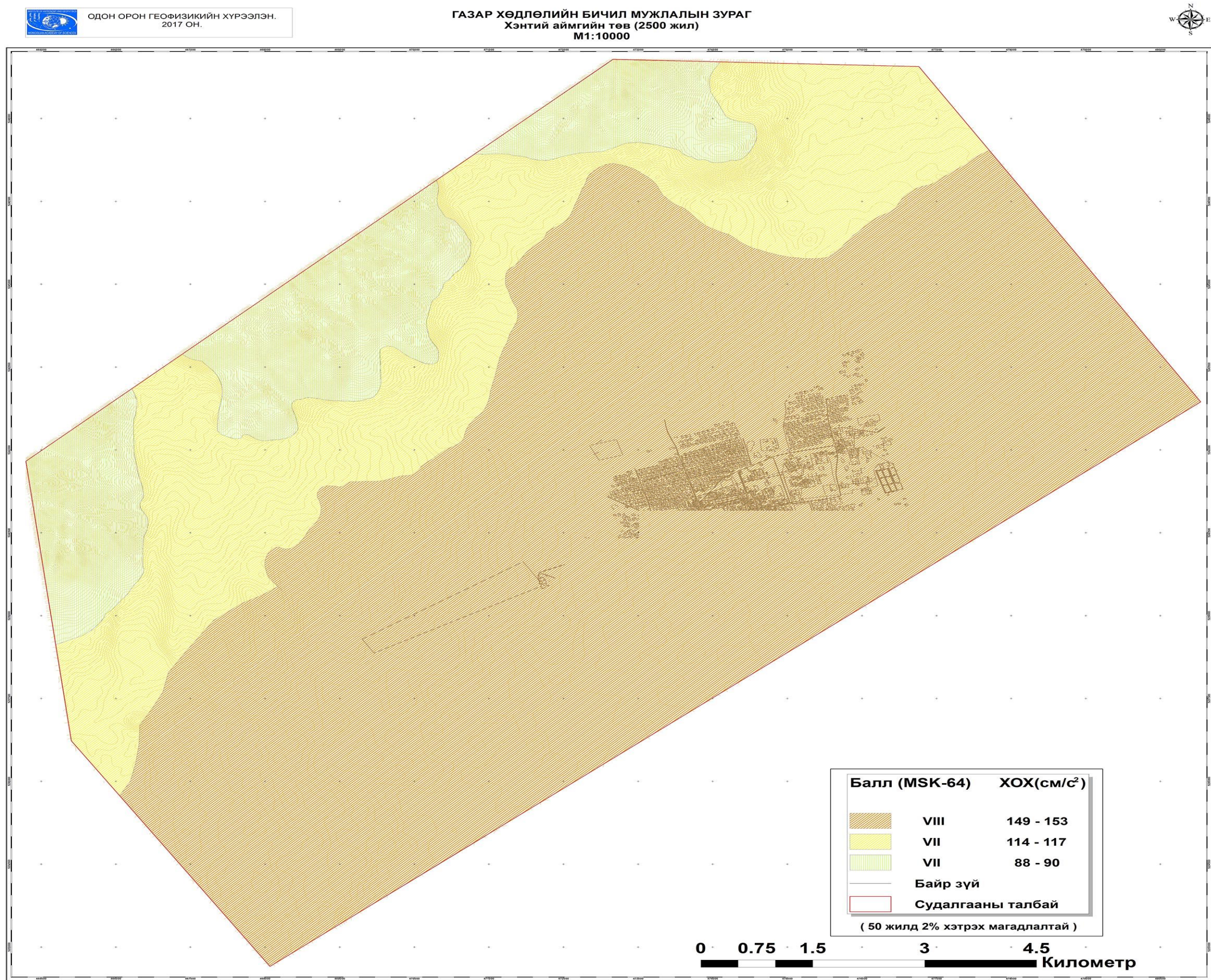
Зураг 102 Хэнтий аймгийн төв Хэрлэн сумын газар хөдлөлийн бичил мужлалын зураг (2500 - жил )
