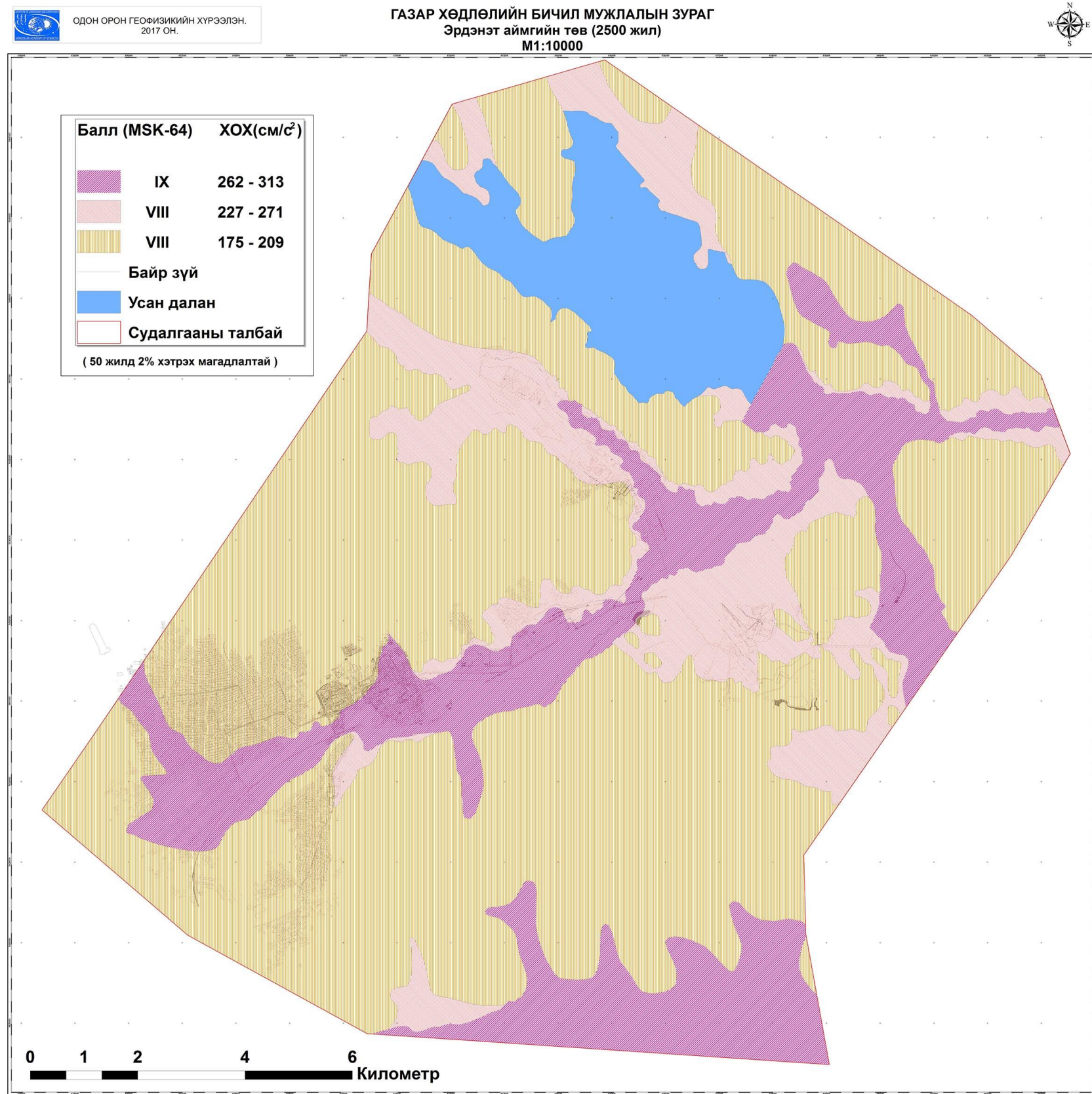
Зураг 91 Орхон аймгийн төв Баян- Өндөр сумын газар хөдлөлийн бичил мужлалын зураг (2500 жил )
