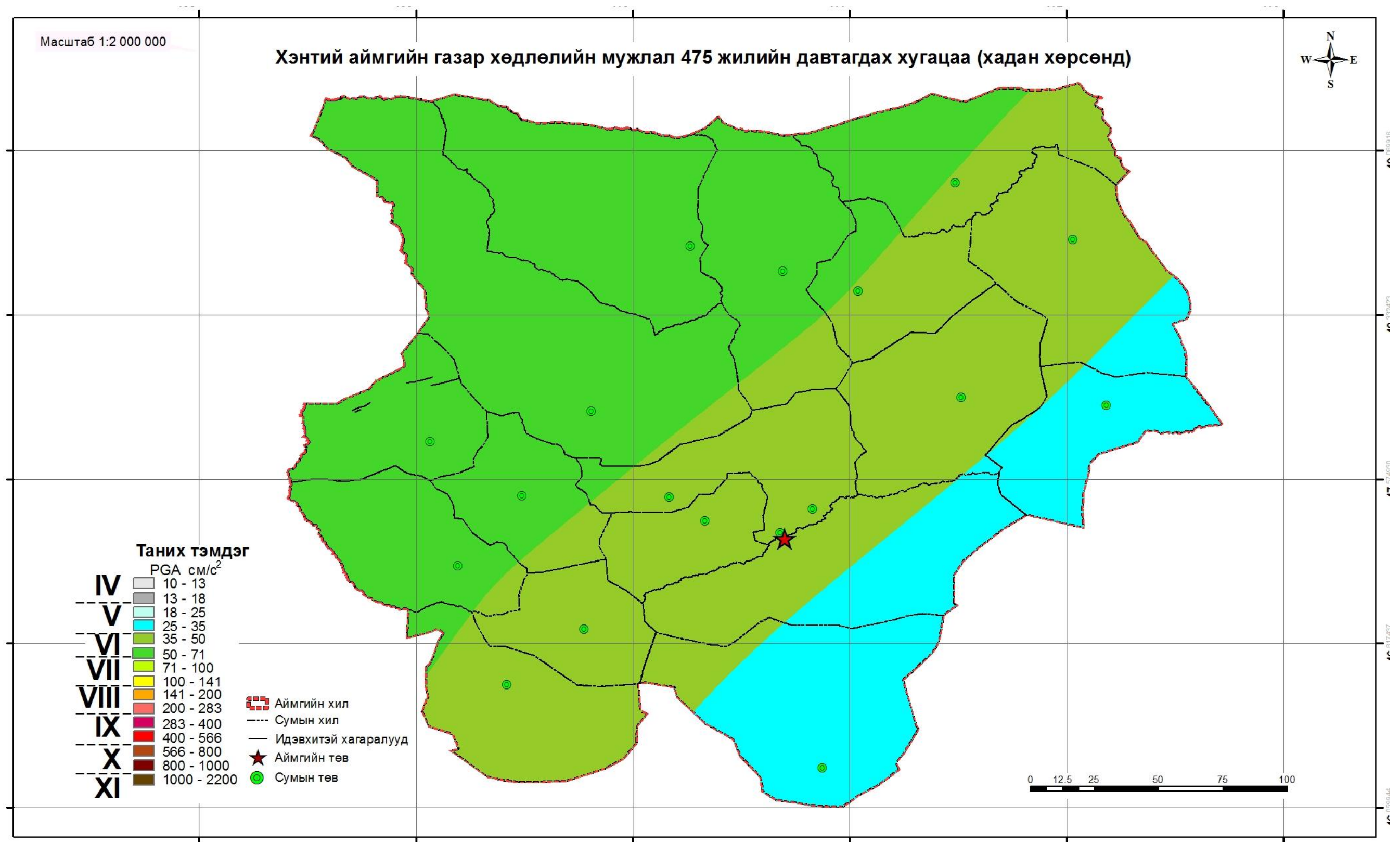
Зураг 97 Хэнтий аймгийн төв Хэрлэн сумын газар хөдлөлийн мужлал (475 жилийн давтагдах хугацаа- хадан хөрсөнд)
