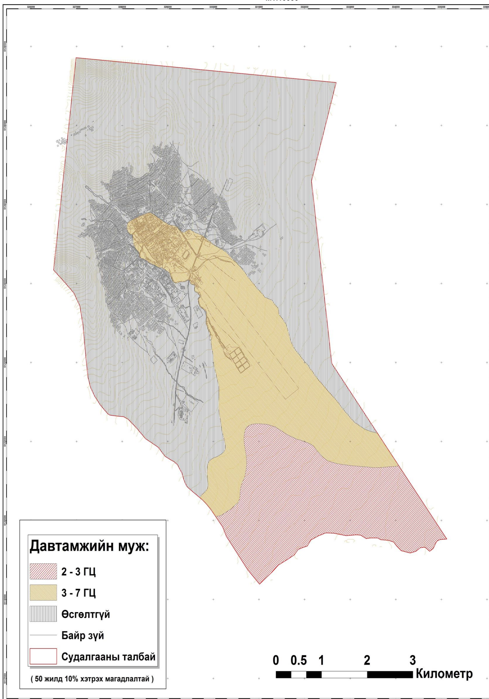
Зураг 122 Өвөрхангай аймгийн төв Арвайхээр сумын хөрсний зонхилох давтамжийн мужлал.
