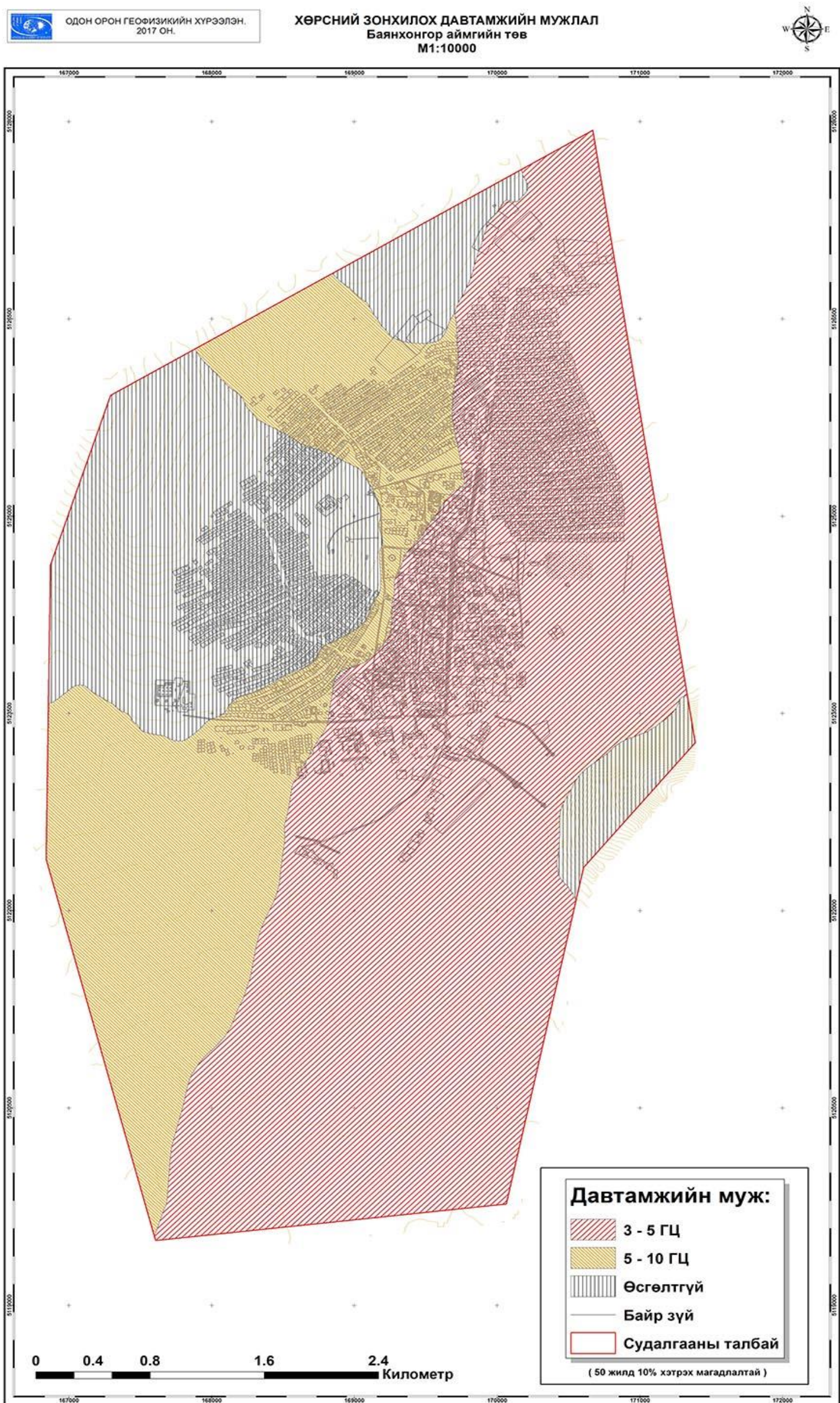
Зураг 23 Баянхонгор аймгийн Баянхонгор сумын хөрсний зонхилох давтамжийн мужлал
