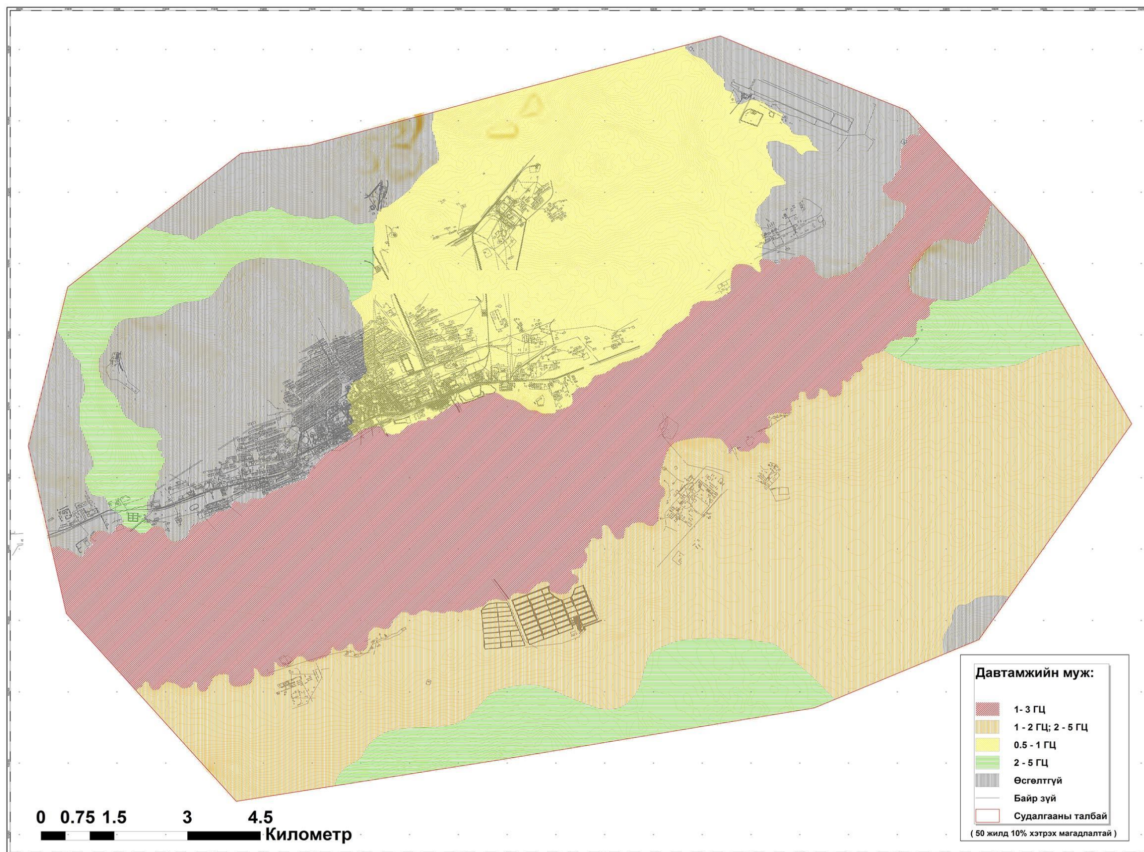
Зураг 133 Дорнод аймгийн төв Хэрлэн сумын хөрсний зонхилох давтамжийн мужлал
