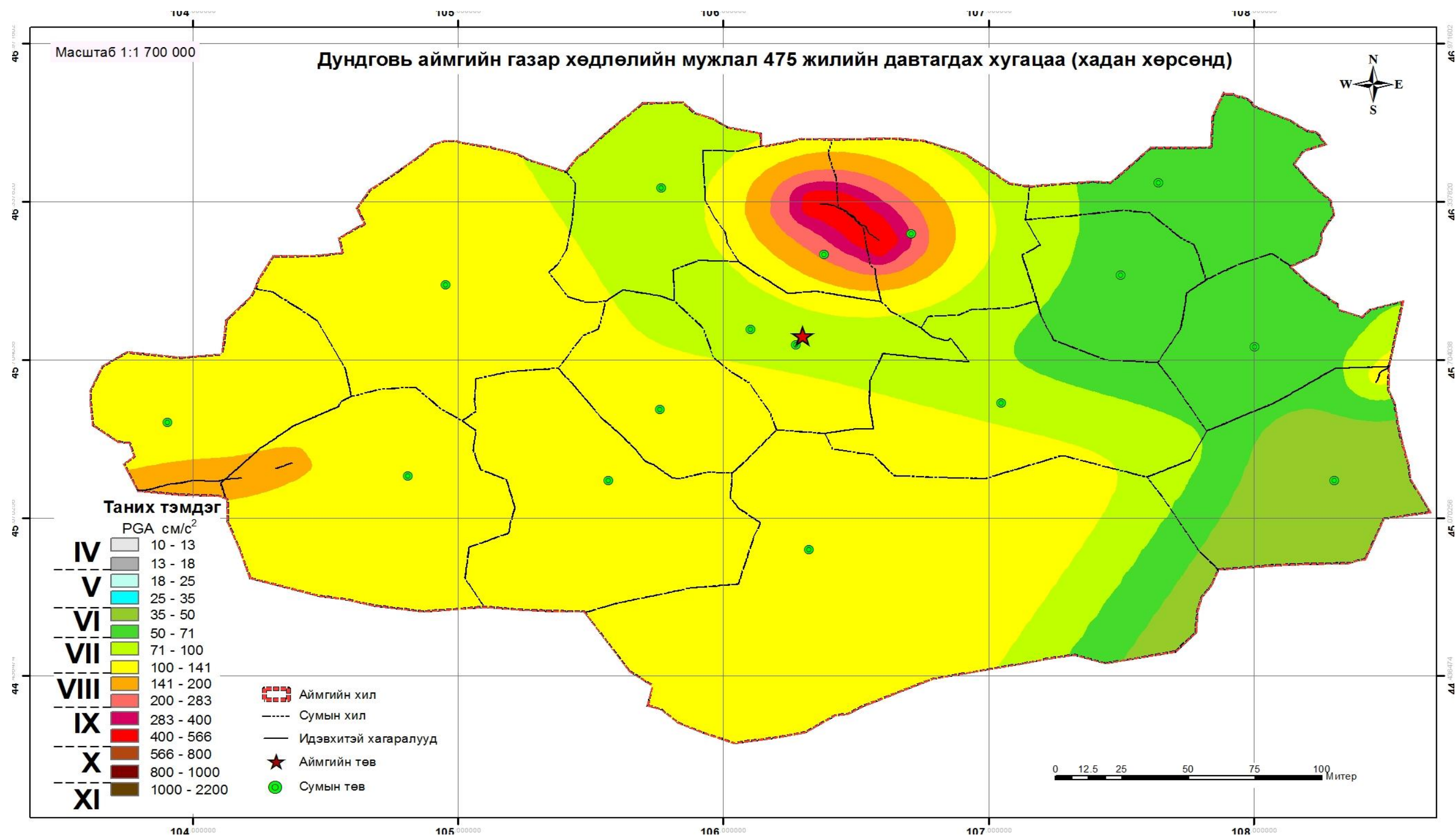
Зураг 64 Дундговь аймгийн төв Сайнцагаан сумын газар хөдлөлийн мужлал (475 жилийн давтагдах хугацаа- хадан хөрсөнд)
