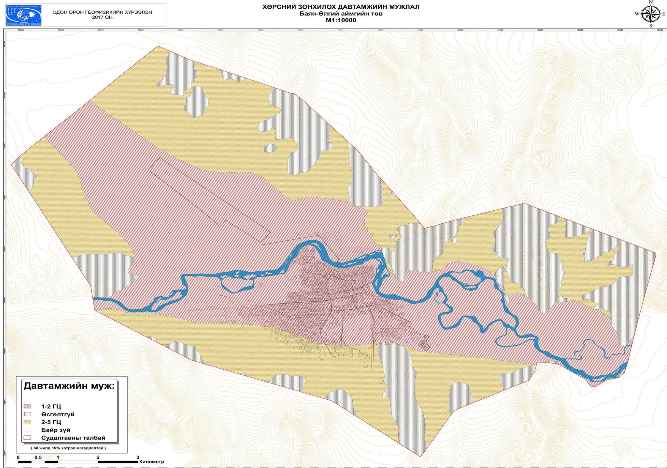
Зураг 34 Баян- өлгий аймгийн төв Өлгий сумын хөрсний зонхилох давтамжийн мужлал
