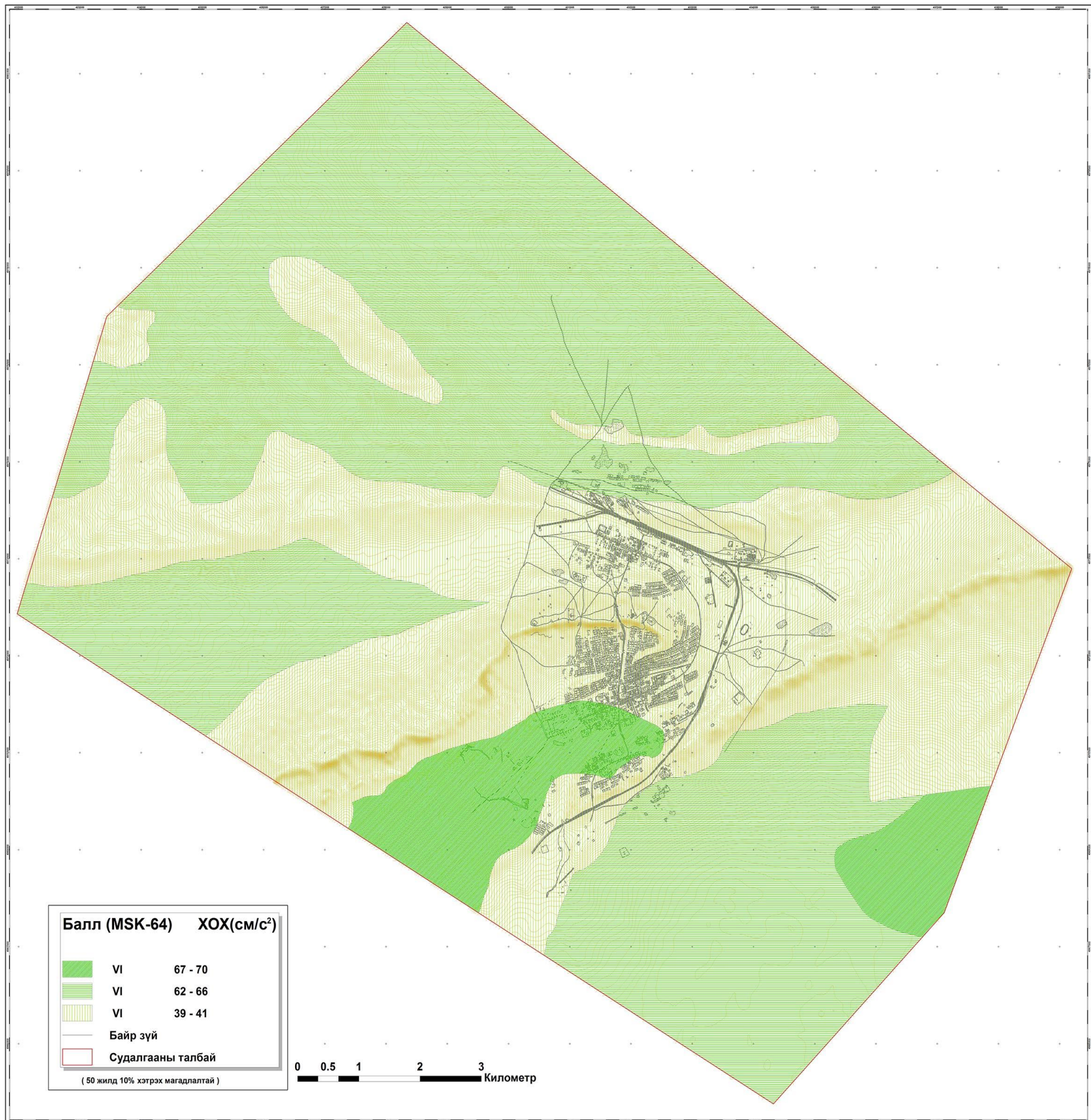
Зураг 57 Дорноговь аймгийн төв Сайншанд сумын газар хөдлөлийн бичил мужлалын зураг (500 жил )
