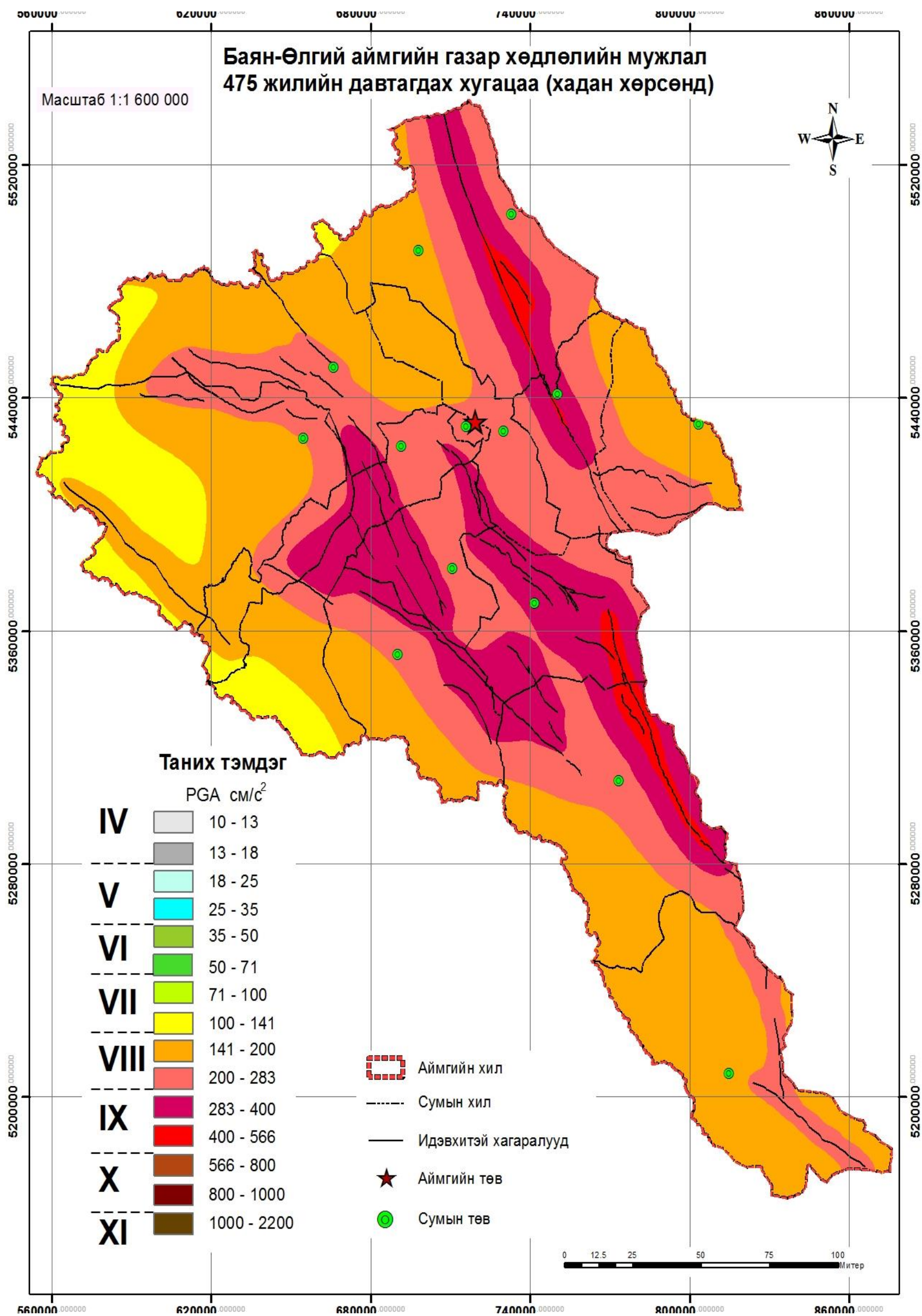
Зураг 31 Баян- өлгий аймгийн төв Өлгий сумын газар хөдлөлийн мужлал (475 жилийн давтагдах хугацаа- хадан хөрсөнд)
