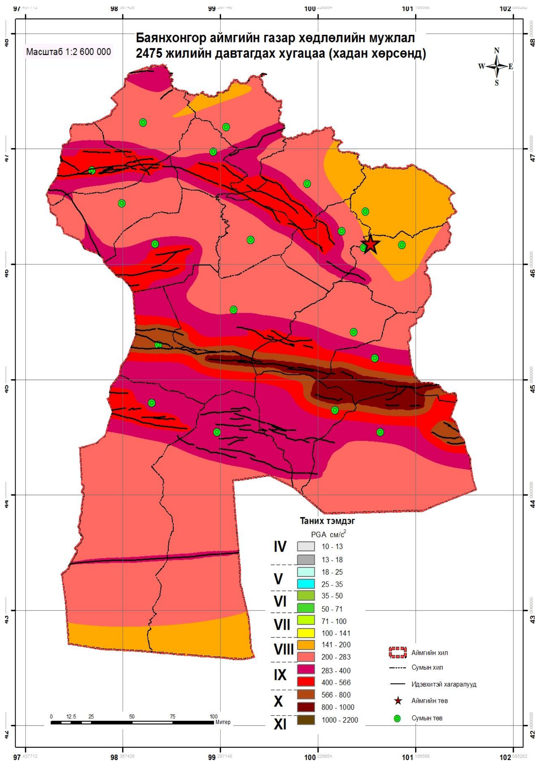
Зураг 21 Баянхонгор аймгийн Баянхонгор сумын газар хөдлөлийн мужлал (2475 жилийн давтагдах хугацаа хадан хөрсөнд)
