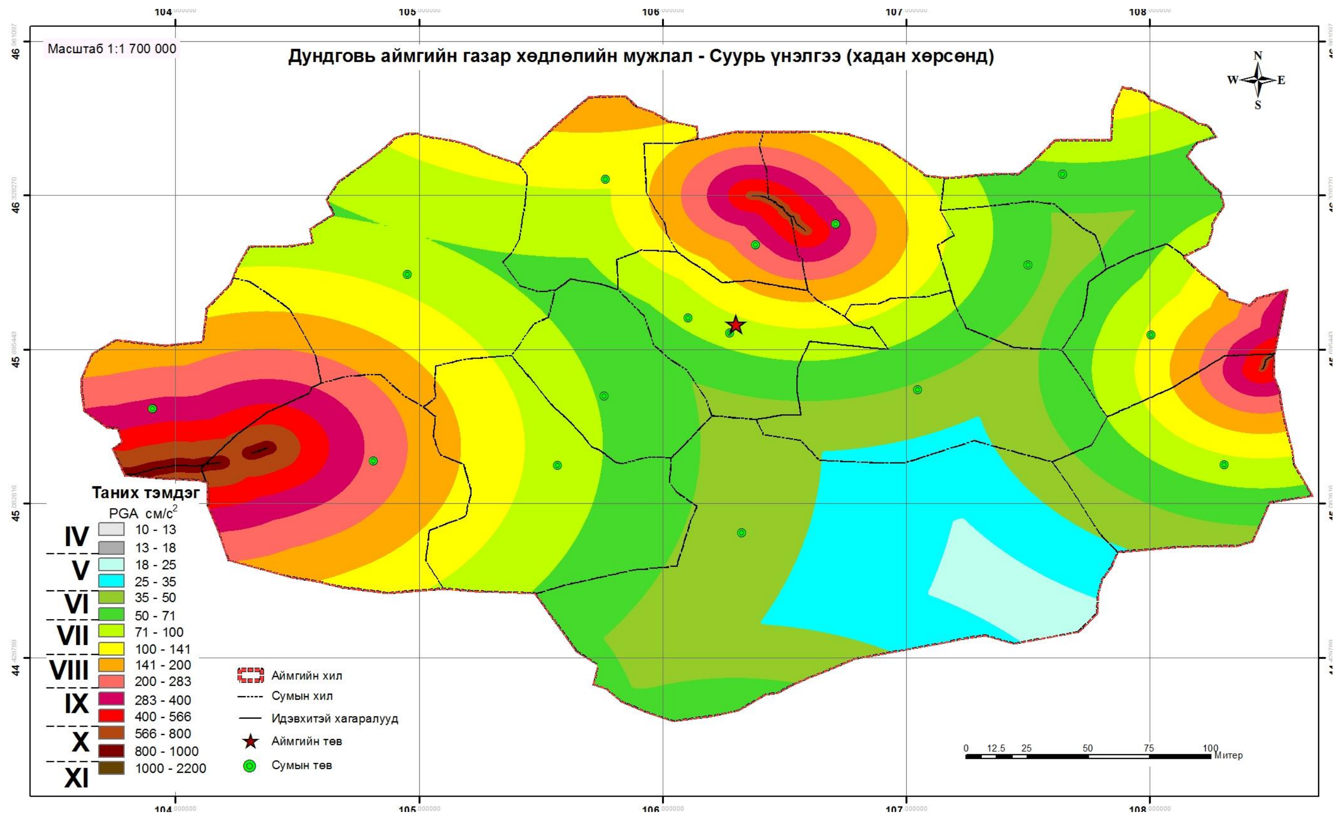
Зураг 66 Дундговь аймгийн төв Сайнцагаан сумын газар хөдлөлийн мужлал – Суурь үнэлгээ (хадан хөрсөнд)
