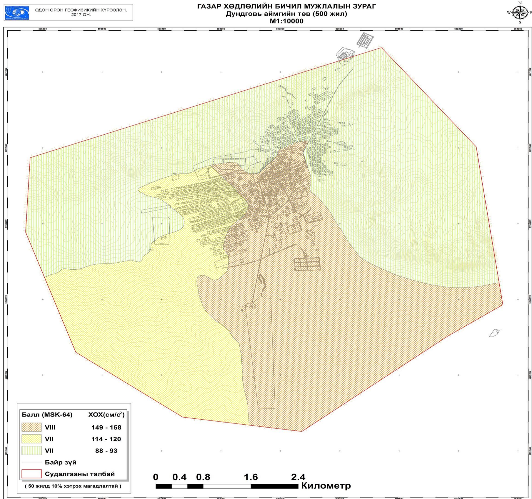
Зураг 68 Дундговь аймгийн төв Сайнцагаан сумын газар хөдлөлийн бичил мужлал (500 жил )
