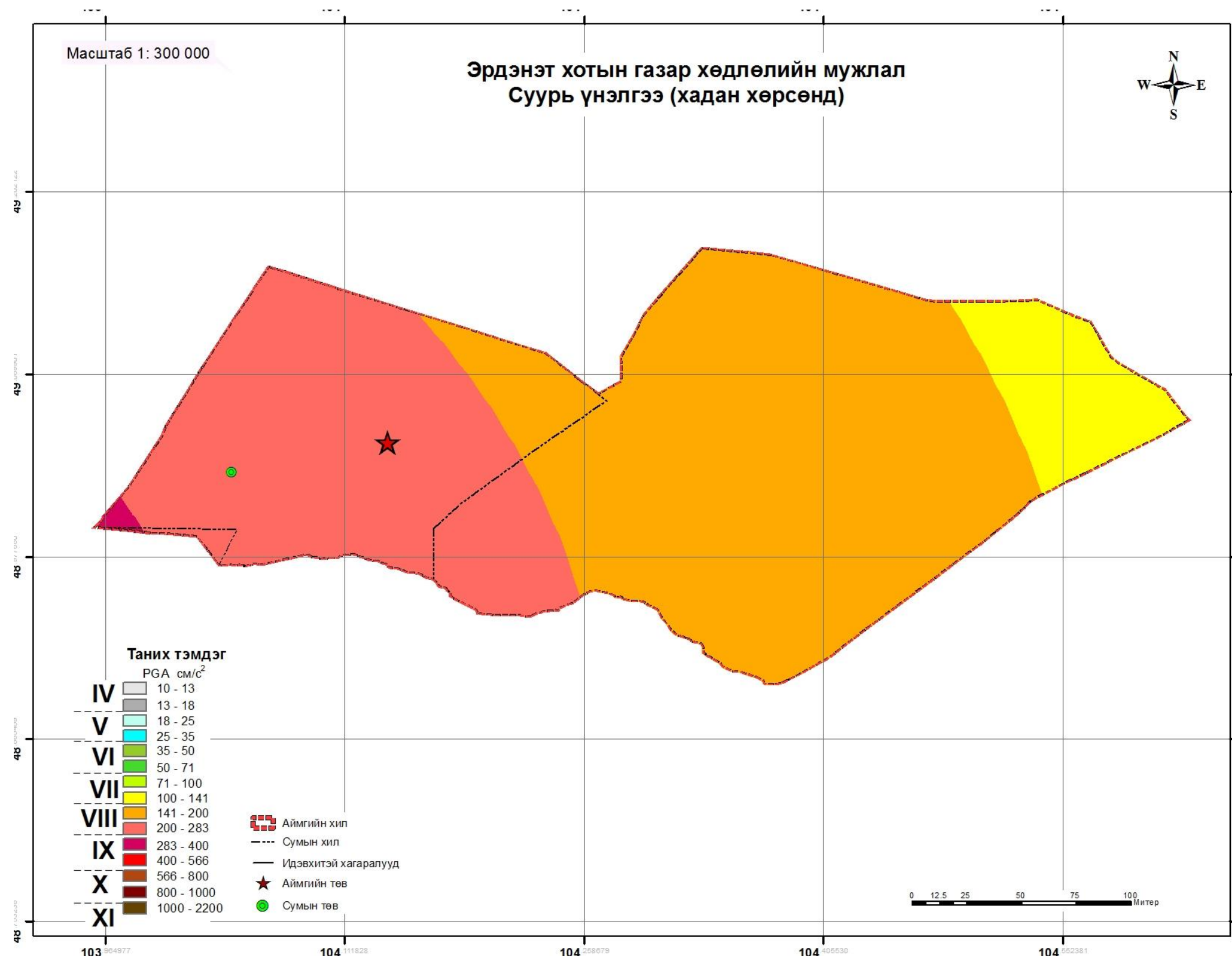
Зураг 88 Орхон аймгийн төв Баян- Өндөр сумын газар хөдлөлийн мужлал – Суурь үнэлгээ (хадан хөрсөнд)
