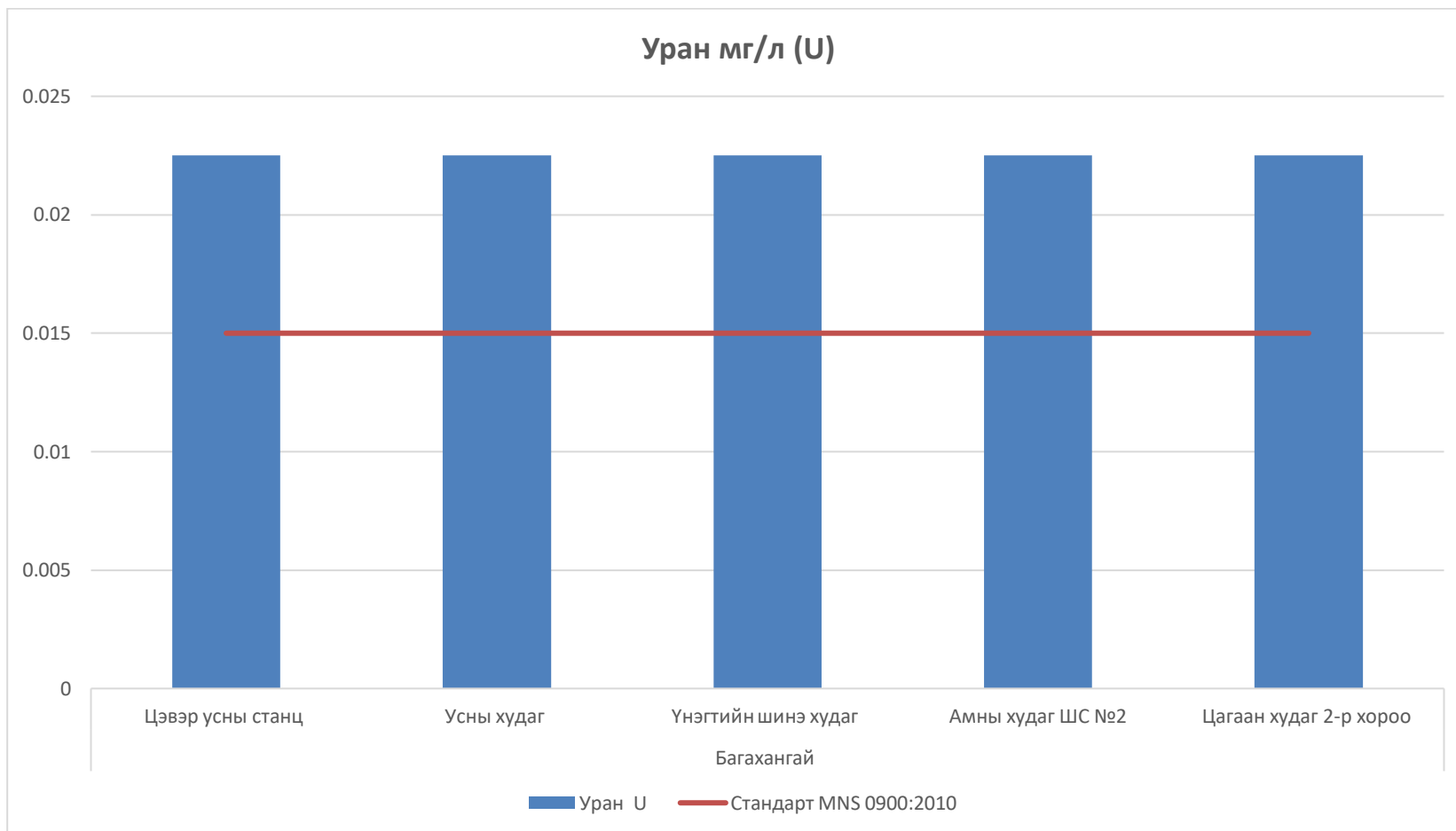
График 2 Ураны агуулга, мг/л
