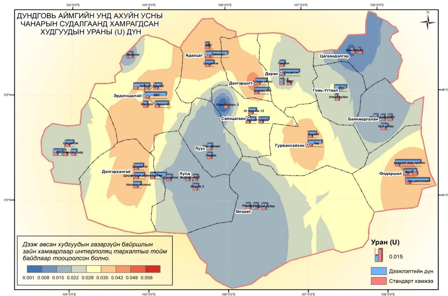
Зураг 2 Дээж авсан худгуудын газарзүйн байршлын Ураны тархалтын тойм зураг
