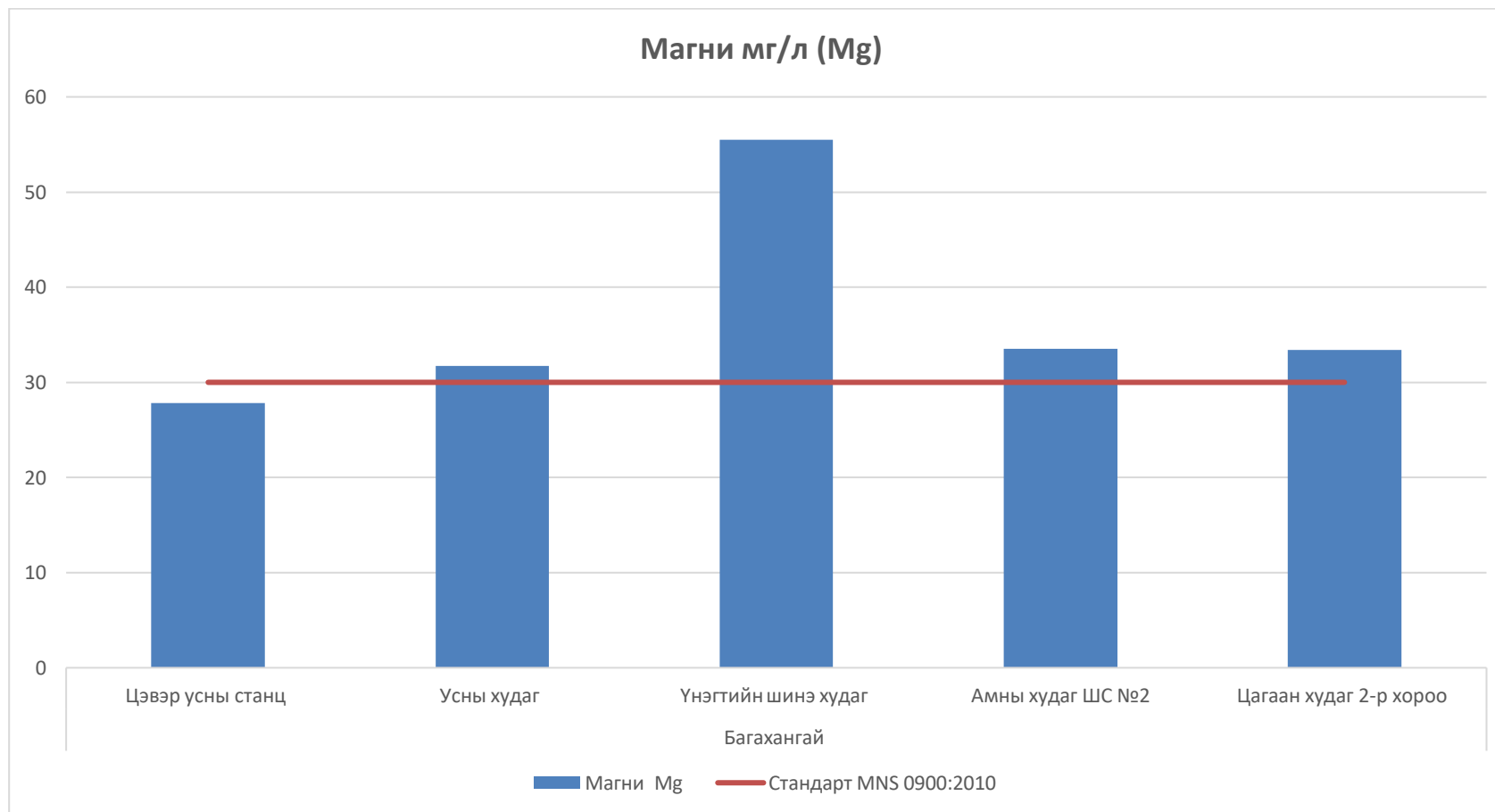
График 1 Магнийн агуулга, мг/л
