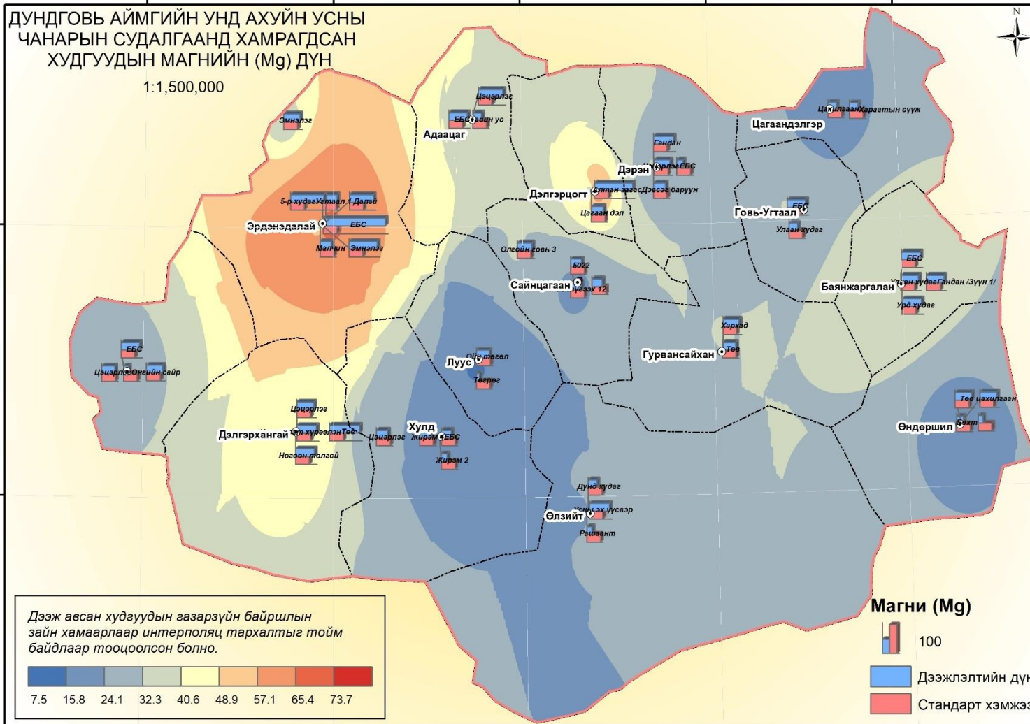
Зураг 1 Дээж авсан хуудгуудын газарзүйн байршлын Магни тархалтын тойм зураг
