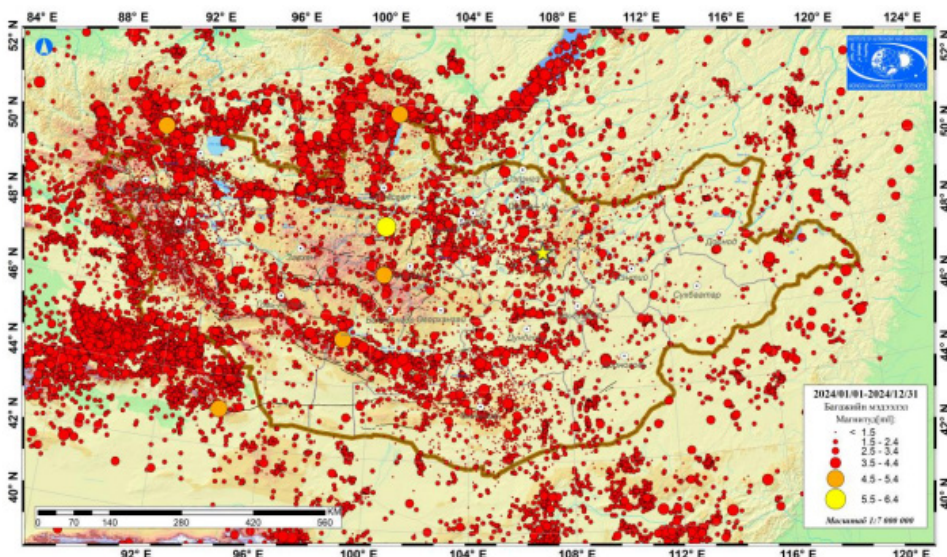
Зураг 82. Газар хөдлөлтийн тархалтын зураг 2024 он
