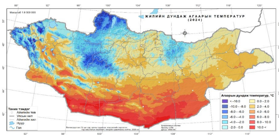
Зураг 89. 2024 оны жилийн дундаж агаарын температурын орон зайн тархалт
