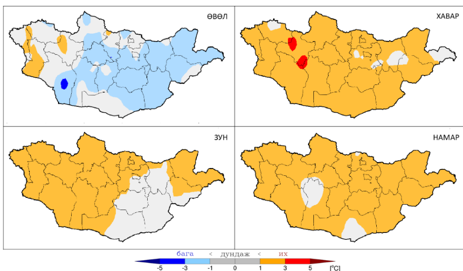
Зураг 90. 2024 оны улирлын агаарын дундаж температурын ОЖД-аас (норм 1991-2020 он) хазайх хазайлт
