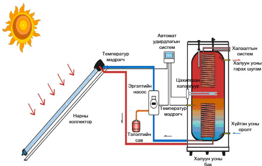
Зураг 35: нарны вакуум коллектор систем
