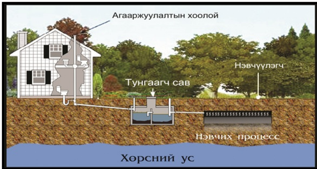
Зураг 41: Тунгаагчтай септик системийн ерөнхий бүдүүвч
