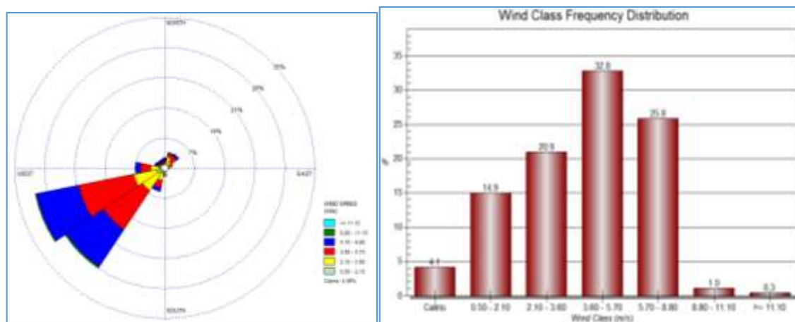
Зураг 3.5. Салхины горим, Өндөрхаан нисэх буудлын уурын автомат станцын мэдээ
