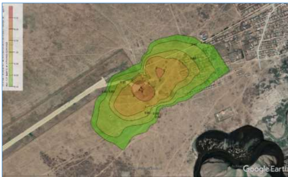
Зураг 3.6. Халаалтын зуухнаас хаягдах хүхэрлэг хийн тархалт, /24 цагийн дундаж/
