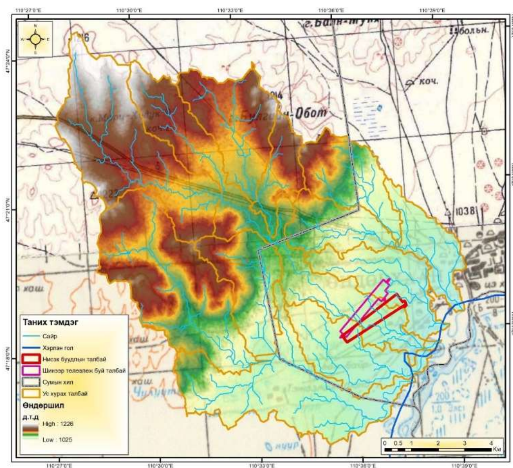
Зураг 3.11. Аэродром дайран өнгөрөх жижиг сайруудын ус хураах
