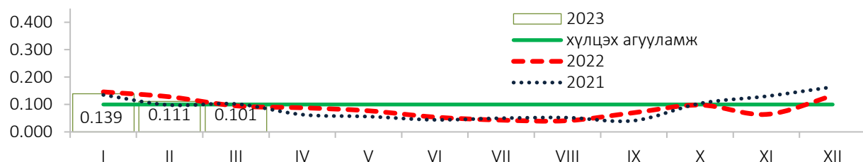
ЗУРАГ 6. УЛААНБААТАР 3 ХОТЫН АГААР ДАХЬ 10 МИКРОНООС БАГА ХЭМЖЭЭТЭЙ ТООСНЫ АГУУЛАМЖ, 15 СТАНЦЫН ДУНДАЖ, МГ/М 3
