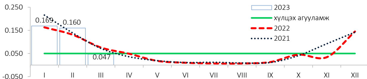
ЗУРАГ 5. УЛААНБААТАР 3 ХОТЫН АГААР ДАХЬ АЗОТЫН ДАВХАР ИСЛИЙН АГУУЛАМЖ, 10 СТАНЦЫН ДУНДАЖ, МГ/М 3
