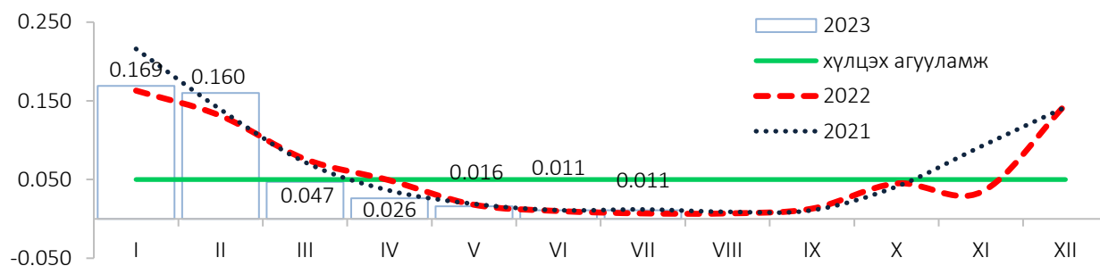
ЗУРАГ 4. УЛААНБААТАР 3 ХОТЫН АГААР ДАХЬ ХҮХЭРЛЭГ ХИЙН АГУУЛАМЖ, 13 СТАНЦЫН ДУНДАЖ, МГ/М 3
