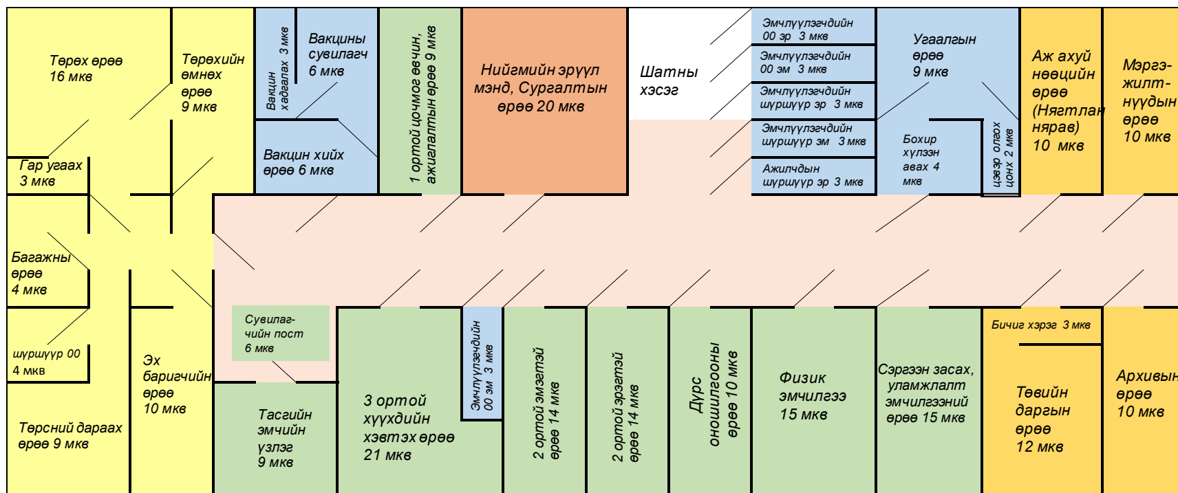
Зураг 7. Булган аймгийн Дашинчилэн СЭМТ-ийн барилгын хоёрдугаар давхрын өрөөнүүдийн байршил, хэмжээ
