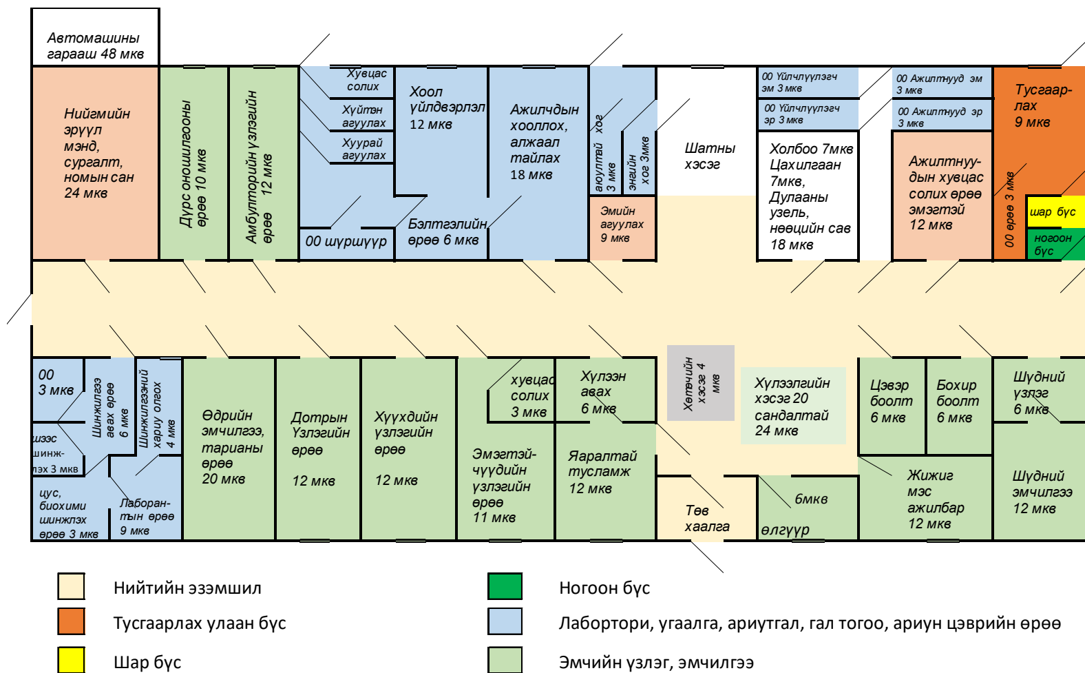
Зураг 9. Хөвсгөл аймгийн Тариалан СЭМТ-ийн барилгын нэгдүгээр давхрын өрөөнүүдийн байршил, хэмжээ
