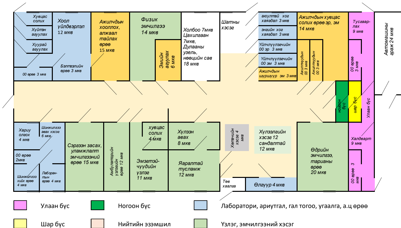
Зураг 4. Өвөрхангай аймгийн Баян-Өндөр СЭМТ-ийн барилгын нэгдүгээр давхрын өрөөнүүдийн байршил, хэмжээ
