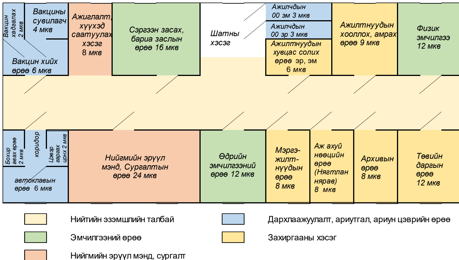
Зураг 2. Өрхийн эрүүл мэндийн төвийн нэг маягийн загварын барилгын хоярдугаар давхрын өрөөнүүдийн байршил, хэмжээ
