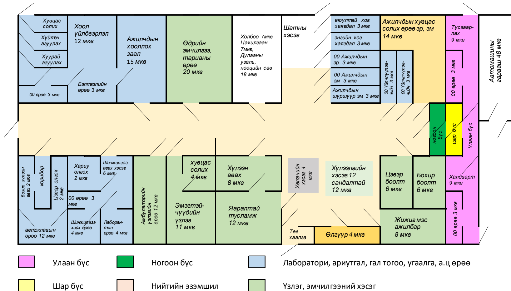
Зураг 6. Булган аймгийн Дашинчилэн СЭМТ-ийн барилгын нэгдүгээр давхрын өрөөнүүдийн байршил, хэмжээ
