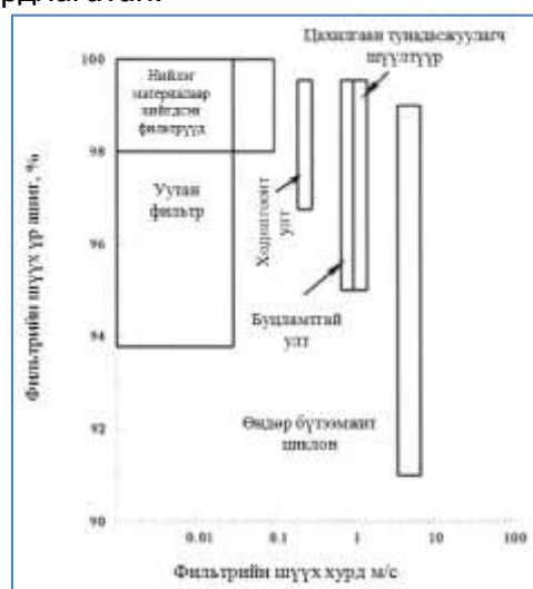
Зураг 4.1. Утаа шүүгч технологиуд ба тэдгээрийн үр ашиг
