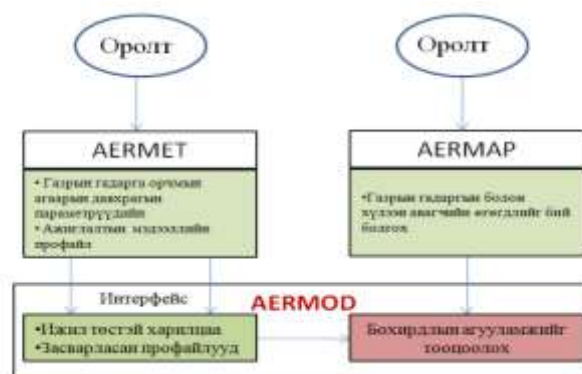
Зураг 3.3. AERMOD загварчлалын мэдээллийн урсгал
